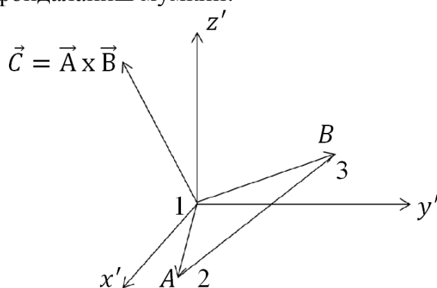
3.7-расм. Радиус-векторлар.
