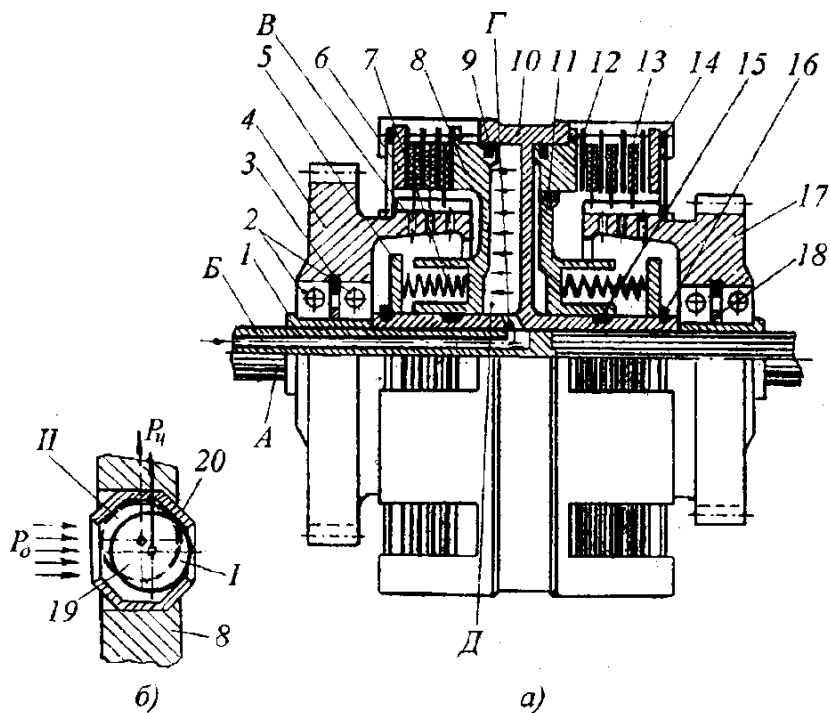
2-расм. Гидравлик тизимнинг суюклик босими билан ишлайдиган икки барабанли фрикцион муфта
