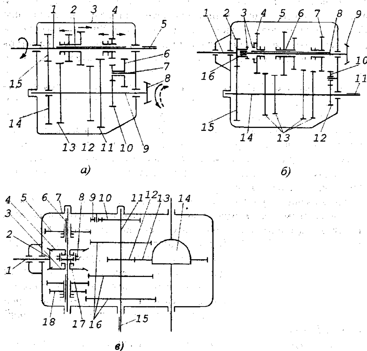
1-расм. Тракторларда қўлланадиган узатмалар қутиларини принципал кинематик схемалари
