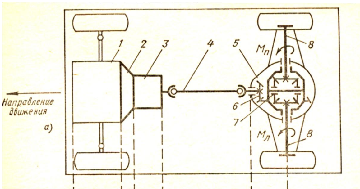
2-расм. Гилдирак схемаси 4x2 бўлган автомобил трансмиссияси схемаси 1-двигател; 2-тишлаши муфтаси; 3-узатмалар қутиси; 4-кардан узатмаси; 5-етакчи кўприк корпуси; 6-асосий ёки марказий узатма; 7-дифференциал; 8-ярим ўқлар
