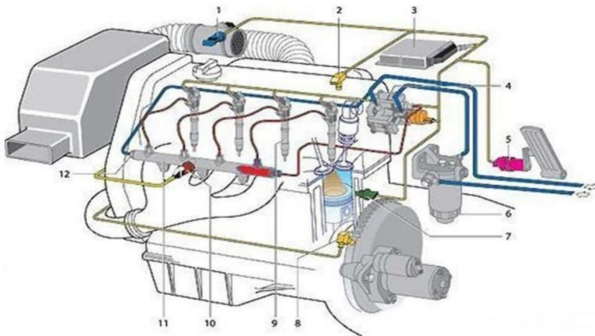
10-расм. Common Rail ёнилги узатиши тизими элементлари
