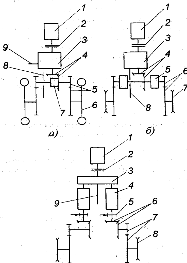
1-расм. Ғилдиракли ва занжирли тракторларнинг трансмиссиялари принципиал схемалари.
