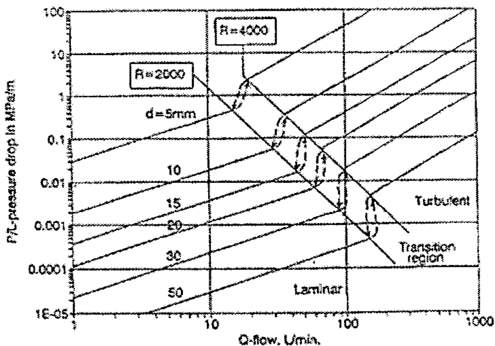
4-расм. Мой учун солиштирма массаси 0.85 ва динамик қовушқоқлиги 27,6 МПа S бўлган гидравлик блокларда босимнинг ўзгариши
