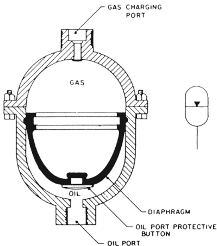
5-расм. Гидравлик аккумулятор
