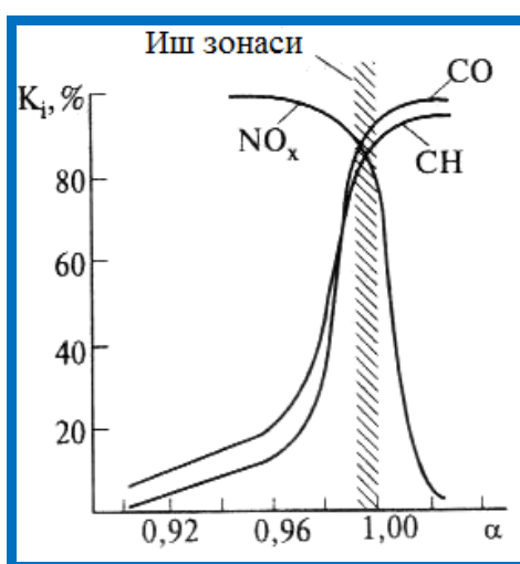
Уч компонентли нейтрализаторнинг эффектив ишлаш зонаси
