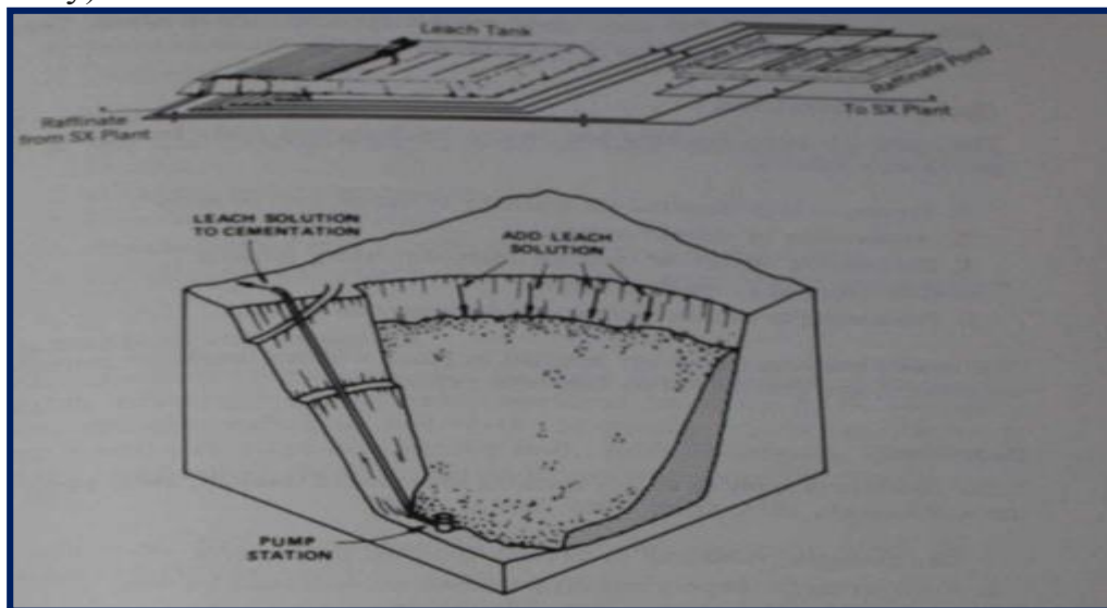
Рис. . Добыча руды путем выщелачивания (сверху) Кучного выщелачивания (после Schetlet, 1962(внизу) ) в-выщелачивании (после Кроуфорд и Hustrulid. 1979 году permiuton от общества горных инженеров. Инк.. Литтлтон. Ко.) 18
