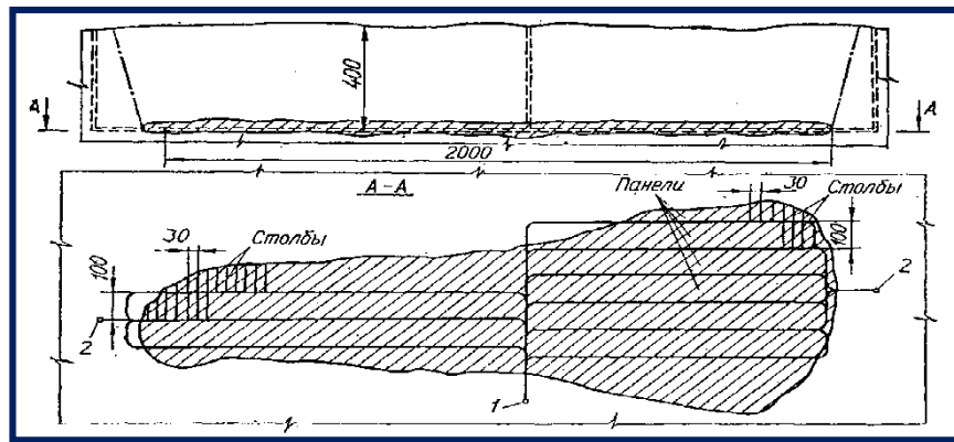
Рис. 2.1. Деление горизонтального месторождения на панели и столбы:
