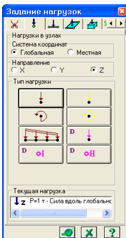
11-рasm. Юкларни қўйиш мулоқот ойнаси
