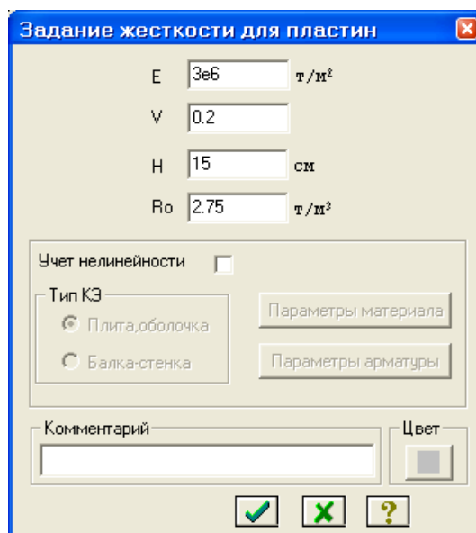
8-расм. Пластина учун бикрлик бериш мулоқот ойнаси
