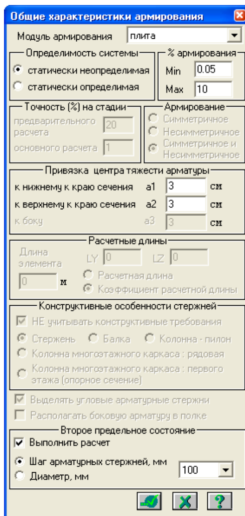
18-расм. Арматуралашнинг умумий характеристикалари мулоқот ойнаси
