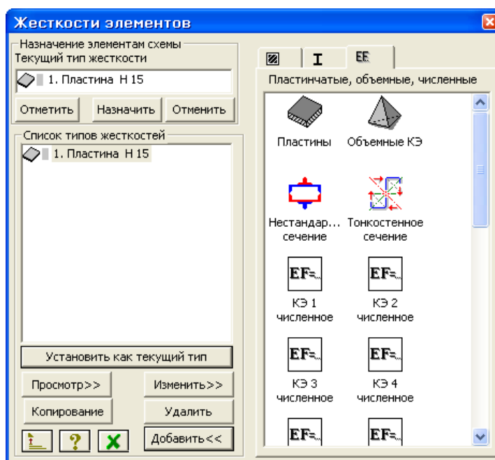
7-расм. Элементлар бикрлиги мулоқот ойнаси
