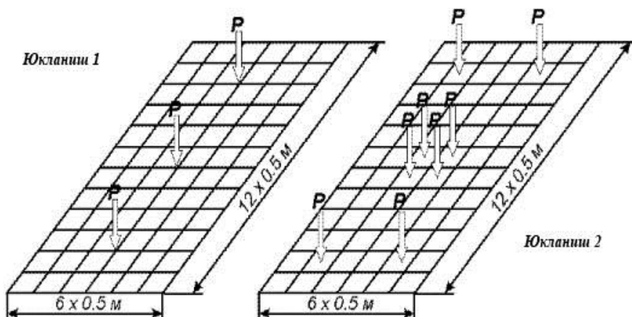
1-расм. Плитанинг ҳисоб схемаси
