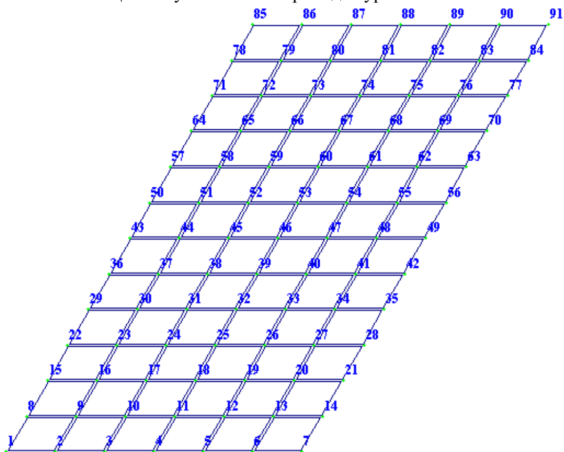
5-расм. Плита ҳисоб схемаси тугунларининг рақамланиши.
