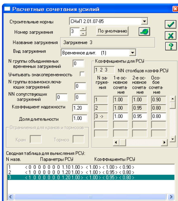
13-расм. Ҳисобий зўриқишлар жамламаси таъсири мулоқот ойнаси
