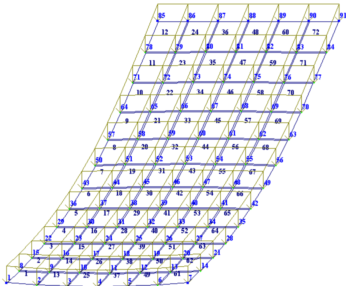
14-расм. Ҳисоб схемасининг кўчишлар ҳисобга олинган ҳолдаги кўриниши
