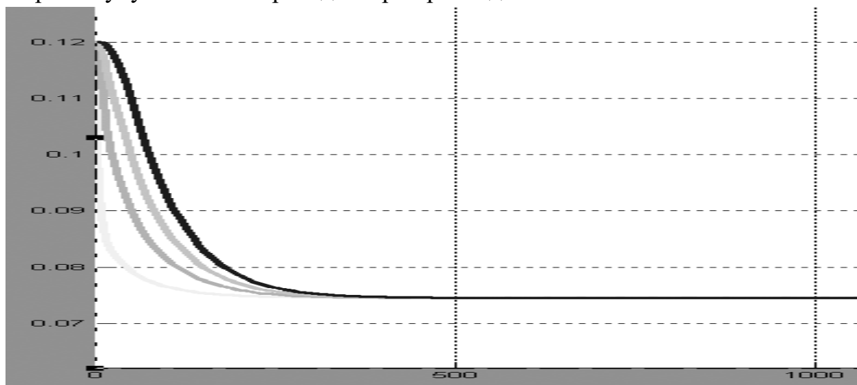
Расм.2.6 .Пахта чигити гул мойили маҳсулотни муаллақ ҳолатда экстракциялаш жараёнининг фикрий қатламларида мицелладаги мойнинг ўртача концентрацияси.
