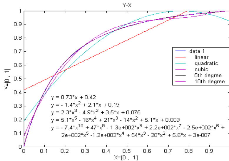
Расм.1.3. Лаурин-пальмитин мой кислоталари аралашмасининг суюкликдаги ва буғ ҳолатидаги концентрацияларинг боғлиқлиги.
