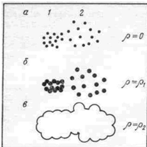
Рис. Функция \Phi(x,y) при различных r
