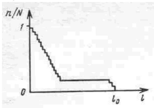
Рис. График n(l)/N
