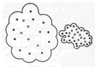
Рис. Граничные точки кластера
