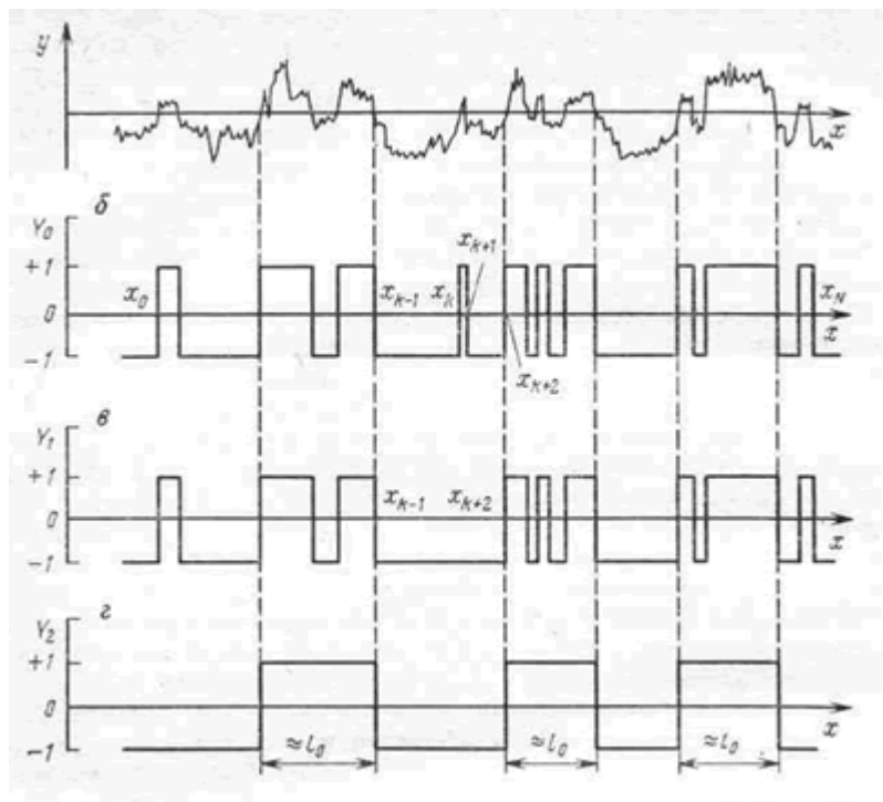
Рис. Разбиение кривой y(x)
