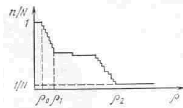
Рис. График n(p)/N
