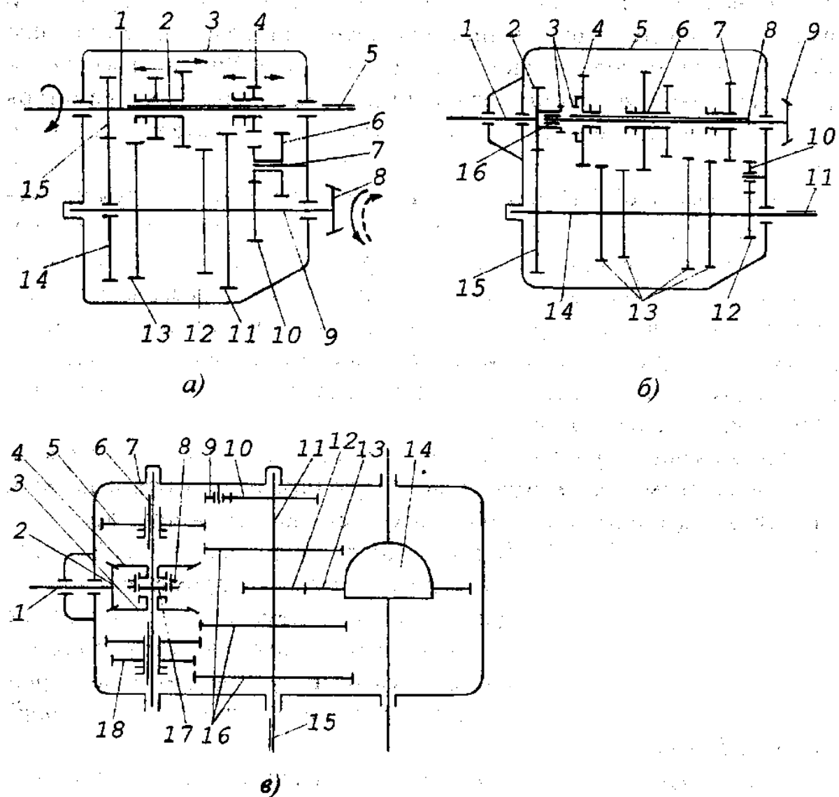
1-расм. Тракторларда қўлланадиган узатмалар қутилари ни принципнал кинематик схемалари
