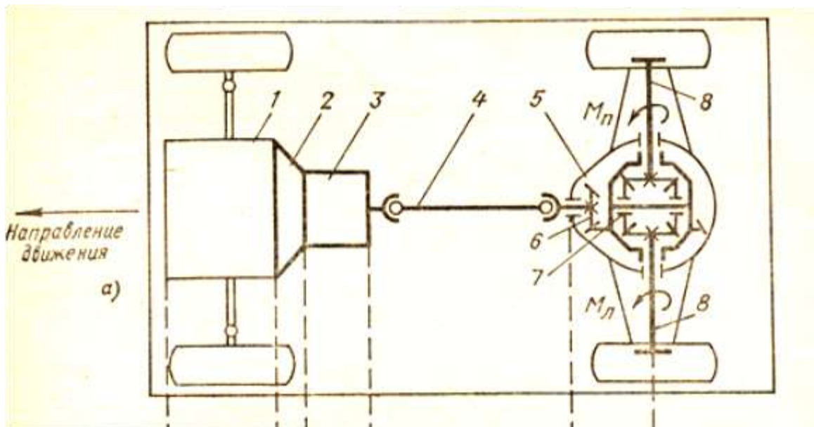
2-расм. Гилдирак схемаси 4x2 бўлган автомобил трансмиссияси схемаси. 1-двигател; 2-тишлашиш муфтаси; 3-узатмалар қутиси; 4-кардан узатмаси; 5-етакчи кўприк корпуси; 6-асосий ёки марказий узатма; 7-дифференциал; 8-ярим ўқлар
