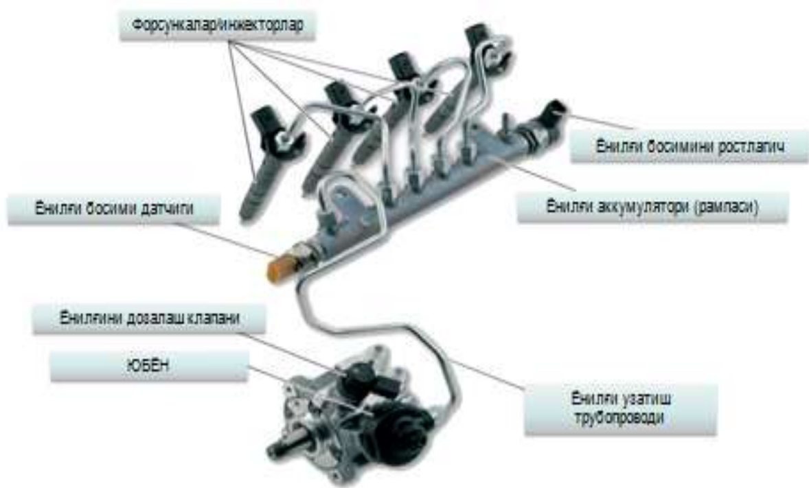
9-расм. Common Rail ёнилги узатиш тизими 22
