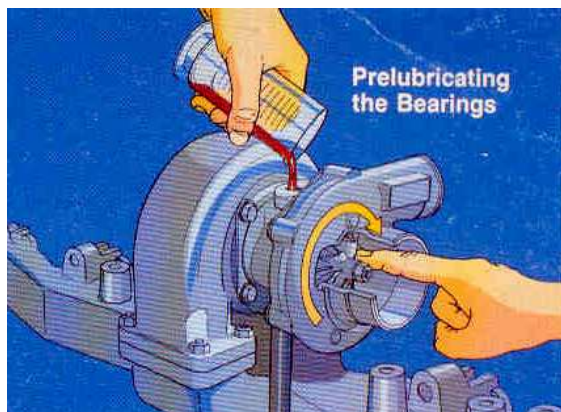
6-расм. Турбокомпрессорларни мойлаш ва совишиш 19
