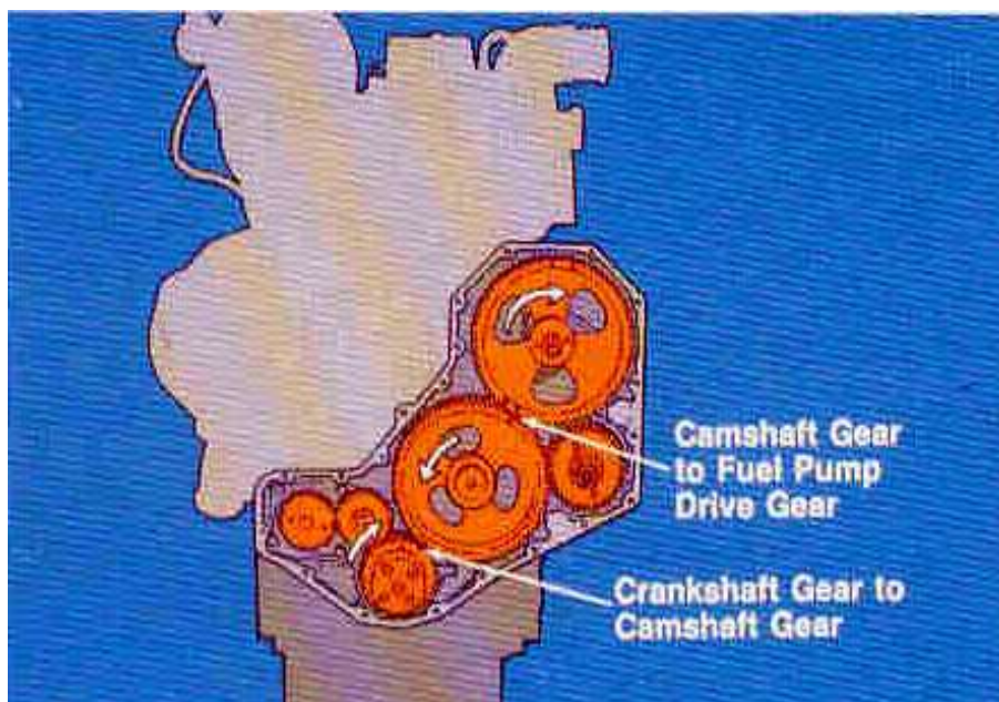
4-расм. Двигателда валларни ҳаракатлантирувчи шестерняларни жойлаштириши 8
