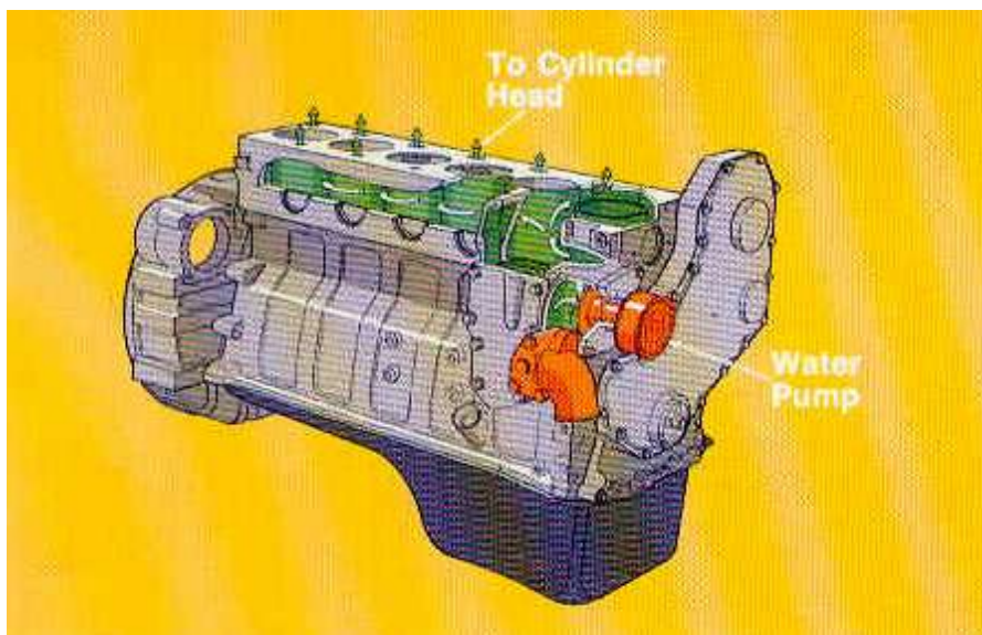
3-расм. Двигател блогида совитувчи суюқликнинг ҳаракатланиши 14
