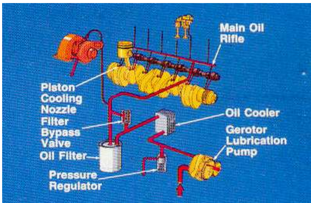
2-расм. Двигател мойлаш тизими элементлари 13
