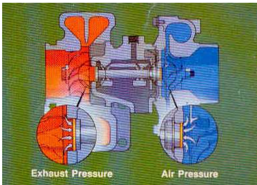
4-расм. Турбокомпрессор секциялари 16
