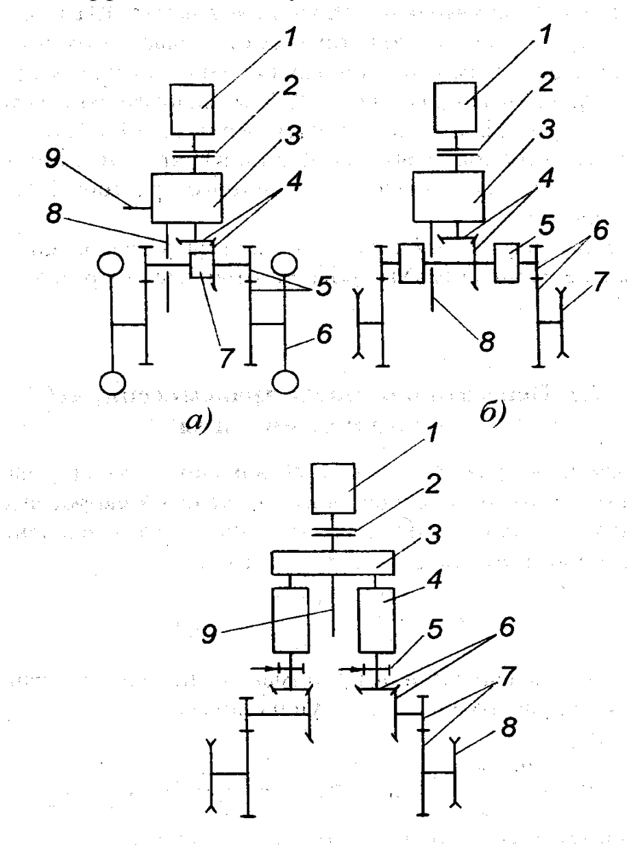
1-расм. Ғилдиракли ва занжирли тракторларнинг трансмиссиялари принципиал схемалари.
