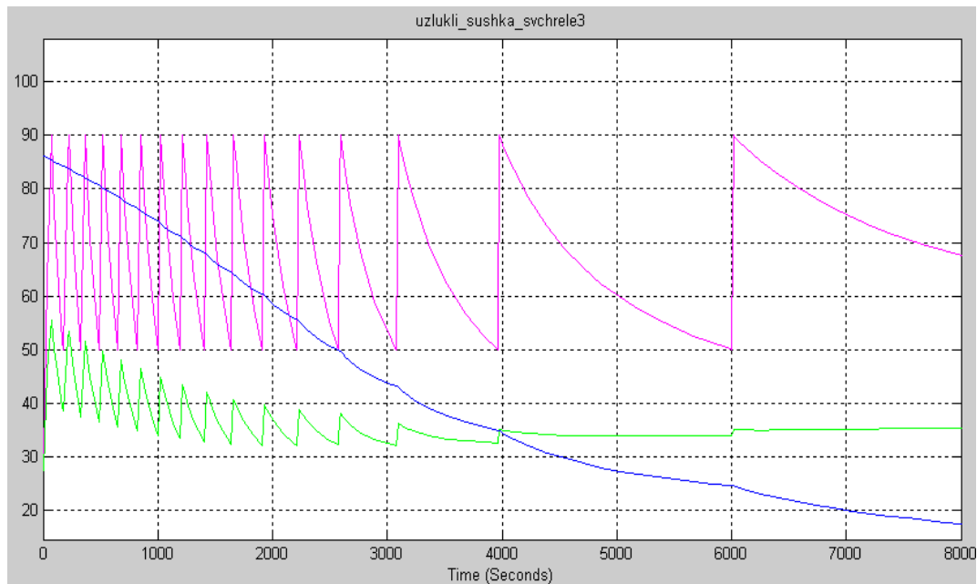
Расм-2.9. Вақт мобайнида материал ҳароратини дискрет иссиқлик узатишдаги оптимал ўзгариши, юқоридаги эгри чизик-ҳақиқий ҳарорат, пастки эгри чизик -мувозанатдаги ҳарорат.
