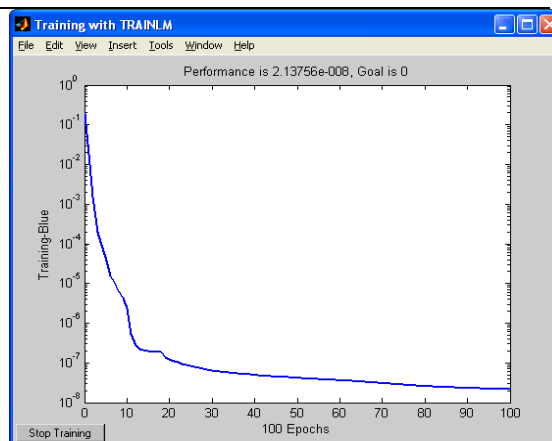
1.7-расм. Ўргатиш жараёнида хатоликнинг камайиб бориши.
