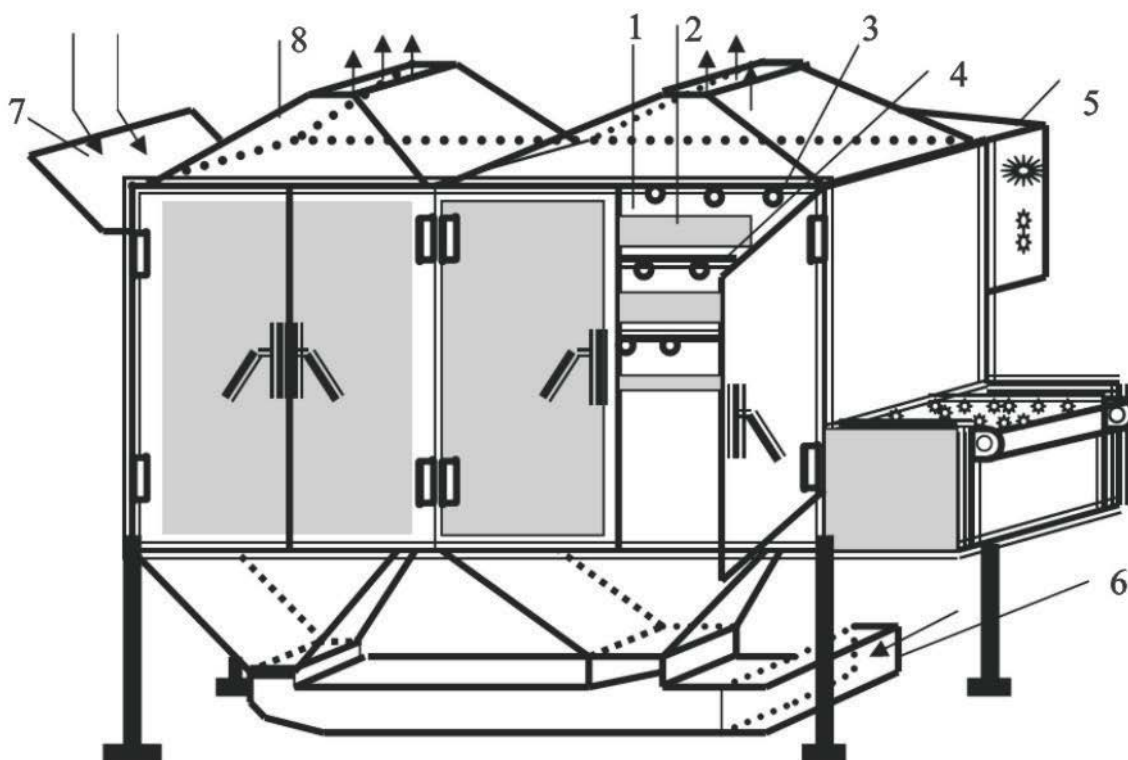
Расм.2.4. ИК - узлуксиз ишловчи конвектив қуриштириш қурилмаси. 1- камера; 2- транспортер; 3- ИК -лампа; 4-рефлектор; 5- шит; 6- коммунокация; 7- юкловчи қурилма; 8-тортувчи.
