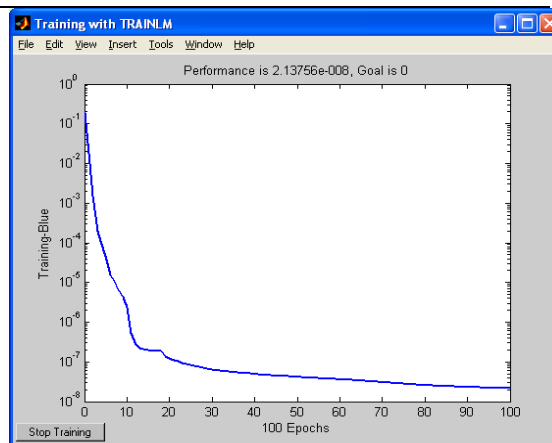
1.7-расм. Ўргатиш жараёнида хатоликнинг камайиб бориши.
