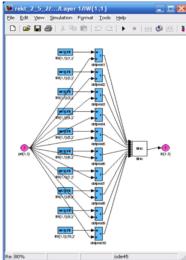
1.10-расм. Нейрон тўр биринчи қатламнинг салмоқлари.
