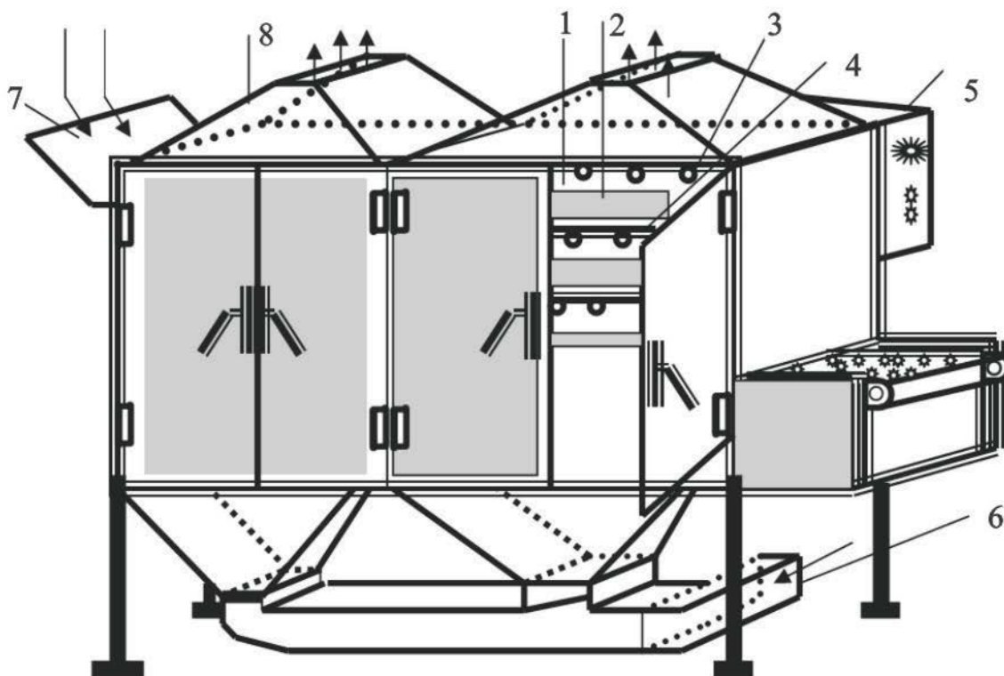
Расм.2.4. ИК - узлуксиз ишловчи конвектив қуритиш қурилмаси. 1- камера; 2- транспортер; 3- ИК -лампа; 4-4-рефлектор; 5- шит; 6- коммунокация; 7- юкловчи қурилма; 8-тортувчи.
