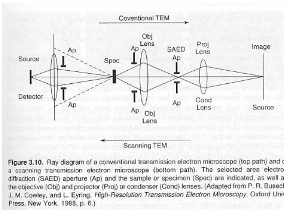
Расм 1. Сингиб ўтиш электрон микроскопнинг (ТЕМ) ишлаш принципи
