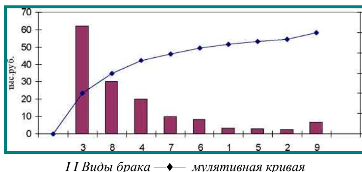
Рисунок 1 - Диаграмма Парето для анализа брака кровельных листов
