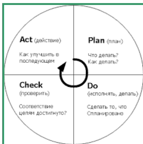
Рис. 4. PDCA-цикл
