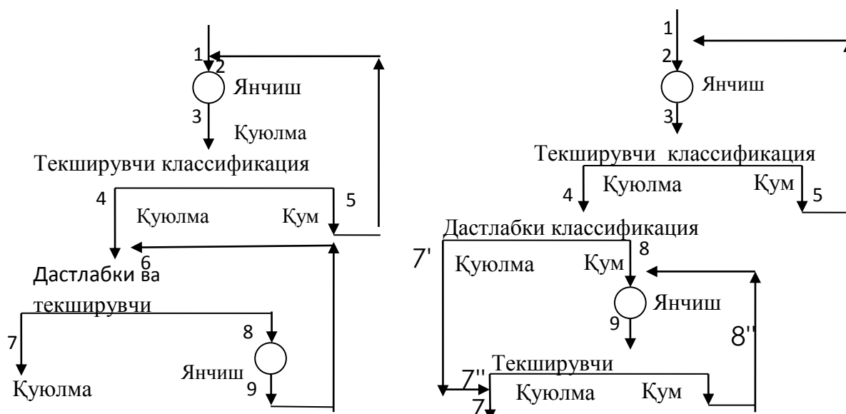
Икки босқичли янчиш схемалари.
