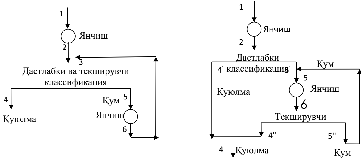
Икки босқичли янчиш схемалари
