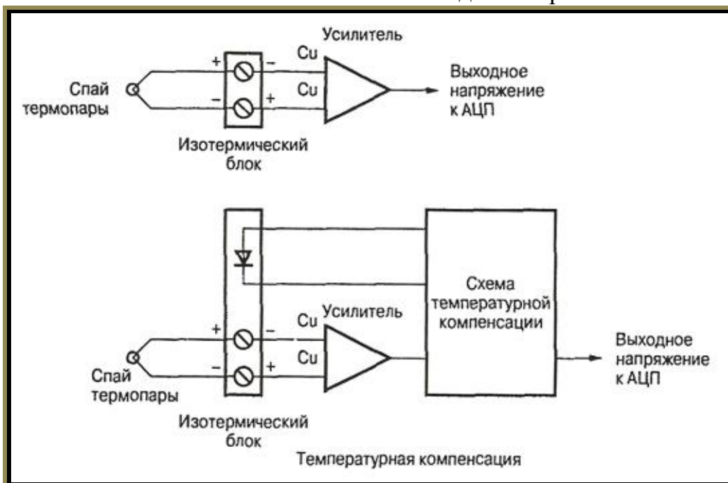
Рис. 1 Термопара
