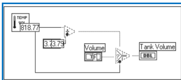
Рис. 42 Соединение блоков.
