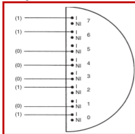
Рис. 3 Простая схема аппаратных средств для декодирования восемь адресных линий
