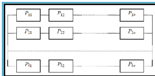
Рис.3 Структурная схема надежности с поканальным резервированием
