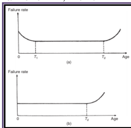
Рисунок 1. Типичные изменения надежности со временем:
