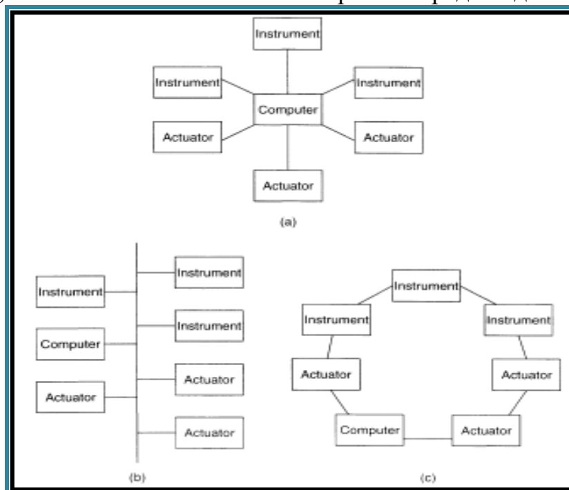
Рис. 5 Сетевые протоколы: (а) звезда, (б) автобус, и (с) кольцо
