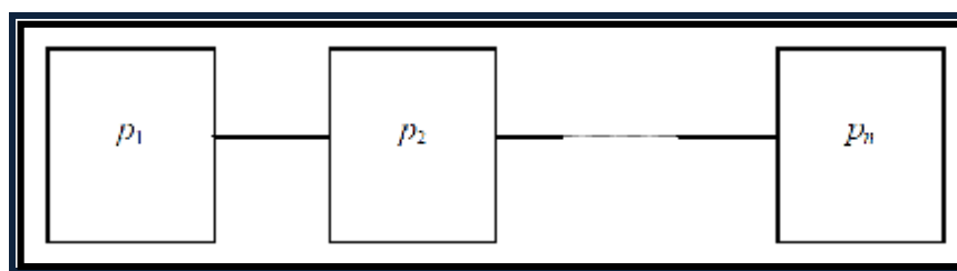
Рис. 3 Структурная схема надежности системы с последовательным соединением элементов
