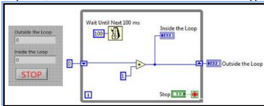
Рисунок 9 Пример контура VI
