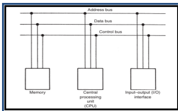
Рис. 1 Элементы микрокомпьютера
