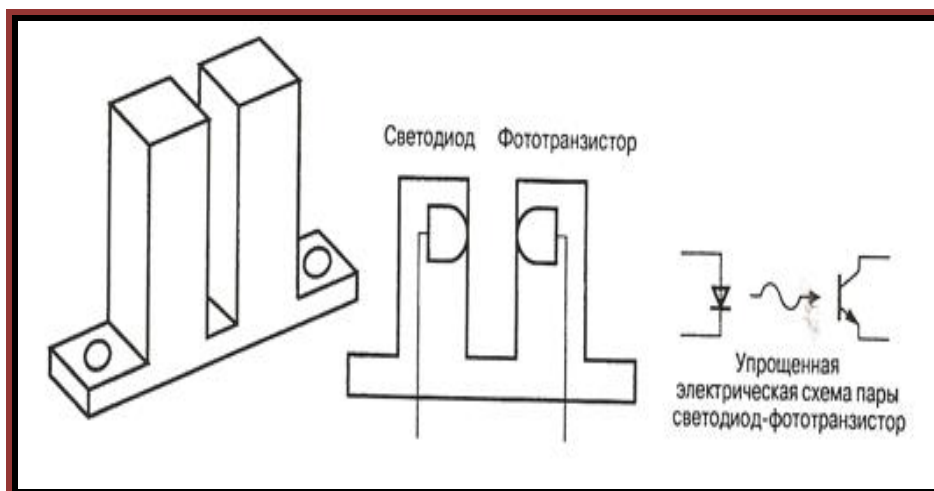
Рис. 3 Оптический датчик — щелевой оптрон
