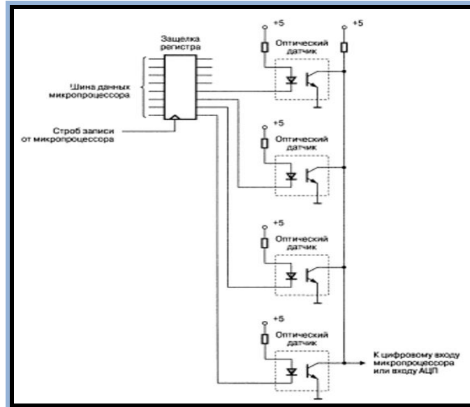
Рис. 5 Несколько оптронов с общим выходом
