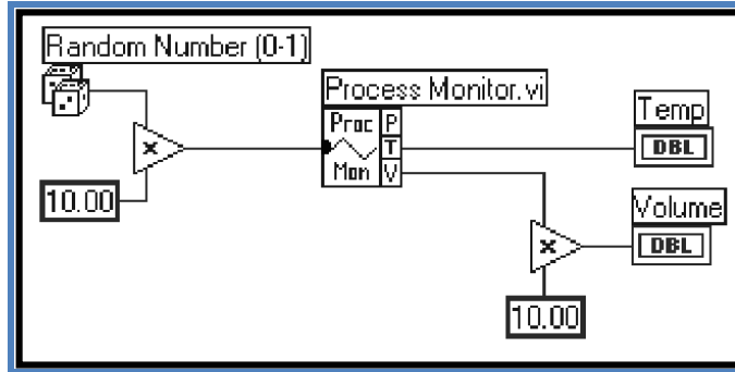
Рис. 36 Соединение блоков
