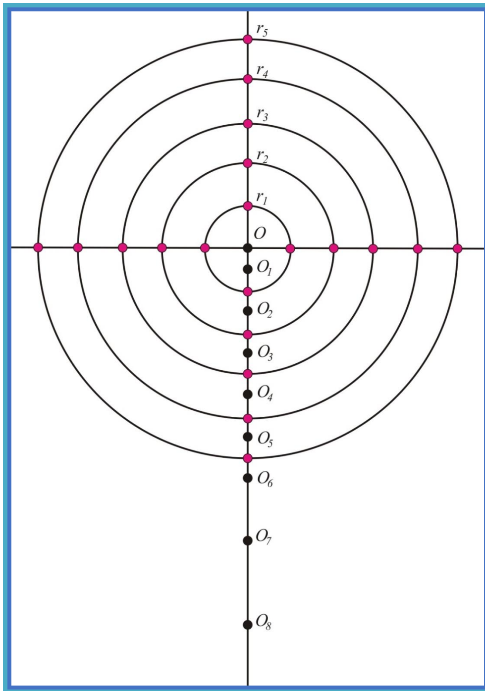
Рис. 1. Схема диска с выступами, контактирующими с шероховатой поверхностью, для вычисления их путей контакта в центричном, эксцентричном и бицентричном режимах вращения
