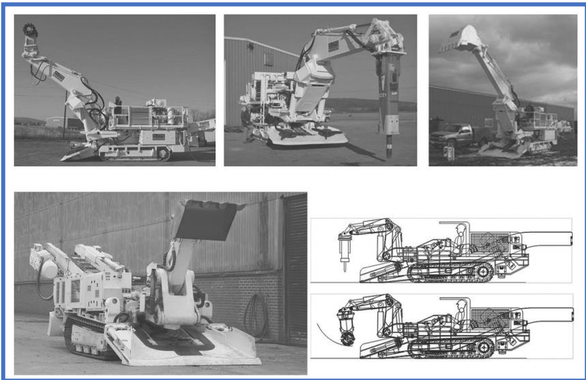
Рисунок 1.9. Взаимозаменяемая стрела проходческого комбайна.
