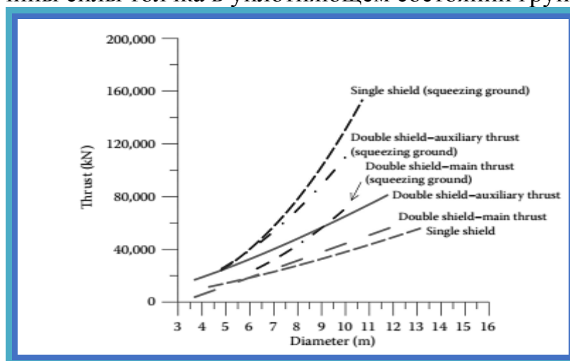
Рисунок 2.7. Зависимость между диаметром и толчком для однощитного и двухщитного проходческого комбайна.
