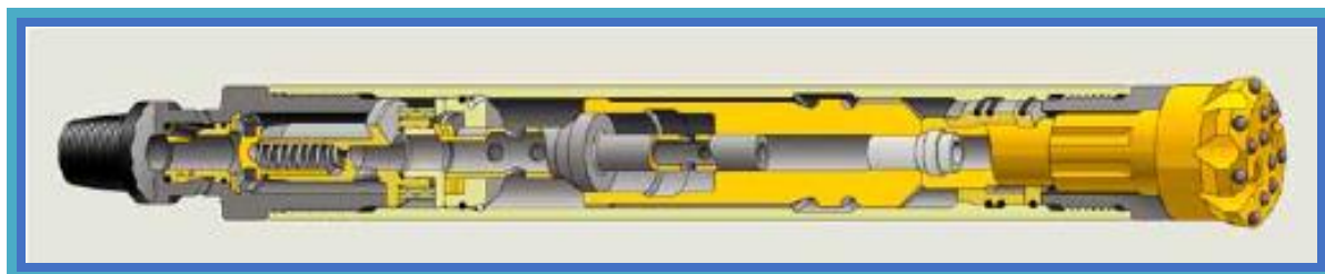
Рис-6. Пневмоударник «Золота Secogoc СОР64»
