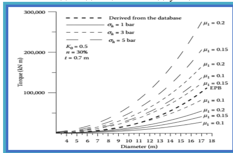
Рисунок 2.10. Зависимость между диаметром проходческого комбайна и вращающим моментом для однощитного и двухщитного комбайна.
