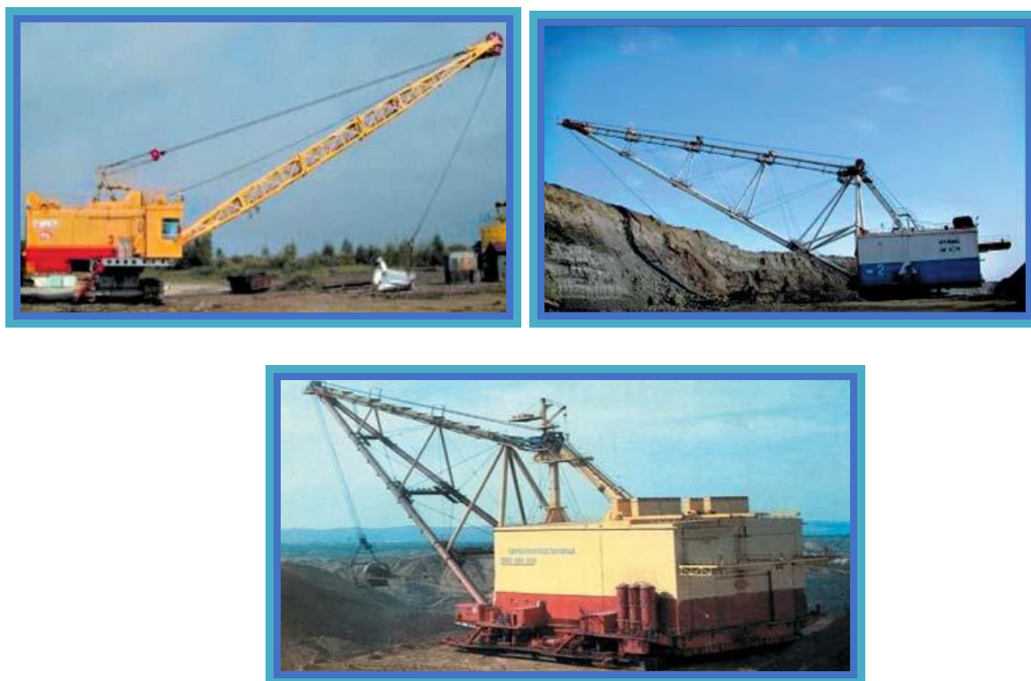
Рис. 11. Экскаваторы-драглайны производства УЗТМ: а - гусеничный драглайн ЭДГ-3,2.30; б - шагающий ЭШ 11.75; в - шагающий ЭШ 100.100
