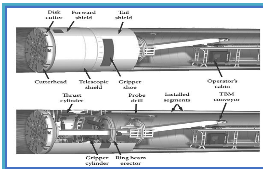
Рисунок 2.4. Общее вид двух щитного проходческого комбайна.
