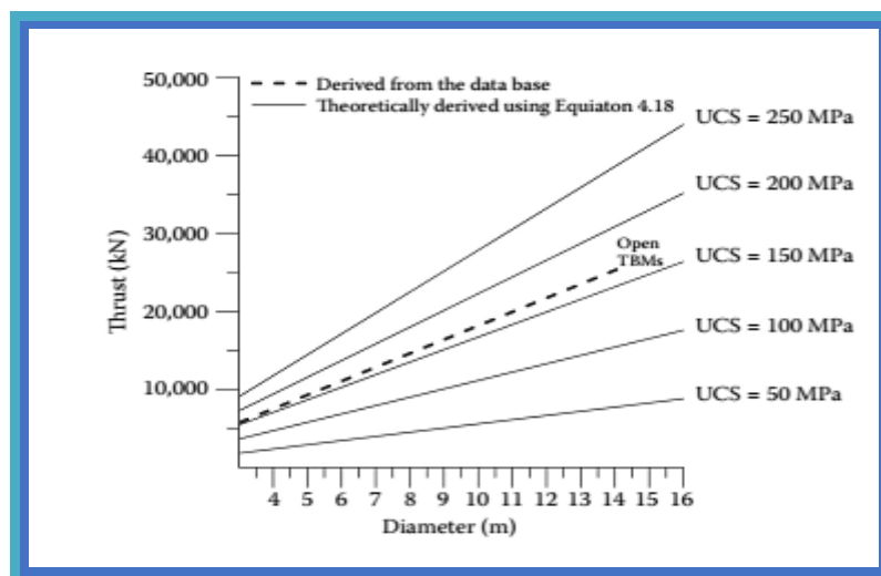
Рисунок 2.6. Зависимость между диаметром и толчком для открытого типа щитовых проходческих комбайнов для различной прочности на сжатие камня.
