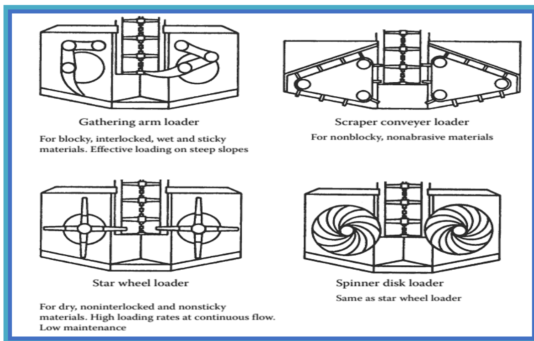
Рисунок 1.10. Общие типы погрузочного оборудования для различного типа горных пород.
