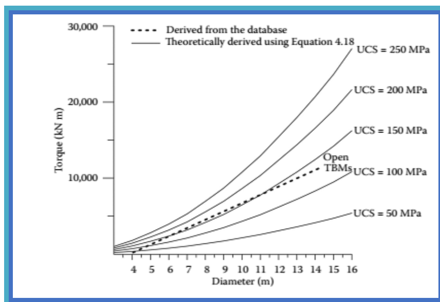
Рисунок 2.9. Зависимость между диаметром щитового проходческого комбайна и вращающим моментом открытого типа.
