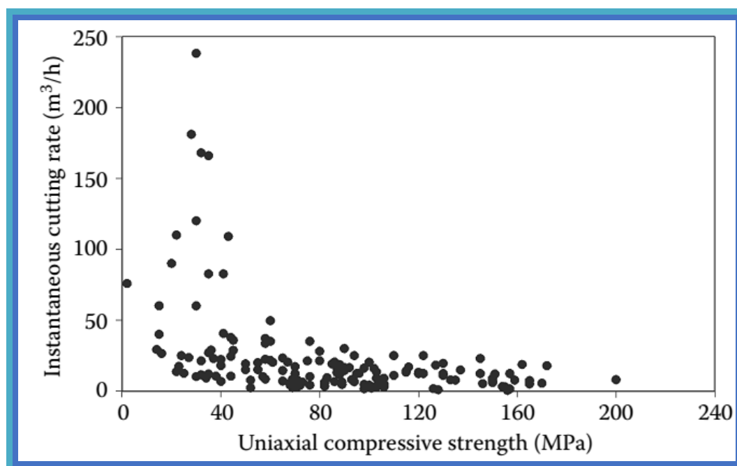
Рисунок 1.2. Связь между силой сжатия рабочего органа с производительностью для проходческих комбайнов
