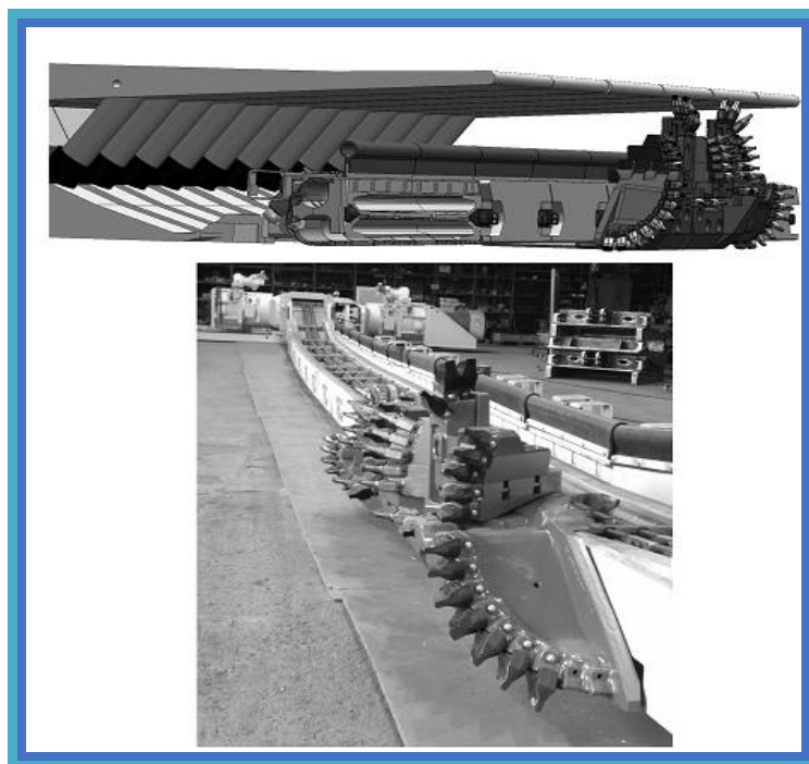
Рисунок 3.4. Общий вид струговой установки.
