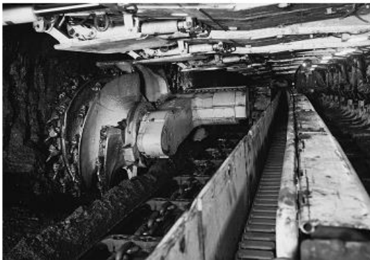
Рисунок 3.3. Общий вид шнекового рабочего органа в забое.
