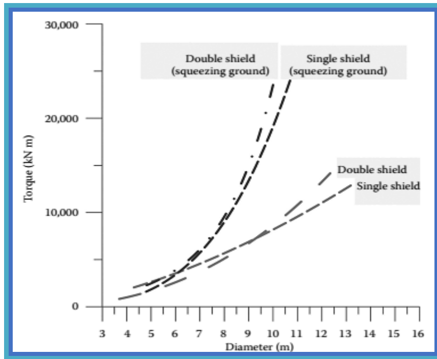
Рисунок 2.10. Зависимость между диаметром проходческого комбайна и вращающим моментом для однощитного и двухщитного комбайна.
