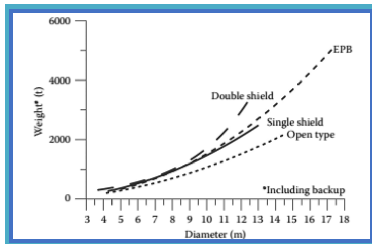
Рисунок 2.14. Зависимость между диаметром щитовых проходческих комбайнов и весом для различных типов комбайнов.
