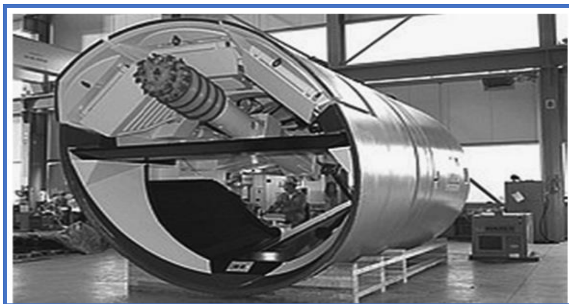
Рисунок 1.5. Шитовой проходческий комбайн (Сандвик)
