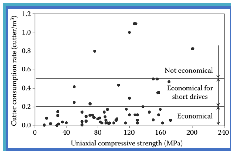
Рисунок 1.4. Связь между силой сжатия рабочего органа с расходом резцов для проходческих комбайнов.
