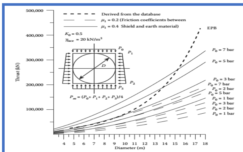
Рисунок 2.8. Зависимость между диаметром щитового проходческого комбайна и толчком для балансировки давления на почву.
