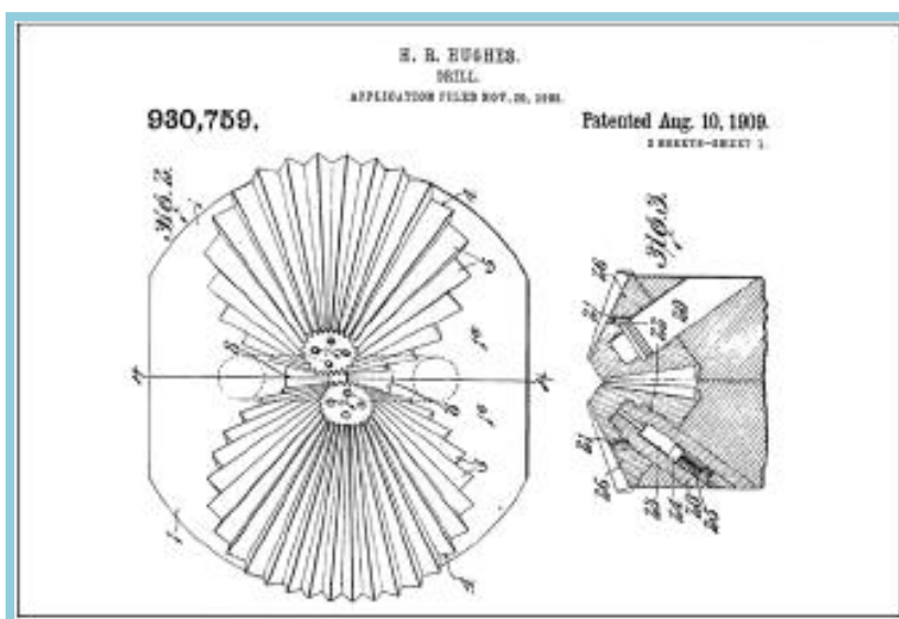
Рис-4. Американский патент для двухпьеверного коронки, был выпущен Говарду Хьюзу старшему в 1909
