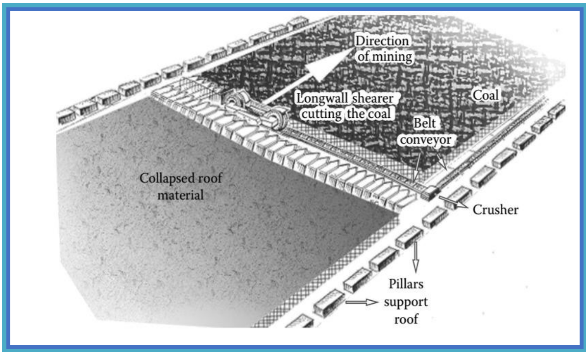
Рисунок 3.2. Вид в плане работ механизированного угольного сплошного забоя.
