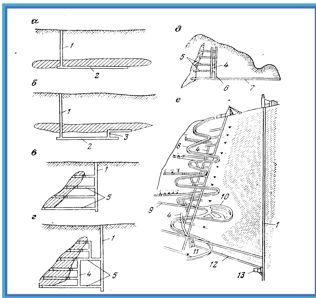
Рис. 1. Схемы вскрытия рудных месторождений:
