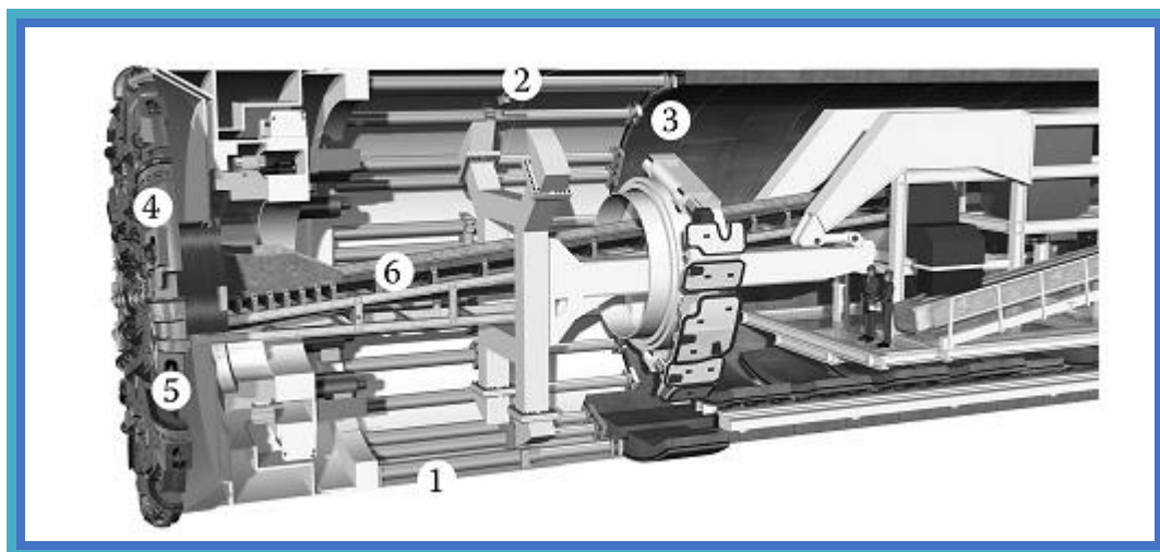
Рисунок 2.3. Общее вид однощитного проходческого комбайна.
