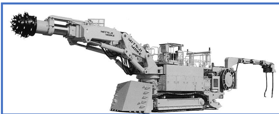
Рисунок 1.7. Телескопическая и сочлененная стрела проходческой машины.
