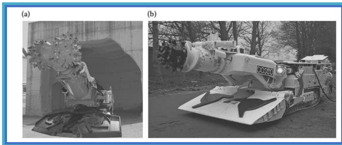
Рисунок 1.1. Радиальные и осевые типы проходческих машин избирательного действия. Машины с (а) радиальными органами избирательного действия и (b) осевыми органами избирательного действия.
