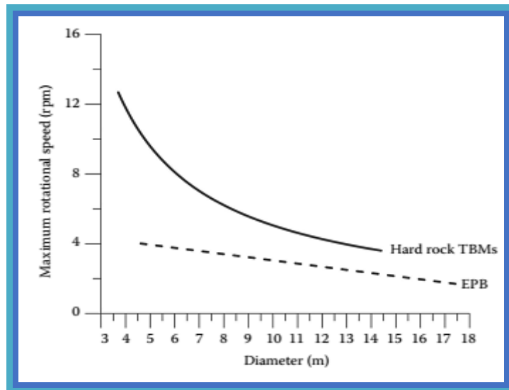
Рисунок 2.12. Зависимость между диаметром щитовых проходческих комбайнов и угловой скоростью для всех типов комбайнов
