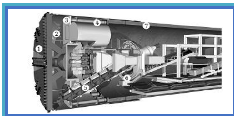
Рисунок 2.5. Общее мнение EPB TBM. (С любезностью Herrenknecht.)
