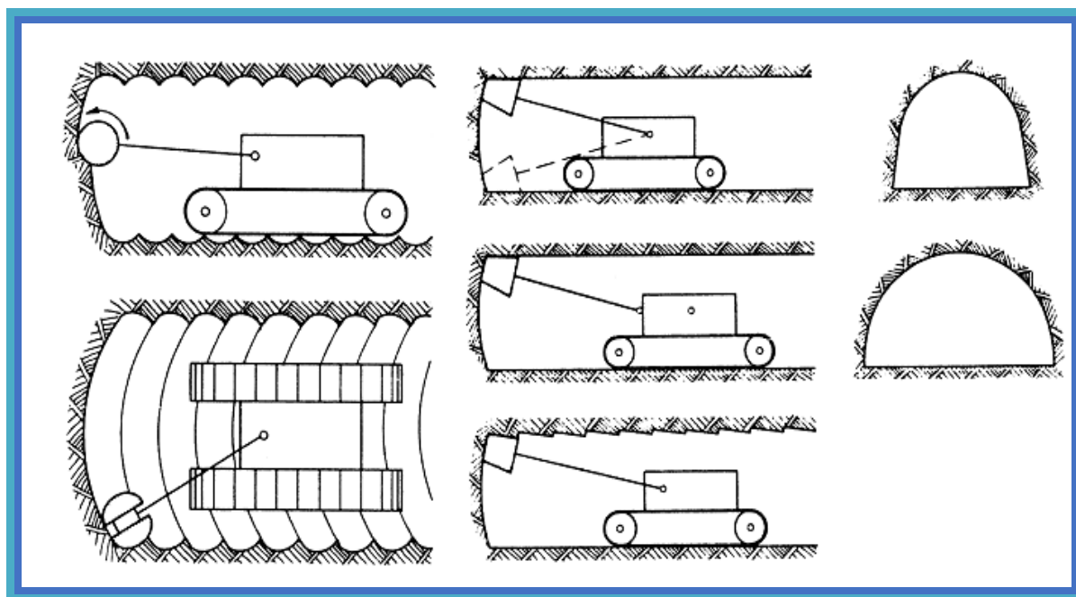
Рисунок 1.11. Проходка с помощью проходческих комбайнов с радиальным (левое) и осевым (правое) рабочим органом.
