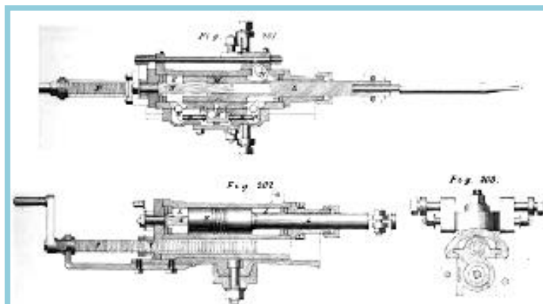
Рис-2. Буровая машина Ингерсолла
