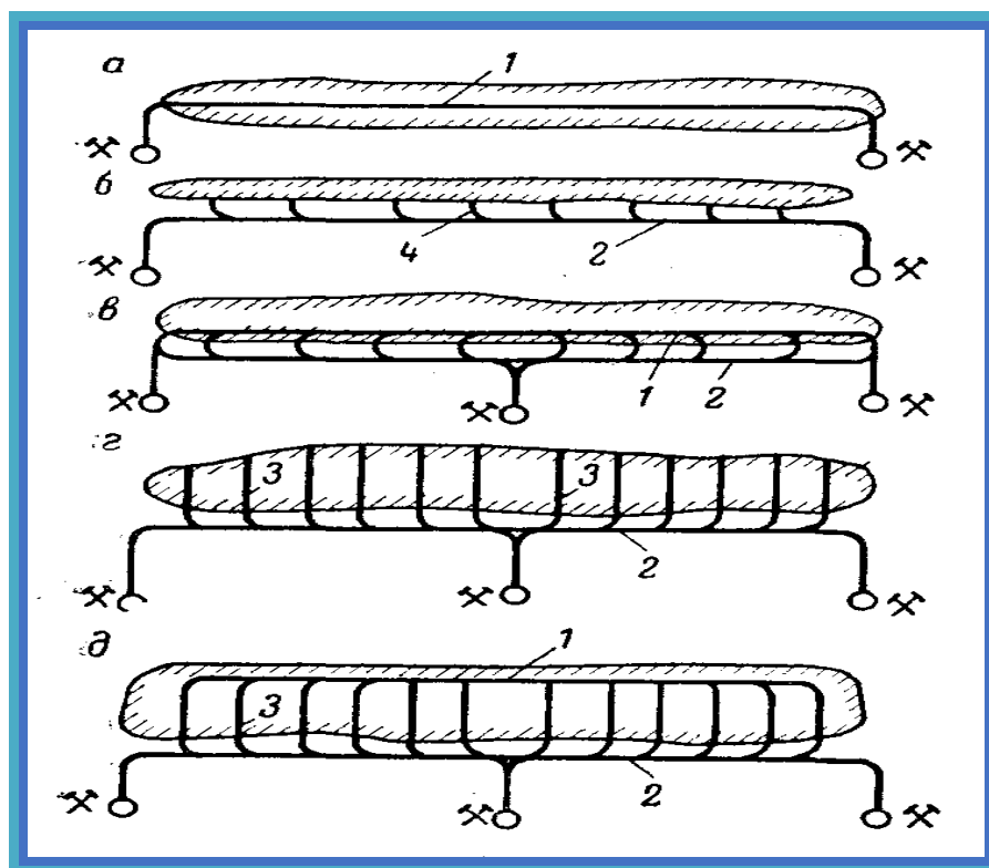
Рисунок 2. Схемы способов подготовки:
