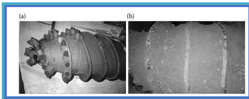
Рисунок 1.3. Чистый рабочий орган проходческой машины (a) и после застревающей глины (b).
