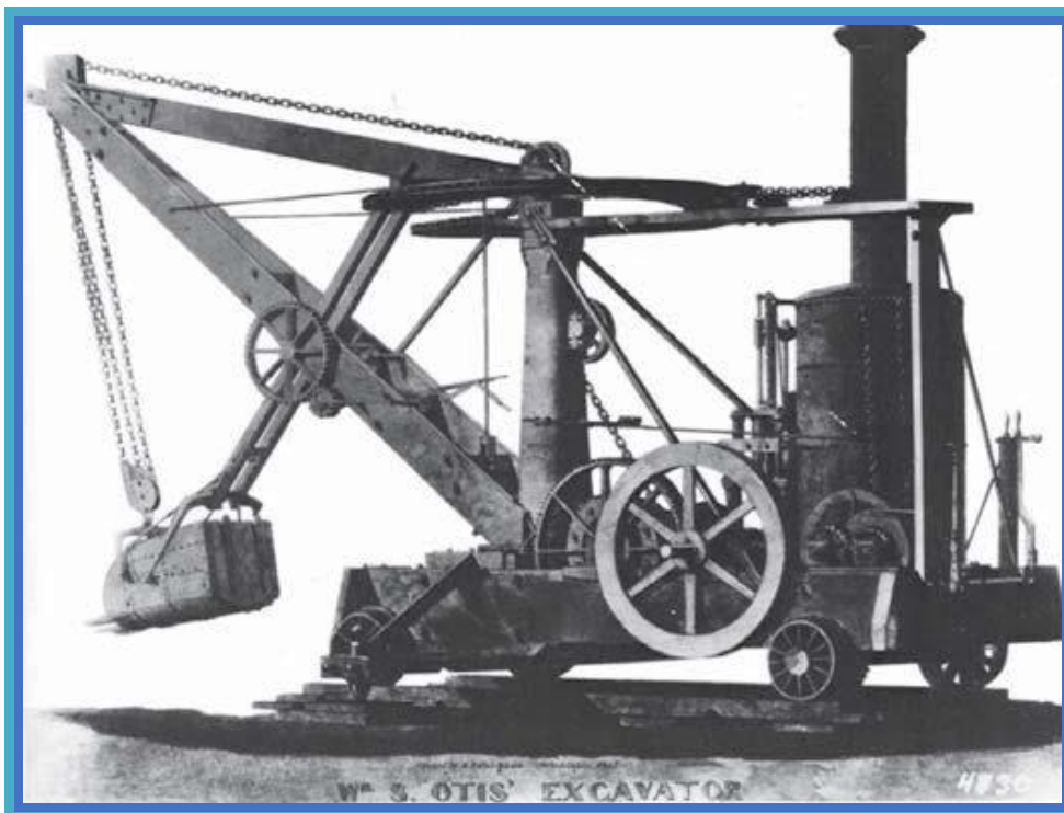
Рис. 1. Прямая механическая лопата Otis с речной системой напора и паровой силовой установкой
