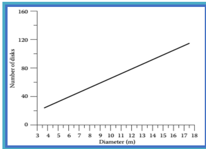
Рисунок 2.13. Зависимость между диаметром щитовых проходческих комбайнов и числом дисков на рабочих органах.
