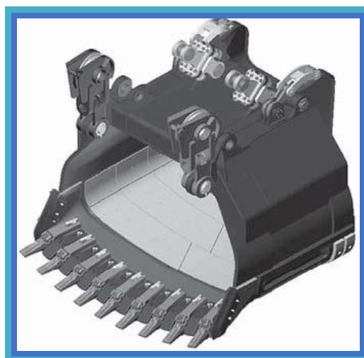
Рис. 3. Ковш конструкции FastFil с оптимизированной геометрией
