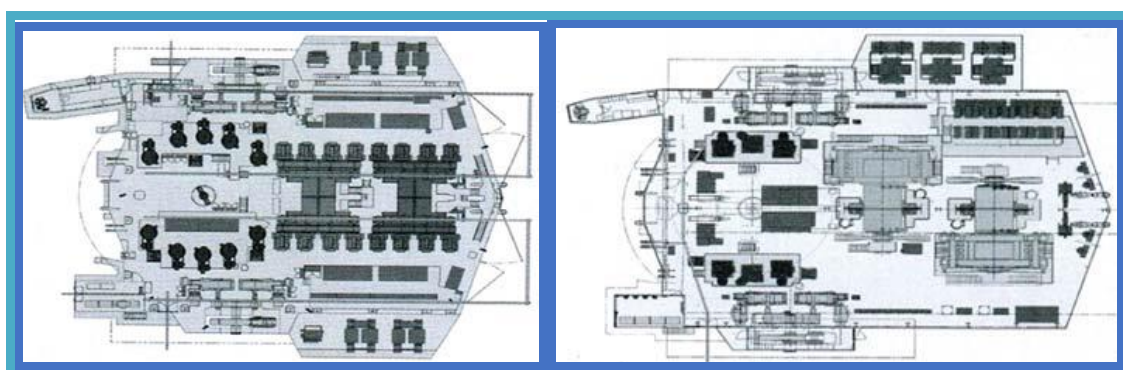
Рис. 14. Расположение механизмов на поворотных платформах шагающих драглайнов компании Caterpillar: а – модель 7850В с традиционными редукторными приводами лебедок подъема и тяги; б – модель 7850D3 с прямыми безредукторными приводами лебедок подъема и тяги
