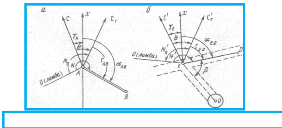
Рис. 10.6. Схема гироскопического ориентирования на земной поверхности (а) и в шахте (б)
