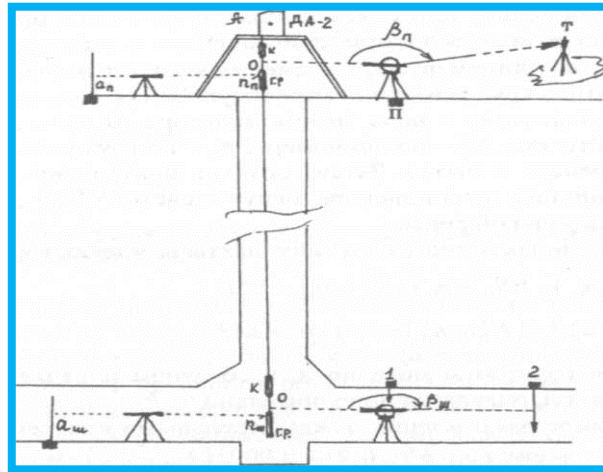
Рис. 10.8. Порядок работ по передаче координаты Z с поверхности в подземную выработку
