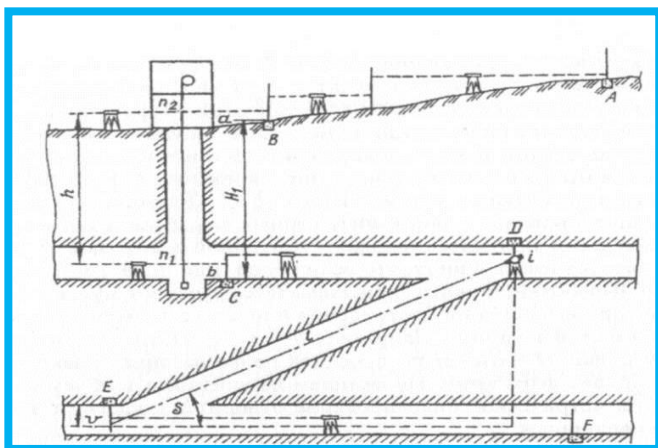
Виды подземной вертикальной съемки
