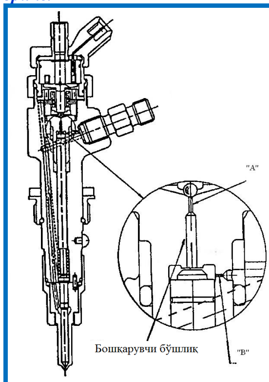
Электрогидравлик форсунканинг тузилиши
