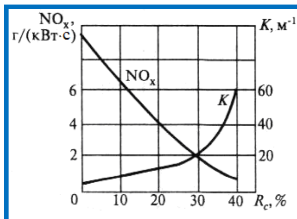
3.6-расм. R_c рециркуляция даражасининг NO_x чиқиши ва оқим ёриқлиги пасайишининг натурал кўрсаткичига таъсири ( n=2000 мин -1 ; p_e=0,2 МПа)
