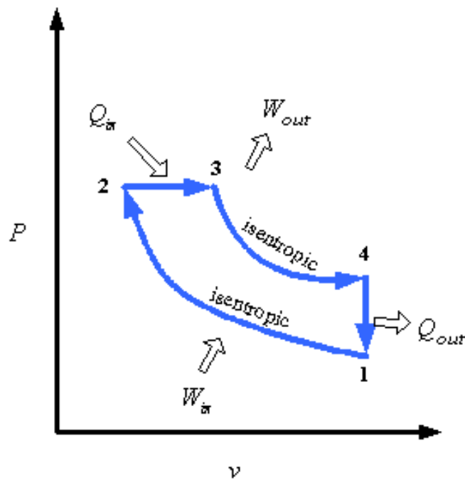
8-расм. Дизелли циклниң P-V диаграммаси
