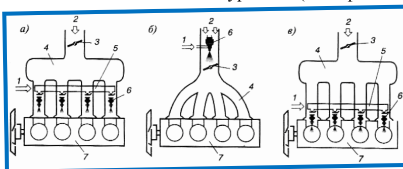
2.2-расм. Бензинни пуркаш тизимлари: а – тақсимланган пуркаш; б– марказий пуркаш; в – цилиндрга бевосита пуркаш; 1– ёнилғи келтирилиши; 2 – ҳаво келтирилиши; 3 – дроссел тўсиги; 4 – киритиш трубопроводи; 5 – форсункаларга ёнилғини келтириш коллектори; 6 – форсунка; 7 –цилиндрлар каллаги
