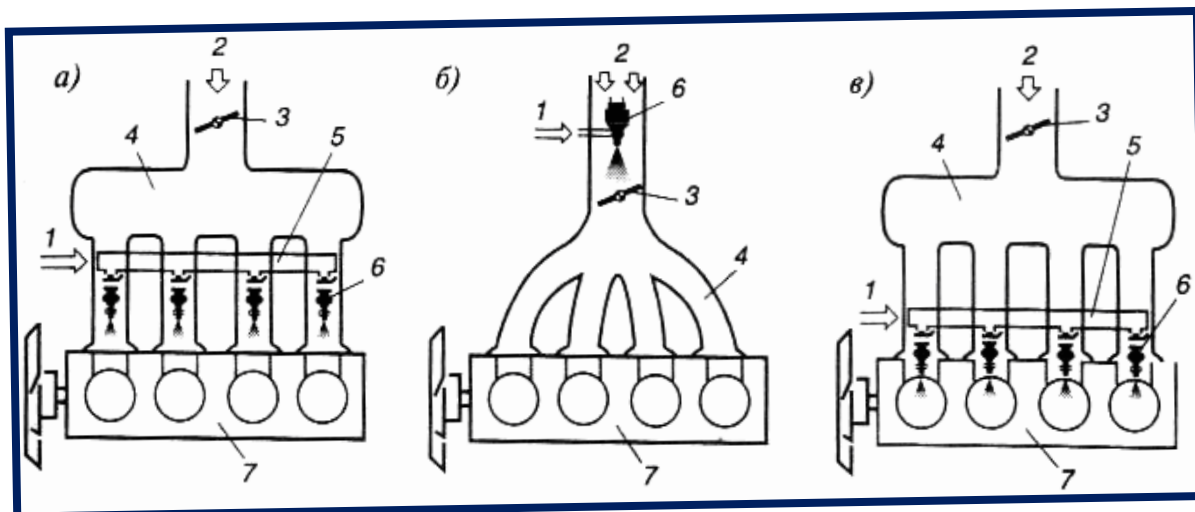
Бензинни пуркаш тизимлари: а – тақсимланган пуркаш; б– марказий пуркаш; в – цилиндрга бевосита пуркаш; 1– ёнилги келтирилиши; 2 – ҳаво келтирилиши; 3 – дроссел тўсиғи; 4 – киритиш трубопроводи; 5 – форсункаларга ёнилгини келтириш коллектори; 6 – форсунка; 7 –цилиндрлар калағи
