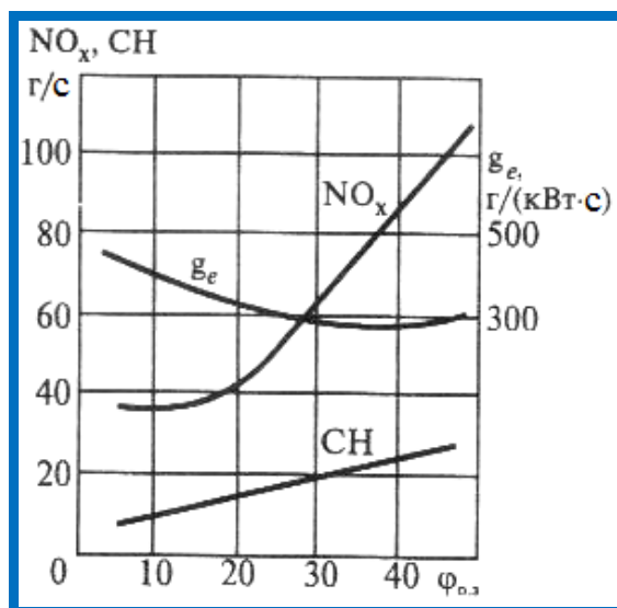
NO_x ва CH ҳосил бўлишига \phi_{0.3} нинг таъсири
