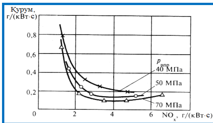
Қурум ва NO_x чиқишлари орасидаги ўзаро боғлиқлик ( n=1500 \text{ мин}^{-1} ; p_e=0,3 \text{ МПа} )
