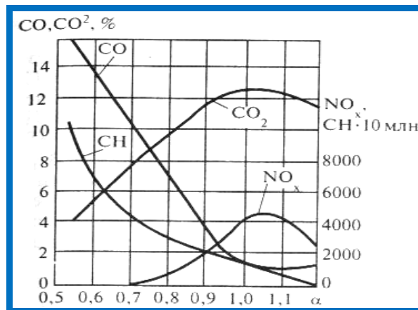
Ишланган газлар таркибига \alpha нинг таъсири
