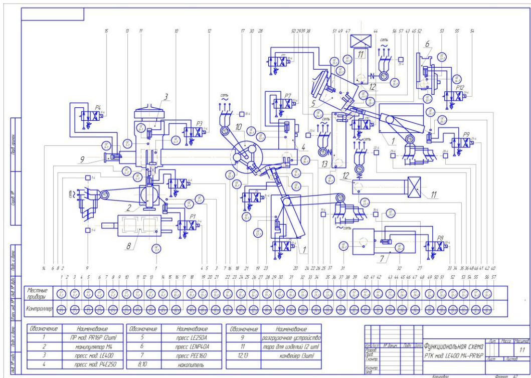
5-расм. AutoCAD дастурида лойихалаш
