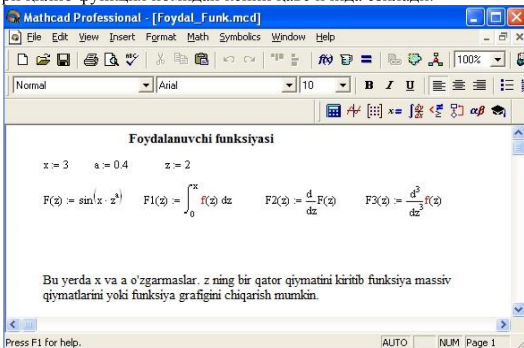
9-расм. Ҳисоблашларда фойдаланувчи функциясини тузиш
