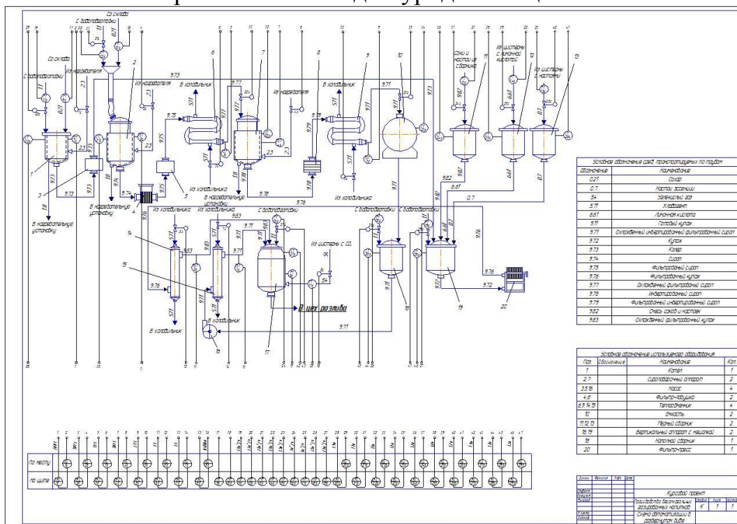
6-расм. AutoCAD дастурида лойихалаш
