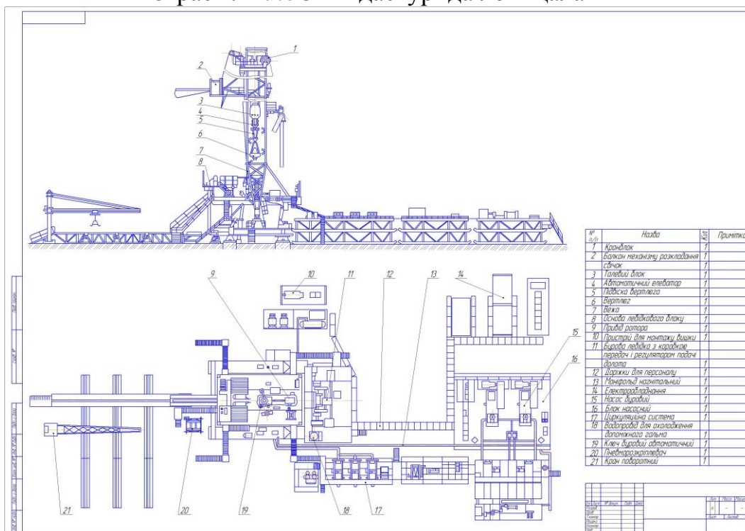
6-расм. AutoCAD дастурида лойиҳалаш
