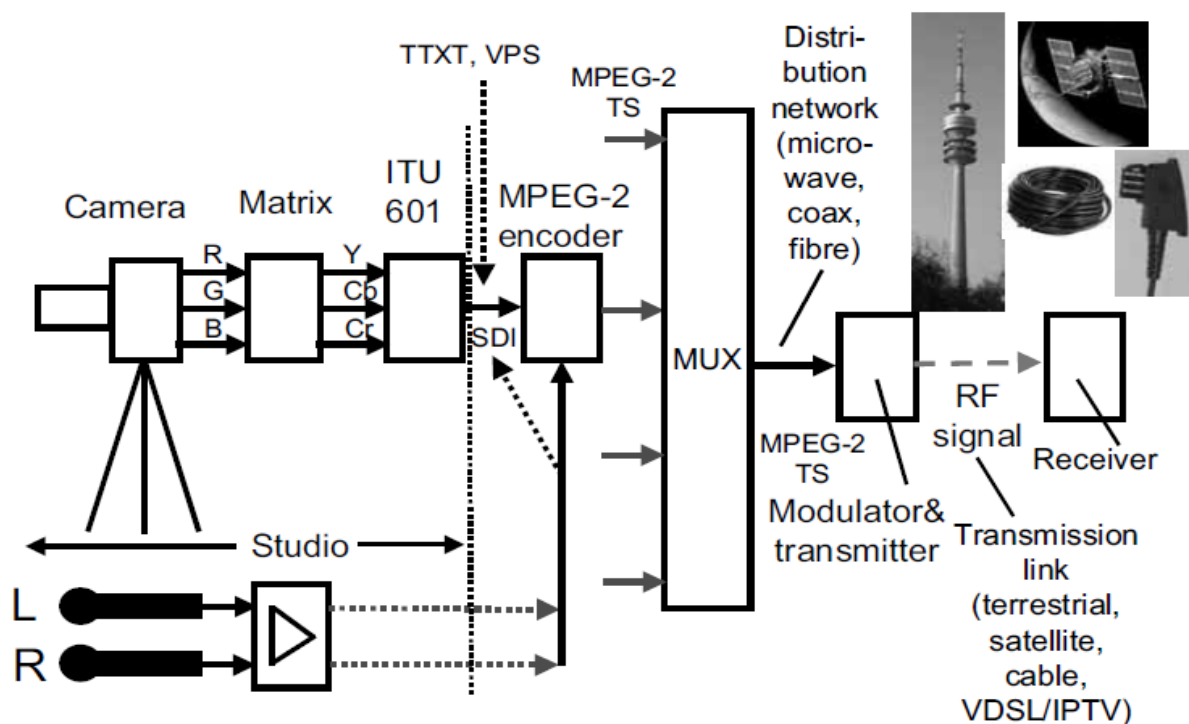
4.13.расм. IPTV ташкил этилиш тармоғи.
