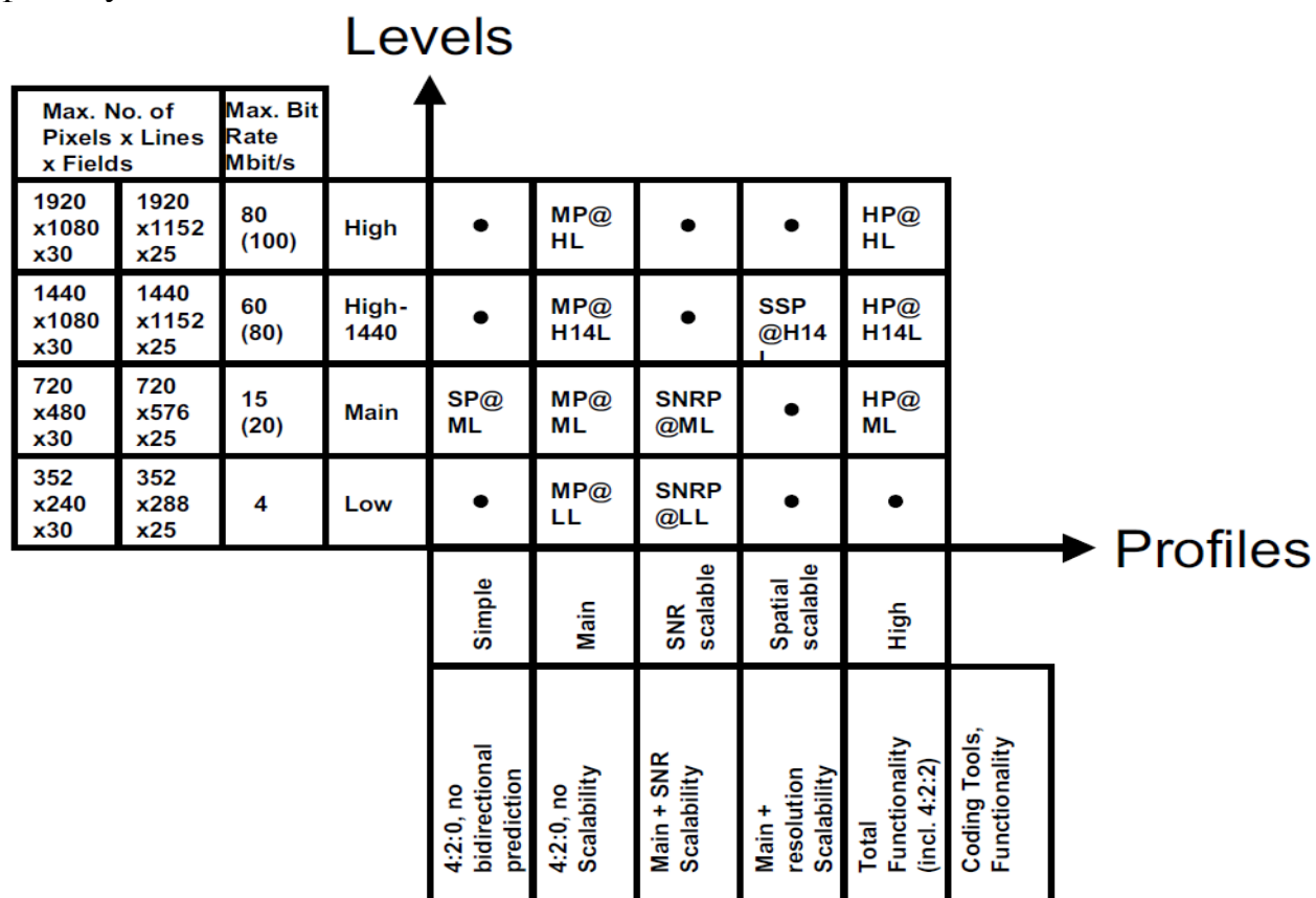
3.13.расм. MPEG-2 профиллари ва даражалари.
