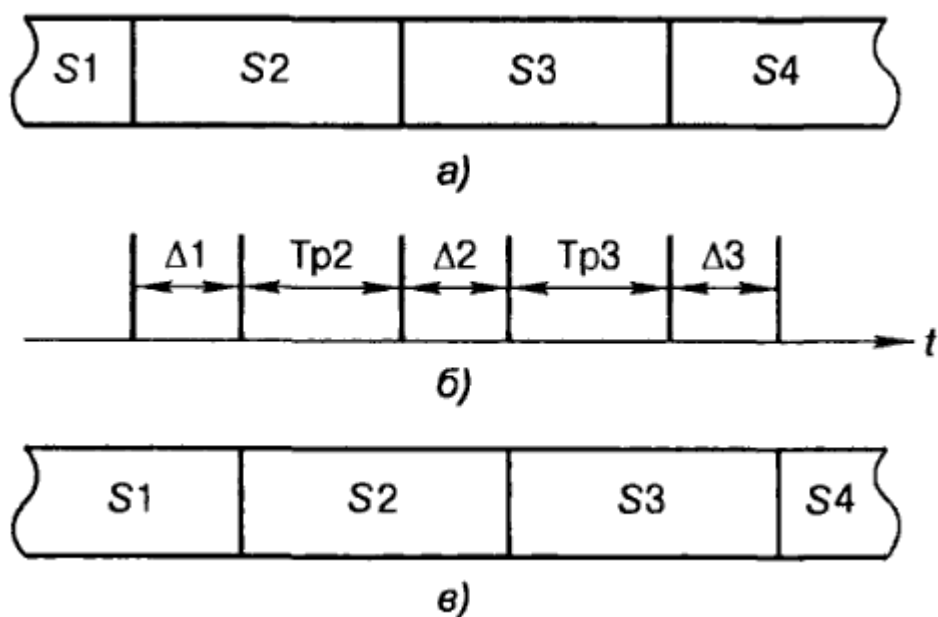
2.18-расм. Ҳимоя интервалларининг шакллантирилиши
