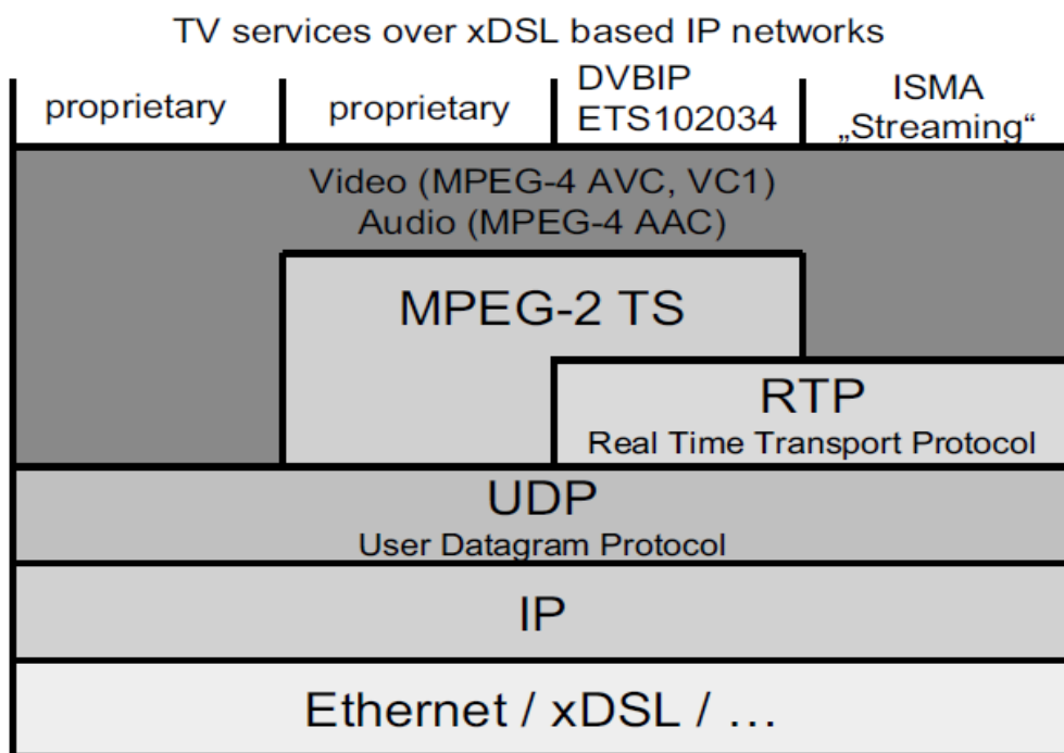
4.14.расм. IPTV протоколлари.
