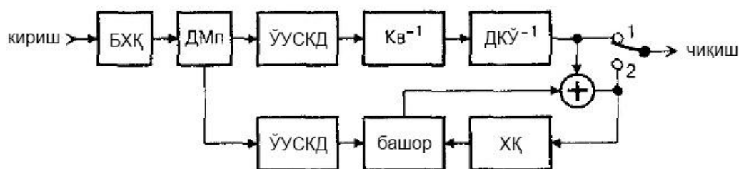
3.21-расм. MPEG-2 видеодекодер тузилмавий чизмаси
