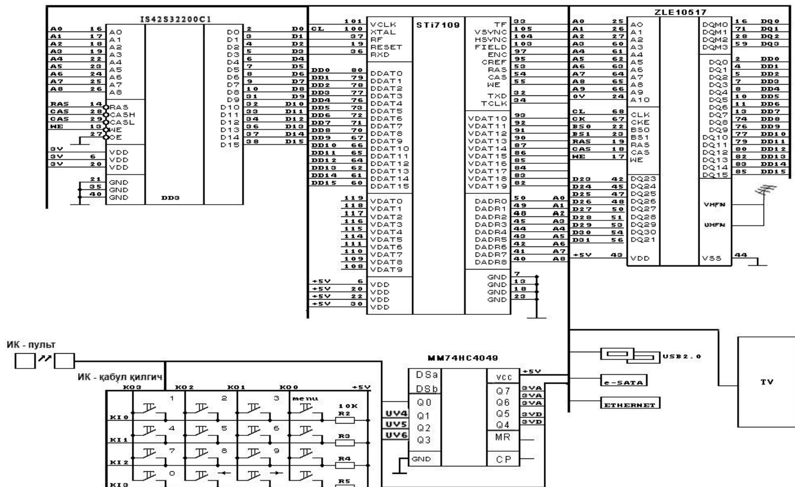
5.21-расм. MPEG 4 стандарти DVB-T қабул қилувчи қурилмасынинг соддалаштирилган шартли чизмасы
