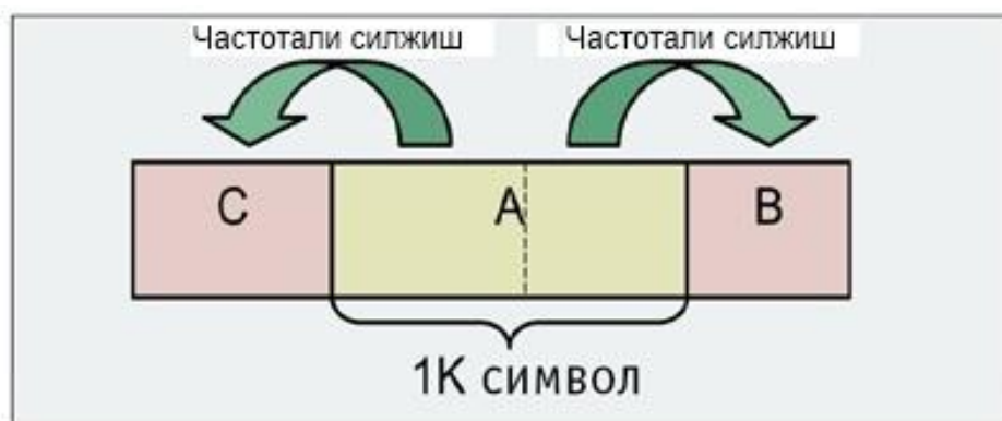
5.9-расм. DVB-T2 сигнализацияси P1 символининг соддалаштирилган кўриниши
