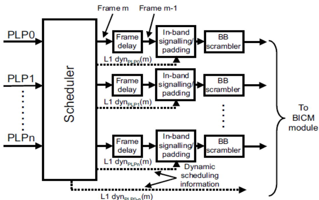
5.5.расм. DVB-T2 тизими маълумотлар оқимиға мослашиш блоки
