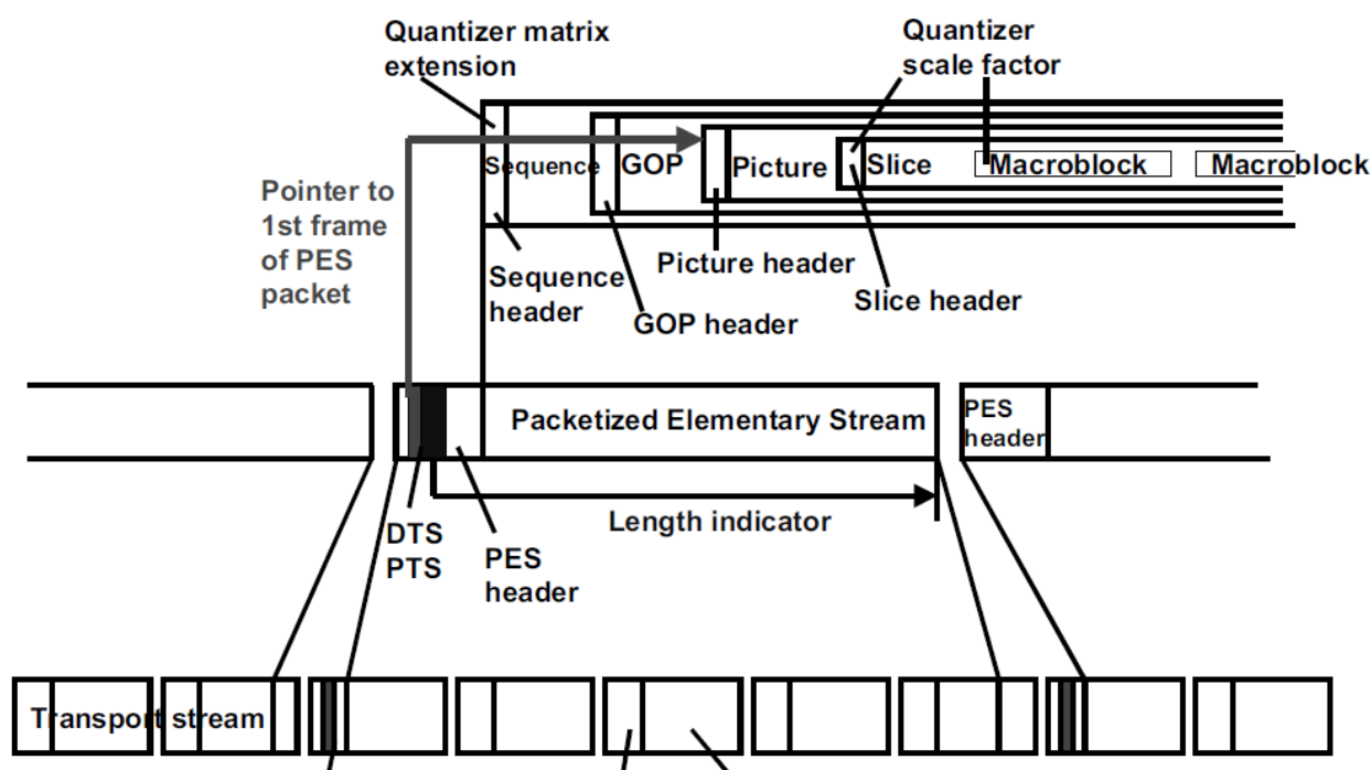
3.14.расм. МРЕG-2 маълумотлар оқими структураси
