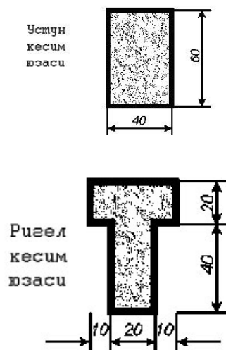
2-расм. Рама элементлари кесимлари
