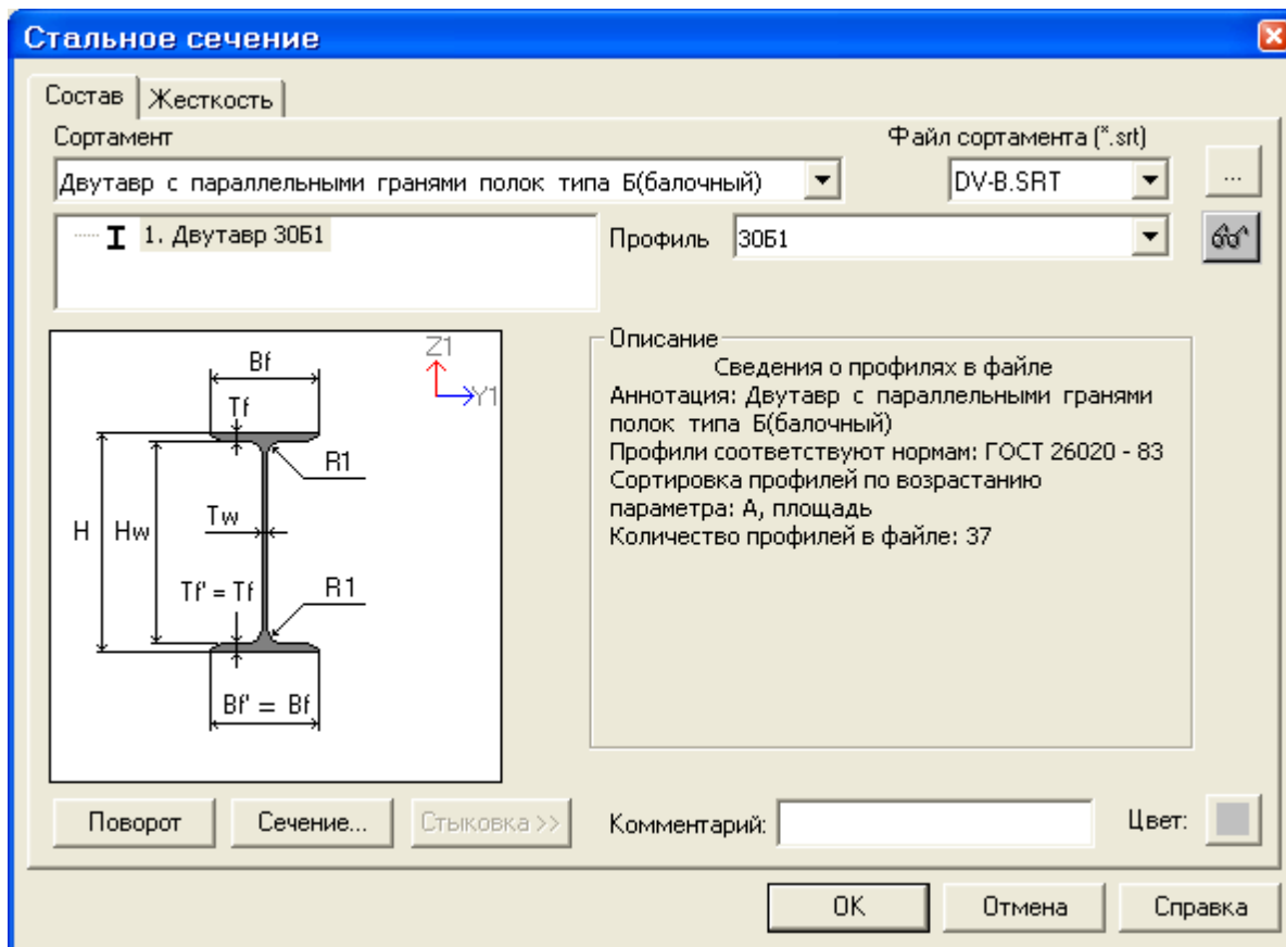
12-расм. Пулат кесим юзалар мулоқот ойнаси
