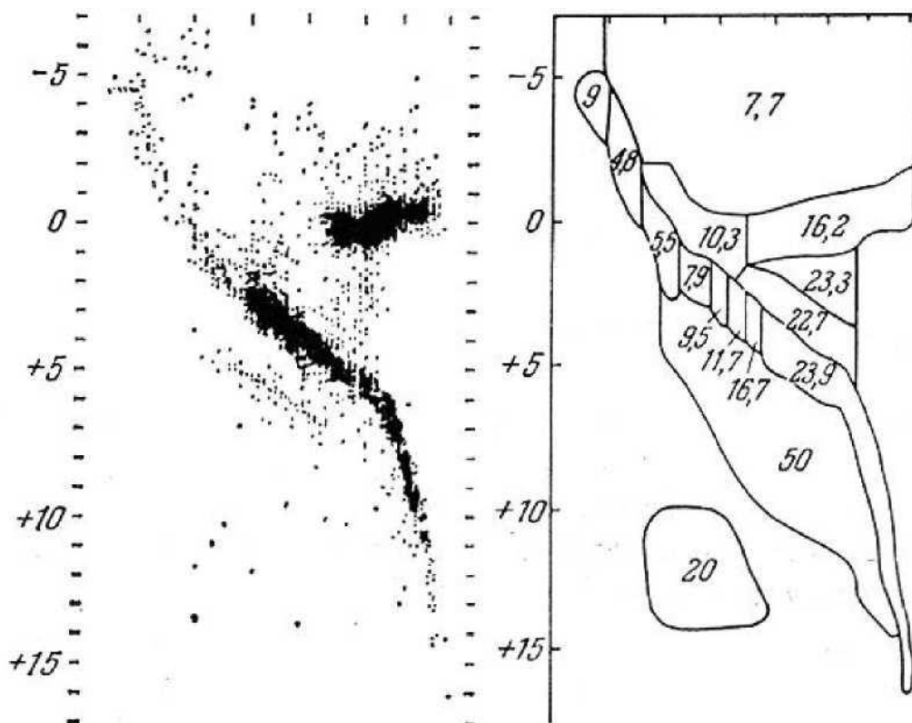
2-rasm-7. Gershprung-Rassel diagrammasi va ayrim yulduzlar guruhlarining fazoviy xarakteristik tezliklari
