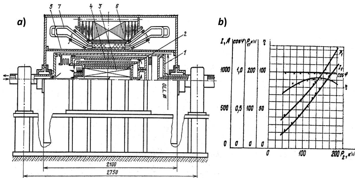
2-rasm. Quvvati 1200 kW, 3000 ayl/min bo'lgan o'ta o'tkazgich qo'zg'atish chulg'amli turbogenerator (a): 1 – rotor; 2 – qo'zg'atish g'altagi ( 3 ) ni siqib turuvchi rotor bandaji (kamari); 4 – ekran; 5 – shisha plastikdan tayyorlangan vacuum idishi; 6 – elektrotexnik po'lat plastinalaridan yig'ilgan stator; 7 – mis o'tkazgichning ichidan suv bilan sovutiladigan stator chulg'ami; b – quvvati 200 kW, 3000 ayl/min bo'lgan o'ta o'tkazgich qo'zg'atish chulg'amli turbogeneratorning yuklama bilan ishlashidagi xarakteristikasi
