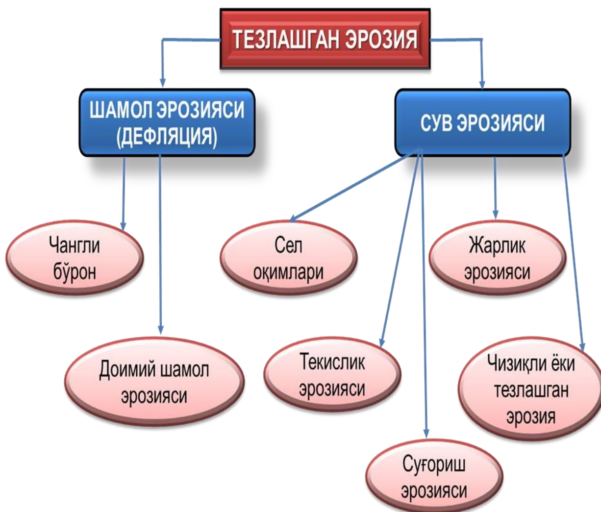
3- rasm. Tuproq degradatsiyasini tezlashtiruvchi omillar (Degradasiya i oхрана почв, 2002).
