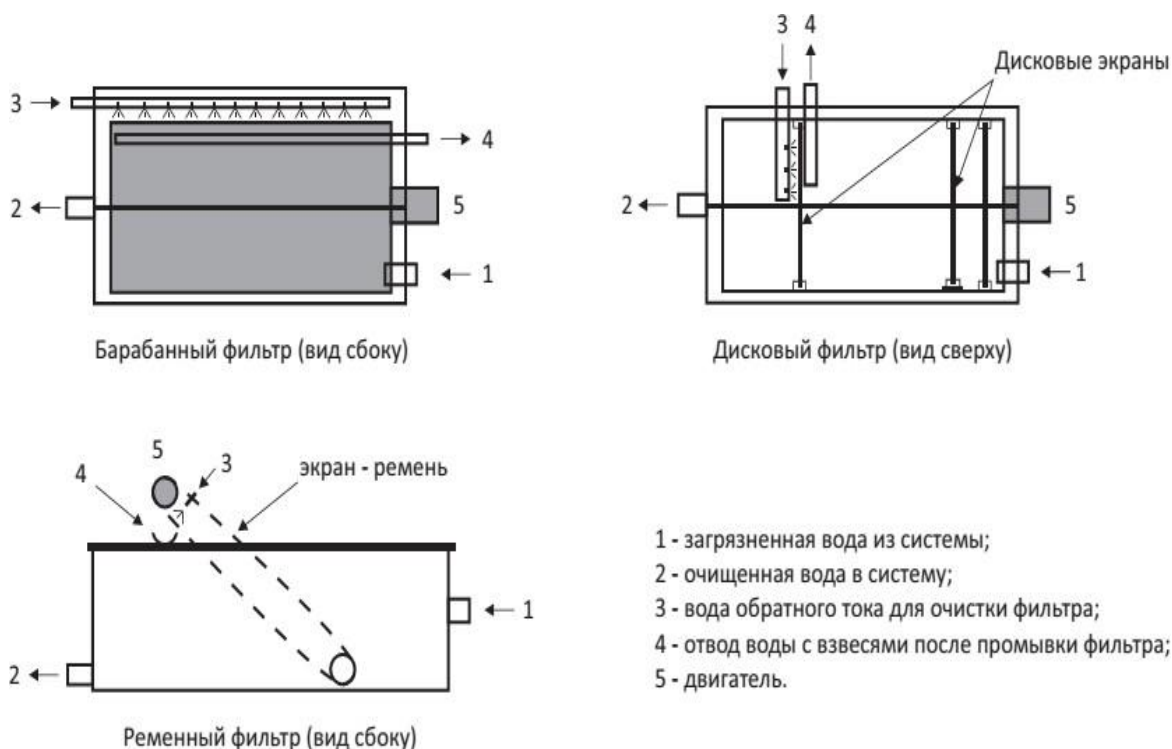
47-rasm. Ekranli mexanik filtrlar chizmasi.
