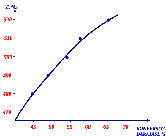
1.4-rasm. Dixloretnan konversiya darajasining jarayon haroratiga bog‘liqlik grafigi
