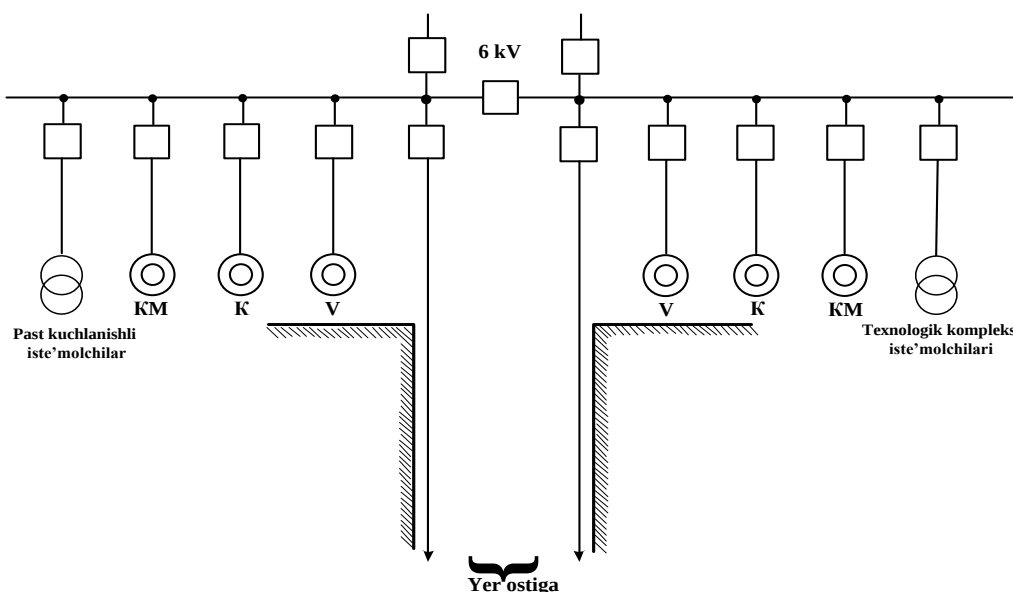
2.1–rasm. Yer usti iste'molchilarining elektr ta'minoti sxemasi
