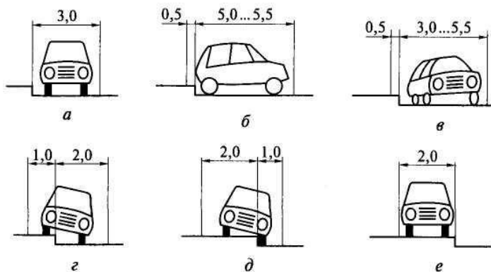
16-rasm. Yo'llarda avtoturargohlarni joylashtirish:
