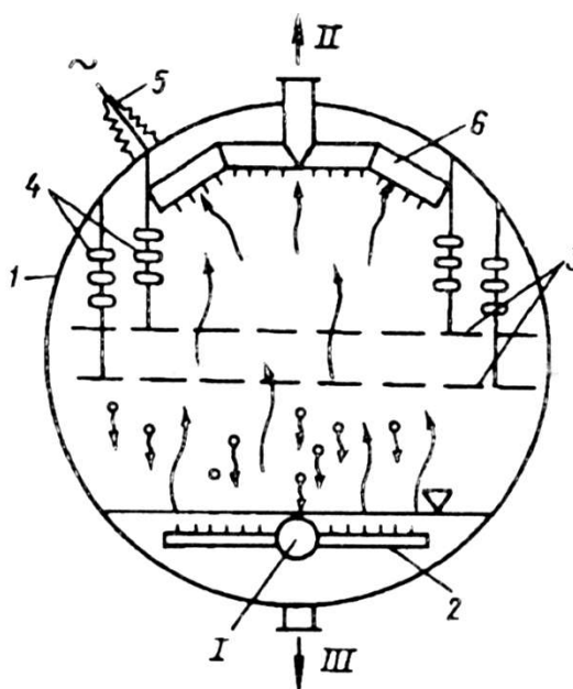
2.9 –Rasm. 2EG – 160 (ko'ndalang kesim) elektrodegidratorni tuzilishi sxemasi:
