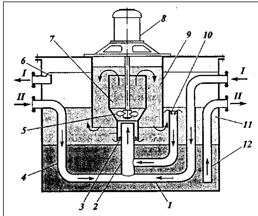
15.8 – rasm. Aralashtirigich – tindirgich rusumidagi ekstraktorning sxemasi:
