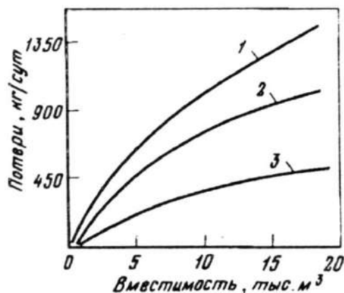
2.12-rasm. Turli sig'imli rezervuarlarda «kichik nafas» da bug'larning yo'qotilishi 1-engil benzin; 2-benzin; 3-neft.
