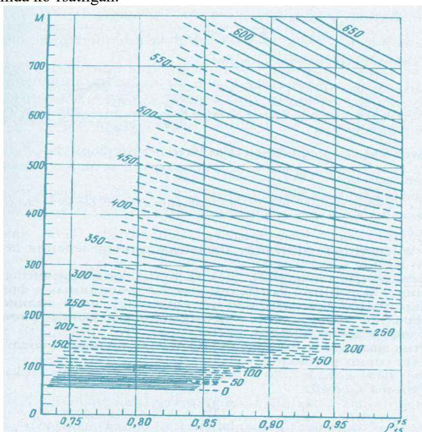
14-rasm. Neft mahsulotlari va ular fraksiyalari o‘rtacha molekulyar massasi M_{ni} aniqlash grafigi (egri chiziqdagi raqamlar– fraksiyalarning o‘rtacha qaynash harorati, ^{\circ}\text{C} ).
