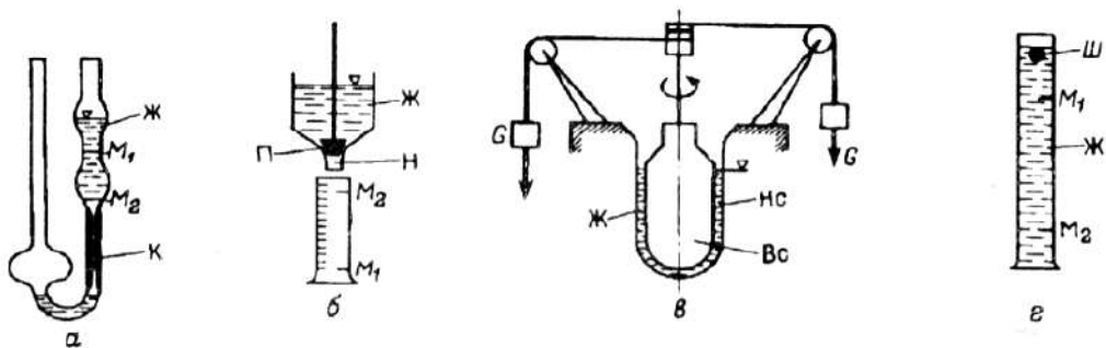
15-rasm. Suyuq neft mahsulotlarining qovushqoqligini aniqlash usullari
