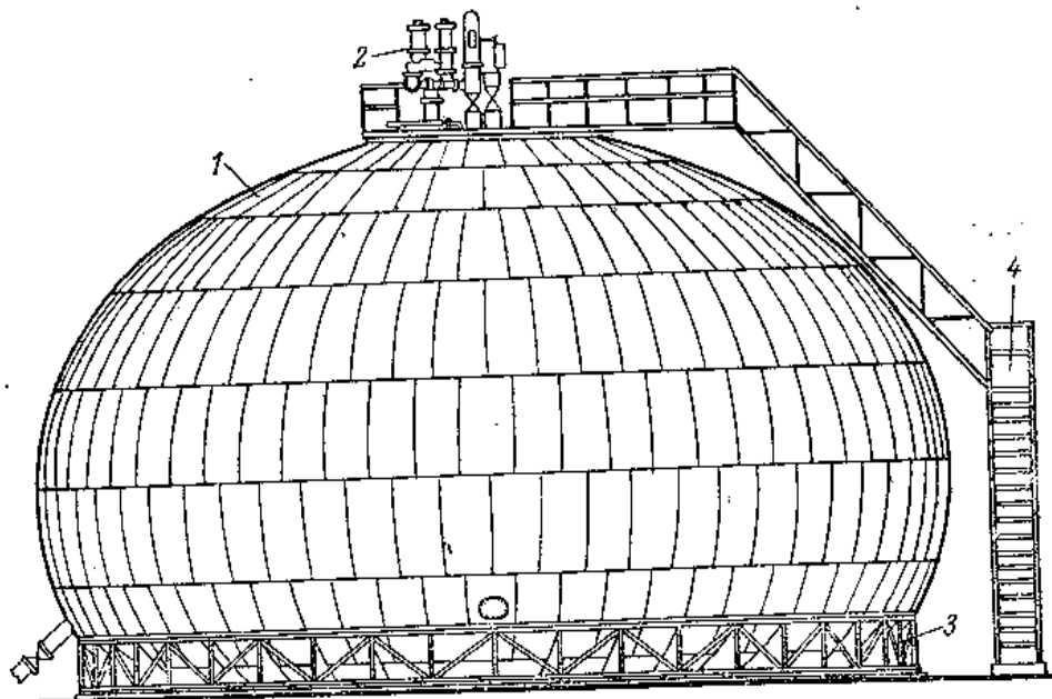
3-rasm. Tomchi ko‘rinishdagi rezervuar 1-rezervuar korpusi; 2-imoyalovchi urilmalar; 3-rezervuar tayanchi; 4-xizmat ko‘rsatish narvoni.
