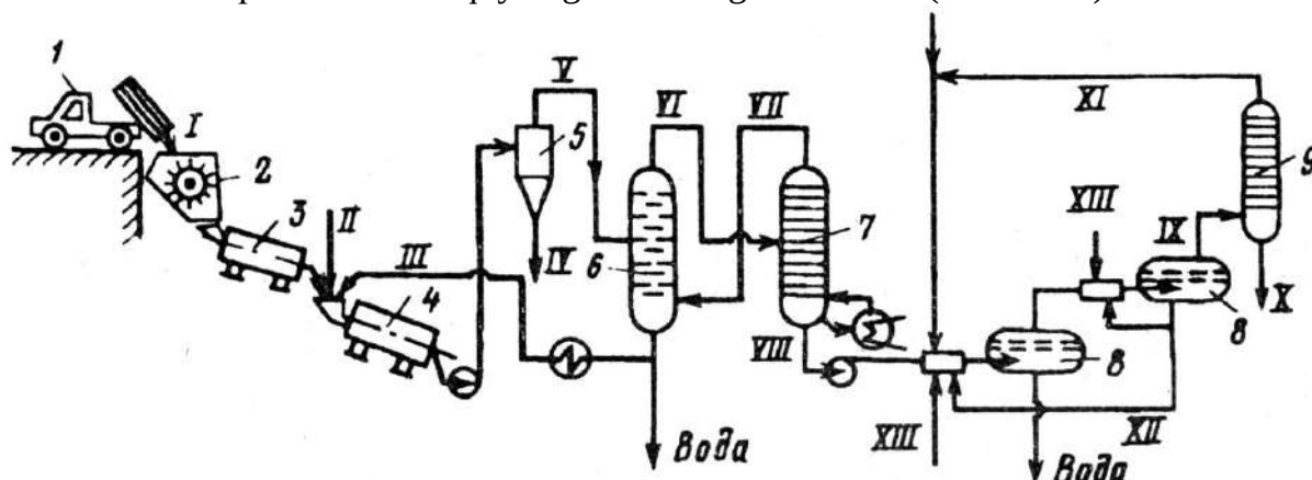
2.11-Rasm. Bitumsimon jinsni qayta ishlashga tayyorlash sxemasi.
