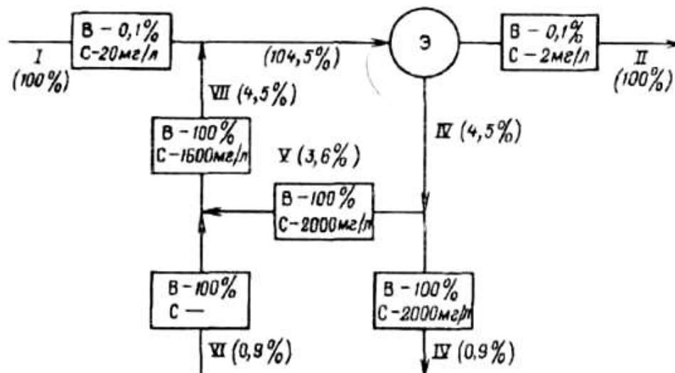
2.6-rasm. Neftning suvni retsirkulyasiyalı yuvish sxemasi va suv bo'yicha tuzli balansi.
