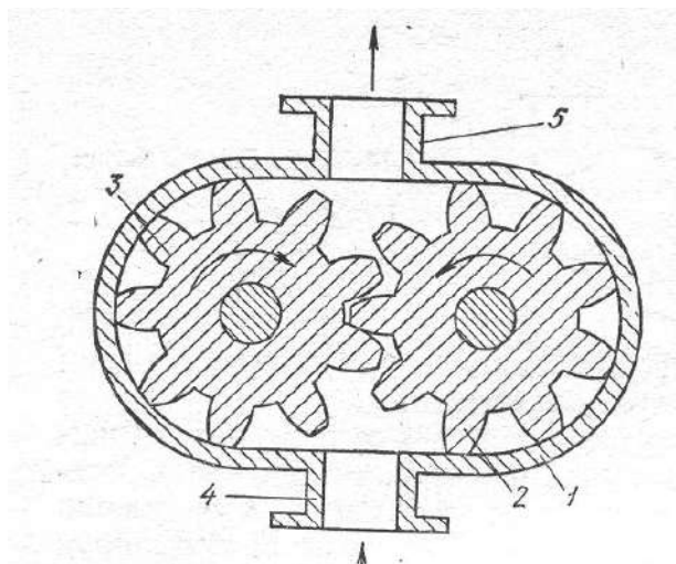
3 – расм. Шестерняли насос. 1 – қобик; 2,3 – бир бирига илашган тишли шестернялар; 4 – сўрувчи потрубка; 5 – узатувчи потрубка.
