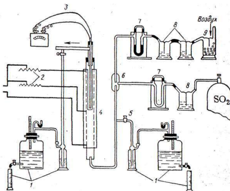
Rasm. 5. Osm katalizatorli qatlamda SO_2 ni oksidlash uchun o'rnatish: 1—Reyx qurilmasi; 2 — reostat; 3—pirometr; 4 pinli qurilma; 5—gazdan namuna olish klapan; 6 - aralashtirgich; 7— reometr; 8— H_2SO_4 solingan shisha
