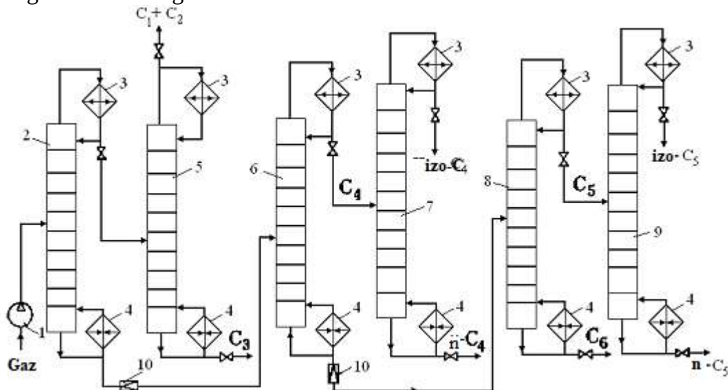
4-rasm. C_1 - C_5 uglevodorodlarini ajratish texnologik sxemasi:
