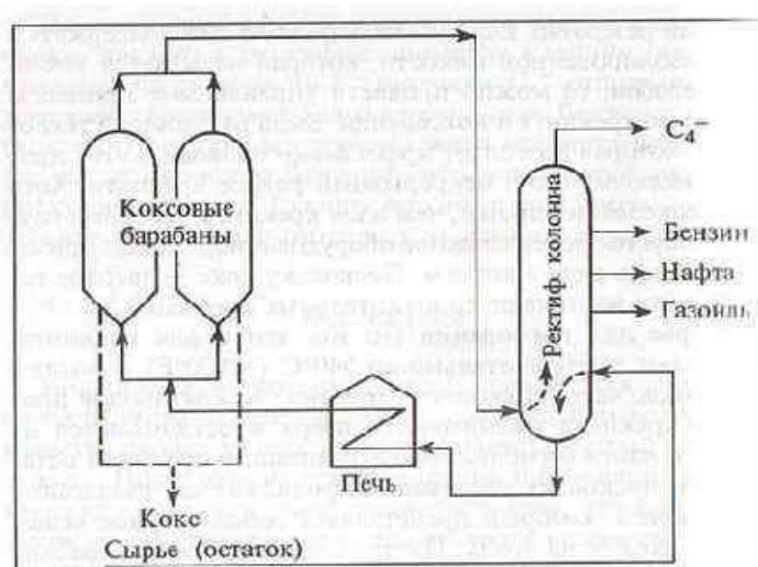
Рис. 10.3. Коксование.
