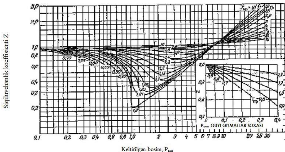
21-rasm. Siqiluvchanlik koeffitsiyenti Z ni aniqlash grafigi
