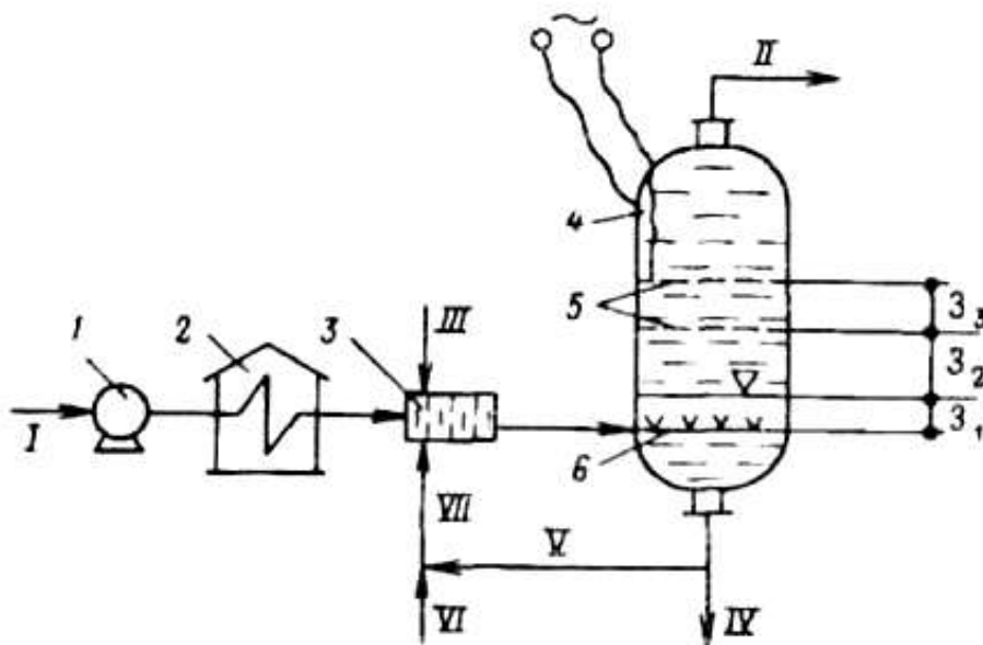
2.5-rasm. Neftni elektrotermokimyoviy suvsizlantirish va tuzsizlantirish sxemasi.
