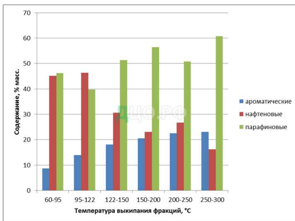
13-rasm - Uglevodorodlar tarkibining turli fraksiyalarga bog'liqligi
