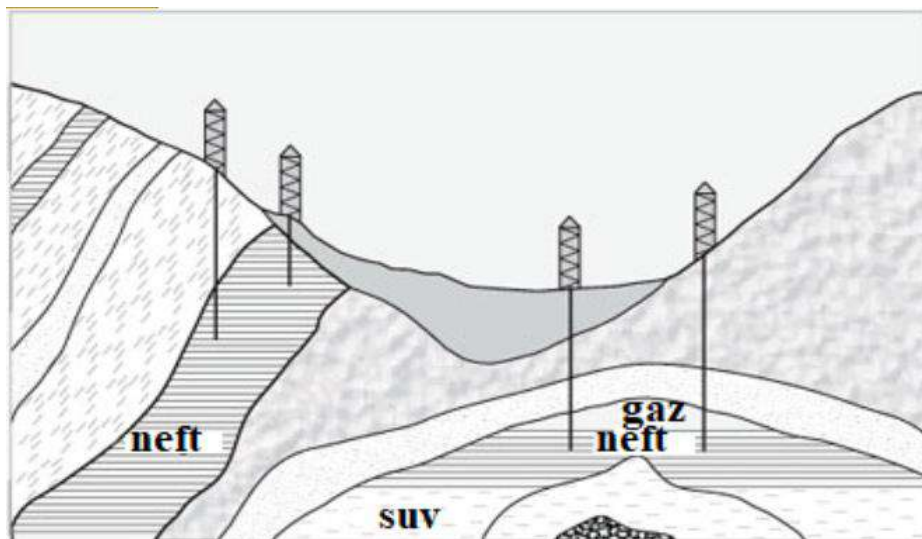
Rasm.5. Neftli hududning geologik kesimi
