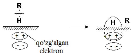
19-rasm. Uglevodorod molekularining yuzasidagi erkin elektronlar (tuynuk)lar o'zaro ta'siri
