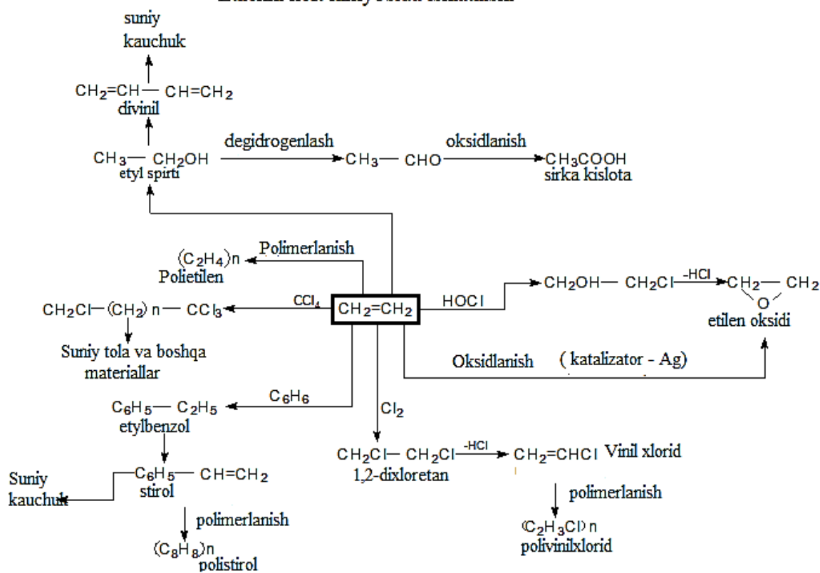
72-rasm. Etilenning neftkimyo sintezda islatilishi
