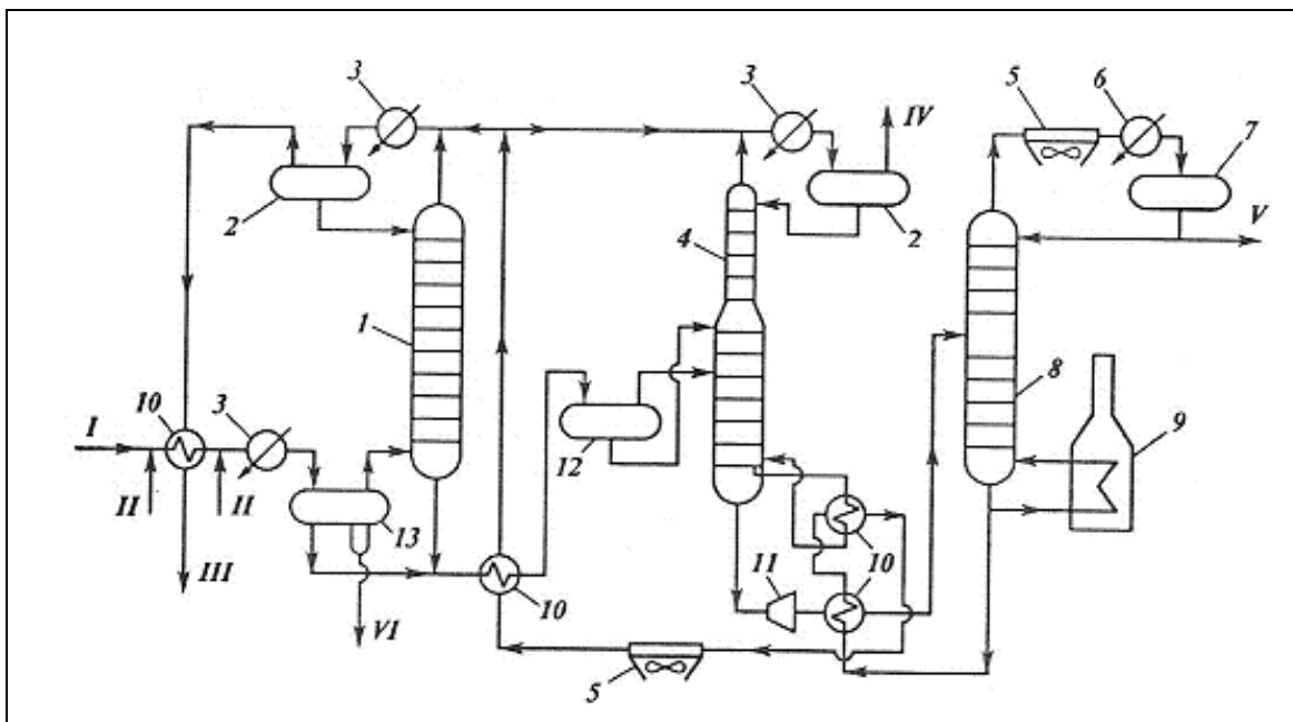
12.6-rasm. Tabiiy va neftga yoʻldosh gazlarni ajratishga moʻljallangan absorbsion - desorbsion qurilmaning sxemasi:
