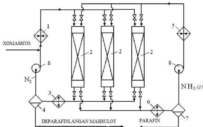
5-rasm. Pareks usuli bilan n-parafinlarni ajratish texnologik sxemasi:
