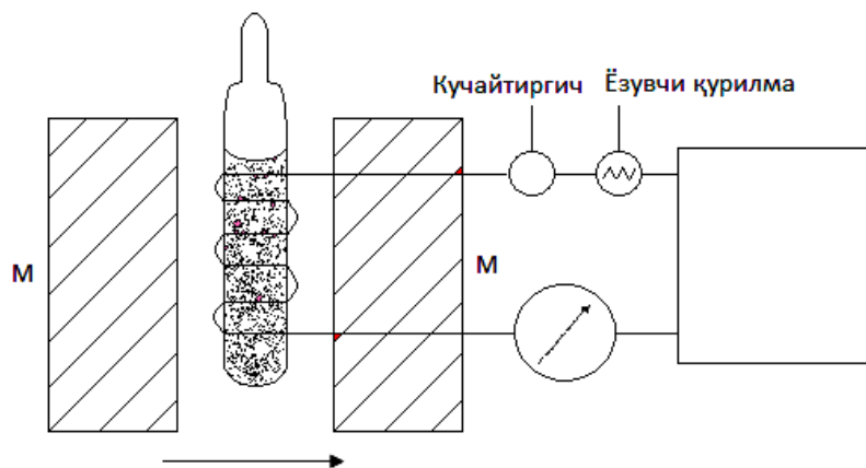
9-rasm. YaMR– spektmetrining umumiy ko’rinishi
