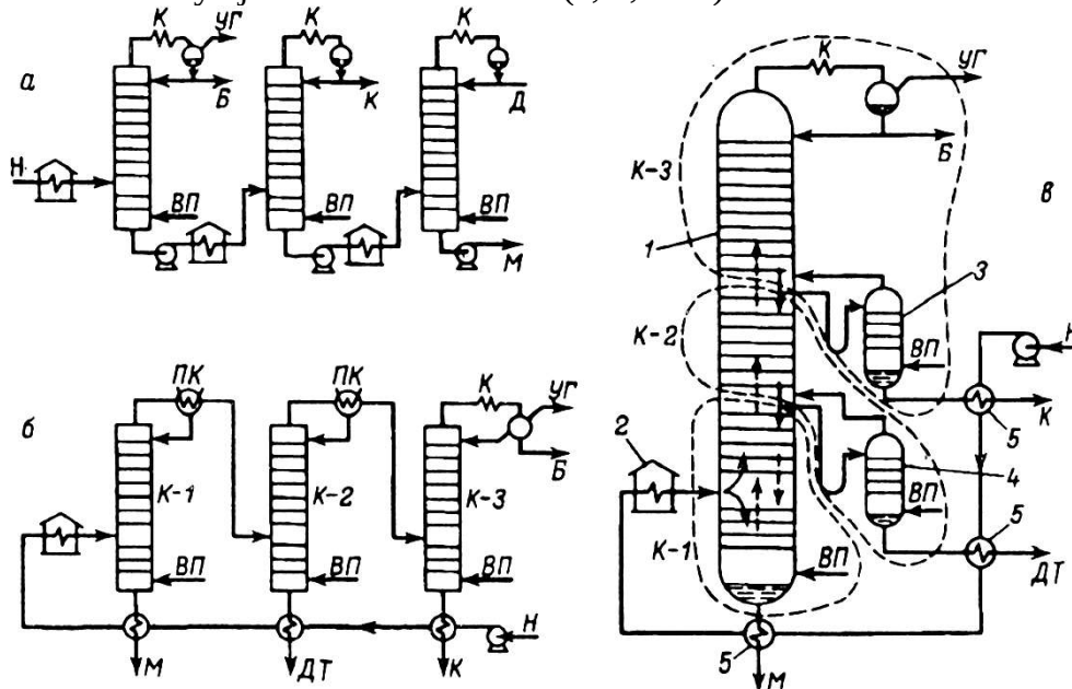
2.21-rasm. Neft (n)ni uch distillat (B, K, DK) va qoldiq (M) ga neftni uchkarra bug‘latish (a), uning bug‘larini uchkarra kondensatsiyalab (b) va bir butun kolonna (v) da reksifikatsiyalash prinsipial sxemasi.
