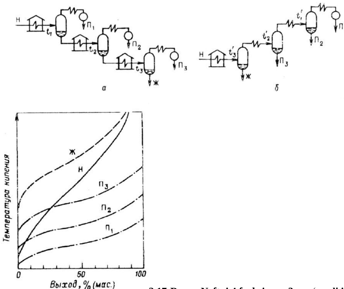
2.17-Rasm. Neftni 4 fraksiyaga 3-pog‘onali isitish (a) va 3-pog‘onali (b) kondensatsiyalab ajratish prinsiplari. havfli belgilashlar bo‘yicha – 2.16-rasmlarga qarang.
