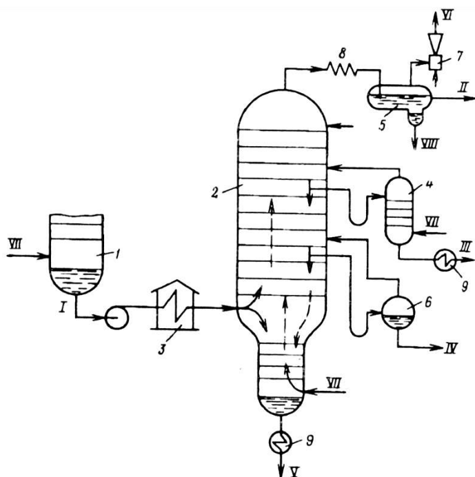
2.22-Rasm. Mazut vakuumda reksifikatsiyalash prinsipial sxemasi.
