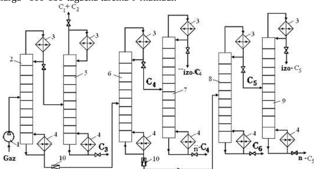
4-rasm. C_1 - C_5 uglevodorodlarini ajratish texnologik sxemasi:
