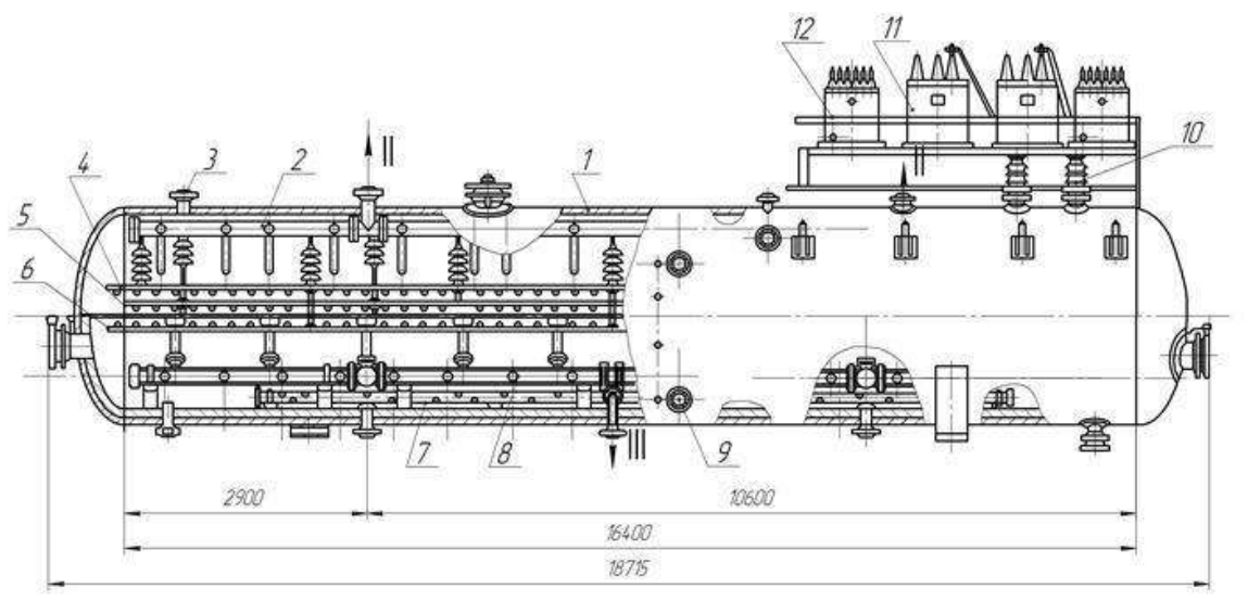
Горизонтал электр қуритгич 2EG 160-2:
