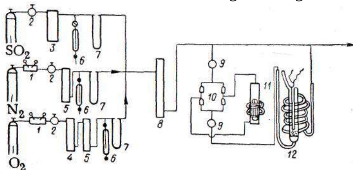
Rasm. 4. SO_2 oksidlanish uchun oqim-sirkulyatsiya birligi : 1—reduktor; 2— nozik sozlash klapan; 3 - H_2SO_4 bilan pufakchalar ; 4— CuO li ustun ; 5—angidronli ustun; 6—
