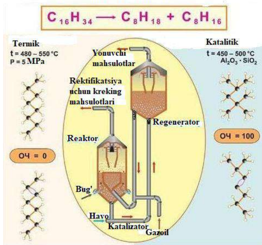
Rasm.9 Neft mahsulotlarining krekingi
