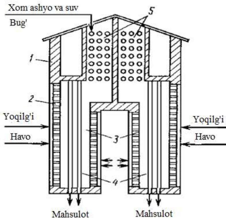
6-rasm. Piroliz pechining sxemasi: 1-korpus; 2-panel gorelkalar; 3-radiant kameralar; 4-vertikal quvurlar; 5-koveksion kamera.
