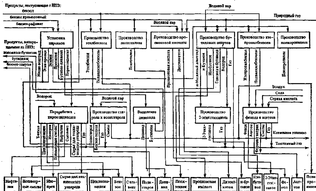
Shakl: 2.4. NHZ oqim sxemasi.
