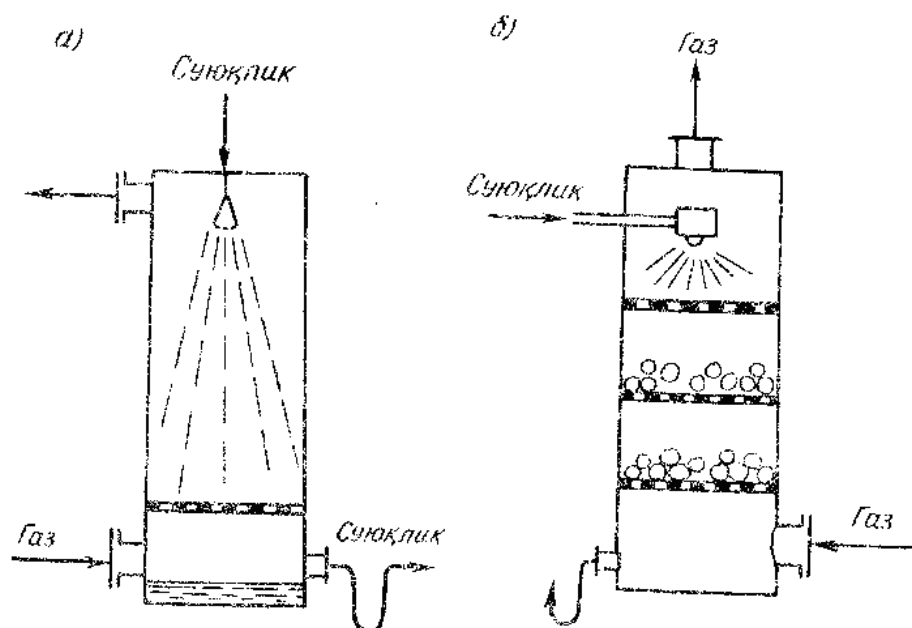
42-rasm. Suyuqlikni sochib beruvchi absorberlar
