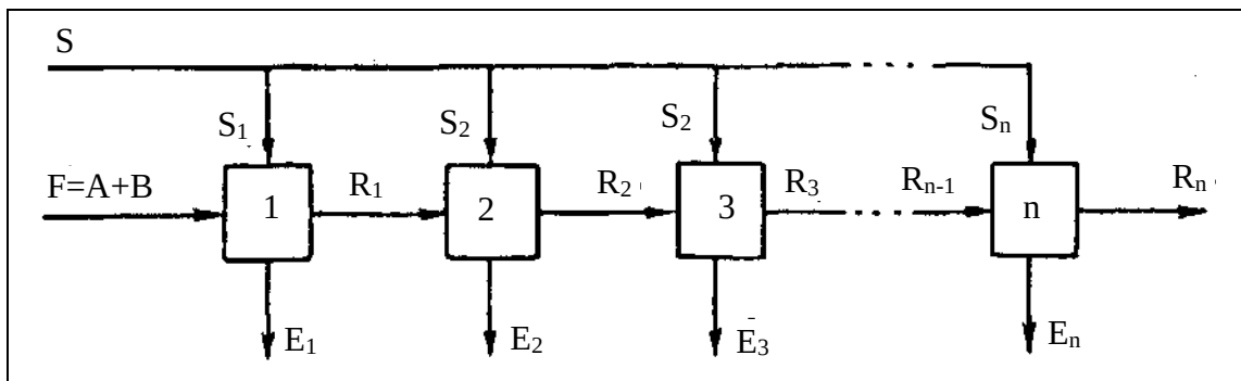
15.6-rasm. Ko'p pog'onali va erituvchini paralel ravishda ishlatishga asoslangan ekstraksiyalashning sxemasi:
