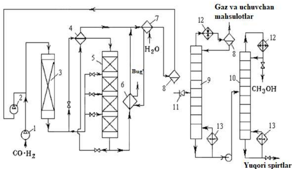
60-rasm. Metanol sintez qilish texnologik sxemasi:
