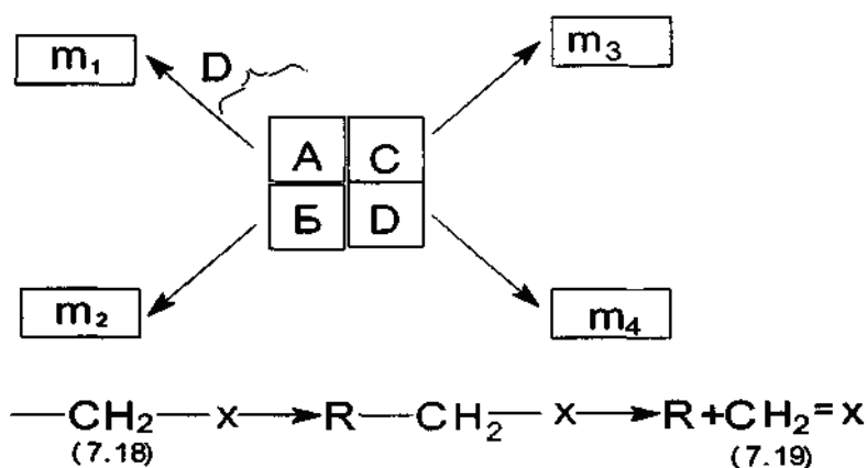
12-rasm. Spekrda kuzatiladigan ionlar
