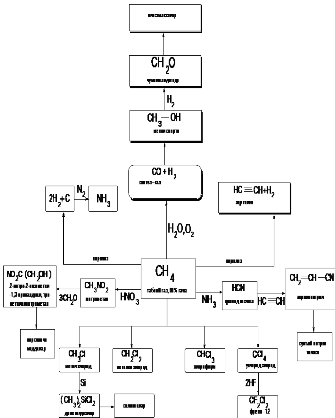
3.1-rasm– Neft kimyosi sanoatida metanni ishlatilish sohalari
