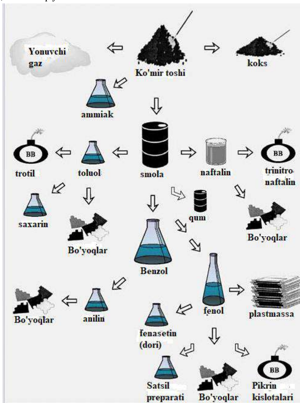
Rasm.10. Ko'mir va uning mahsulotlarini quruq distillash
