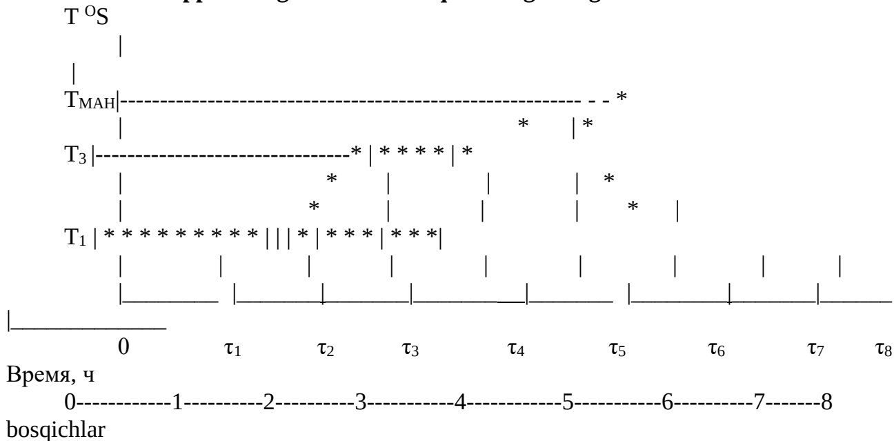
Shakl 2. Apparatdagi moddalar miqdorining siklogrammasi.
