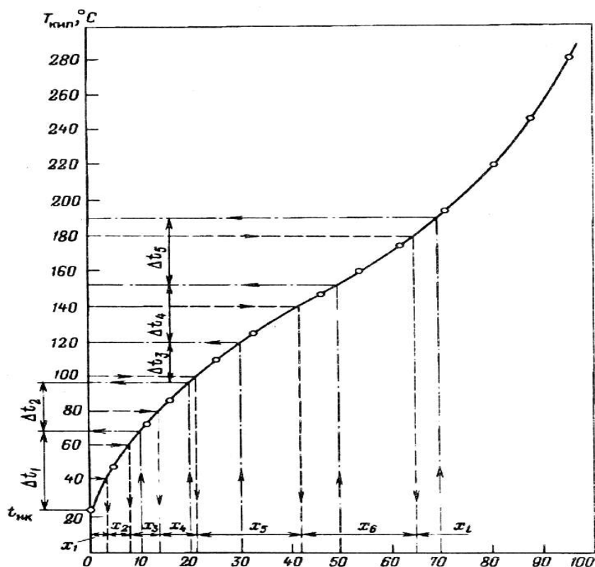
12-rasm. HQH egri chizig'ini shartli komponentlar bilan ko'rsatilishi (0–tajribaviy nuqtalar; punktir–qaynash harorati shkalasi bo'yicha tor fraksiyalarga bo'lish; shtrix-punktir–fraksiyalarni chiqish miqdori bo'yicha tor fraksiyalarga bo'lish).
