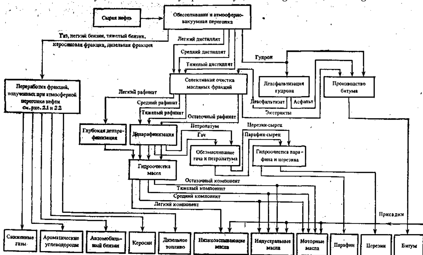
Shakl 2.3. Yoqilg'i-moy profilidagi neftni qayta ishlash zavodining oqim sxemasi.
