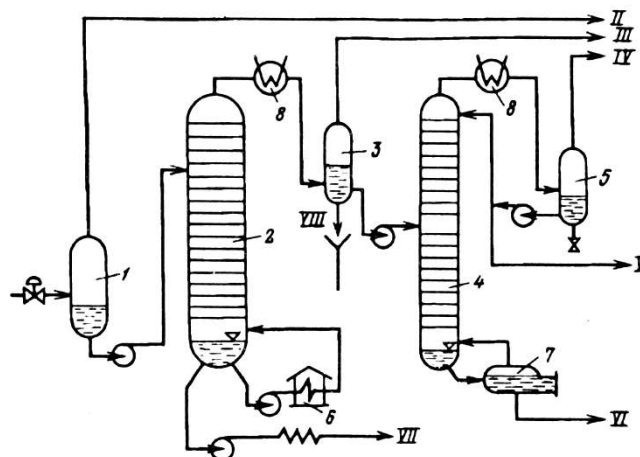
2.14-Rasm. Neftni ikki pog'onali barqarorlashtirish qurilmasi prinsipial sxemasi.
