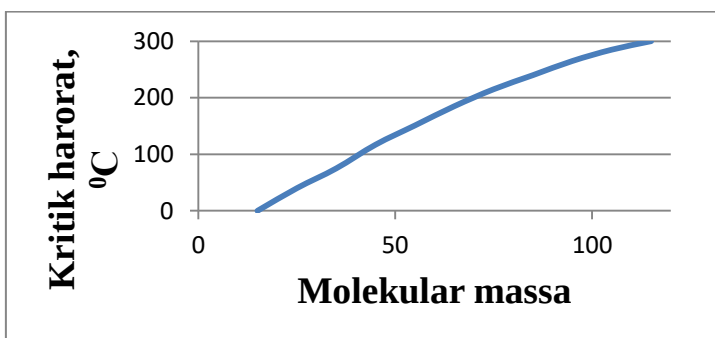
16-rasm. Gazlarning kritik haroratini aniqlash grafigi
