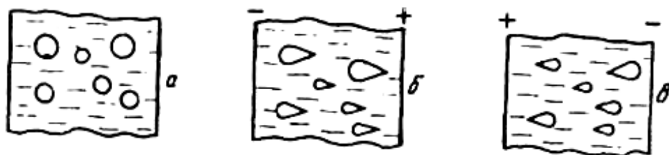
2.4-rasm. Elektr maydonni emulsiyaga ta’sir etish sxemasi.
