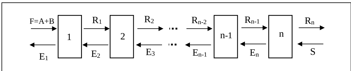
15.7-rasm. Ko'p pog'onali va qarama-qarshi oqimli ekstraksiyalashning sxemasi:
