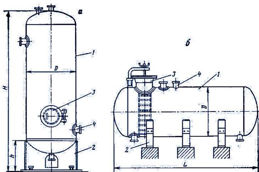
1.1-rasm. Suyuqltirilgan gazlar va engil benzin fraksiyalarini saqlash idishlari a-vertikal; b-gorizonta; 1-korpus; 2-tayanch; 3-lyuk; 4- shtusterlar.
