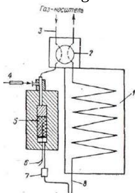
расм. 6. Пулси каталитик микрореактор:
