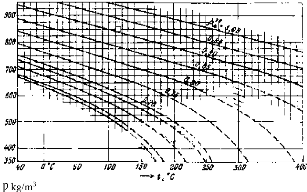
13-rasm. Neft mahsulotlari zichligining haroratga t ga bog'liqligi (egri chiziqdagi raqamlar – nisbiy zichlik \rho_4^{20} )
