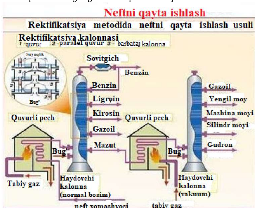
Rasm.7.Rektifikatsiya usulida neftni qayta ishlash.
