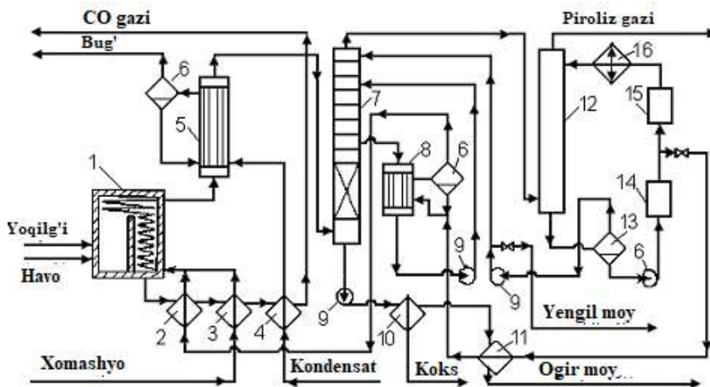
7-rasm. Benzinni piroliz qilish texnologik sxemasi:
