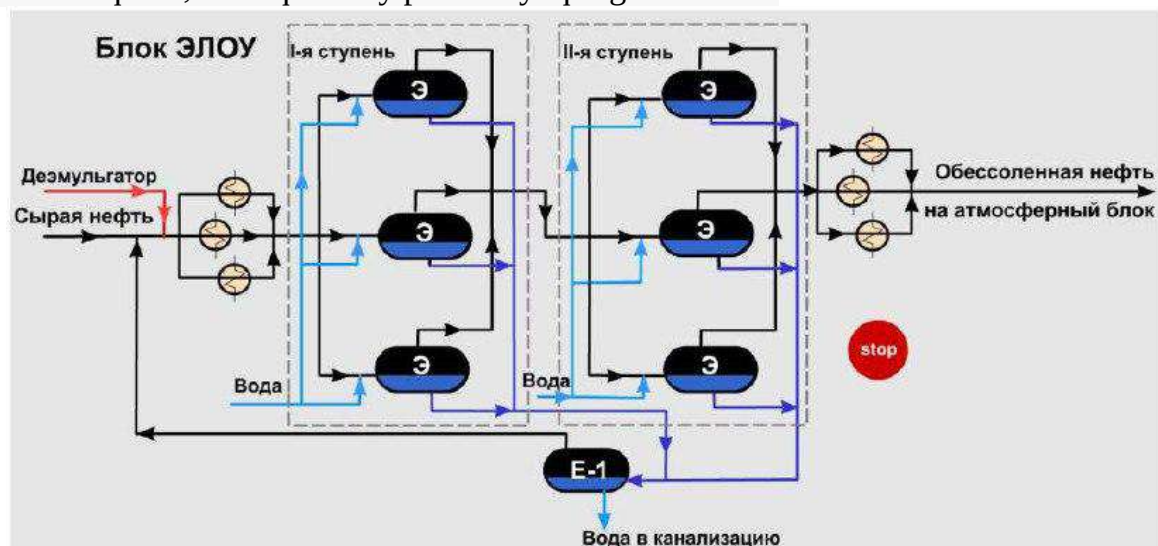
Горизонтал электр қуритгичлар билан ELOU sxemasi
