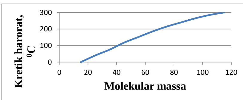
17-rasm. Gazlarning kritik bosimini aniqlash grafigi
