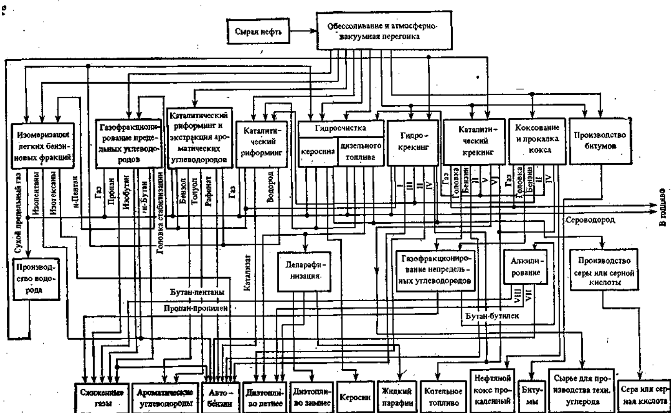
Shakl 2.2. Neftni chuqur qayta ishlash bilan yoqilg'i profilidagi neftni qayta ishlash zavodining oqim sxemasi:
