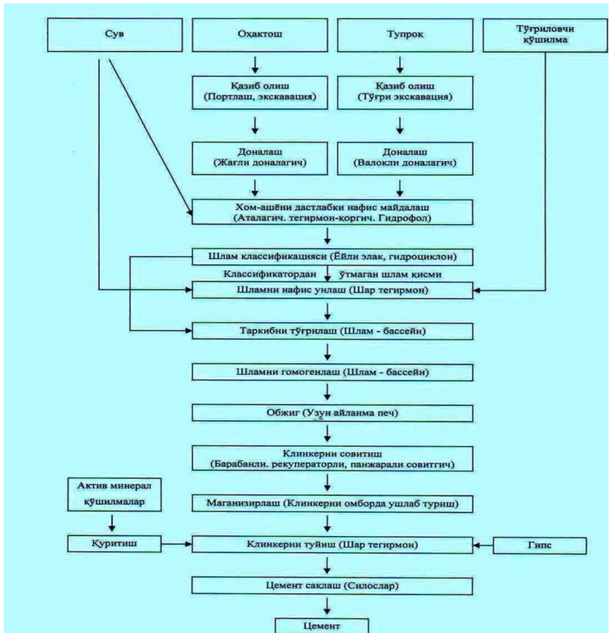
5.13- rasm. Portland sementni «xo'l» usulida ishlab chiqarish texnologik tizimi.
