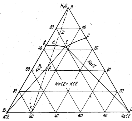
Рис. 5. Изотерма растворимости в системе \text{NaCl}-\text{KCl}-\text{H}_2\text{O} при 100^\circ\text{C}
