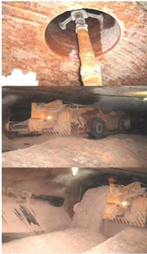
2-3-расм. Тўбетатан калийли маданларнинг жойлашсини ва уни казиб олиш жараёнлари.
