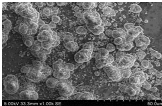
6-Rasm B. Amin qatlamini natriy metasilikati bilan ishlanganidan so'ng mikrofotografiyasi T=25^{\circ}\text{C} (SEM, 1000X kattalashtirish)
