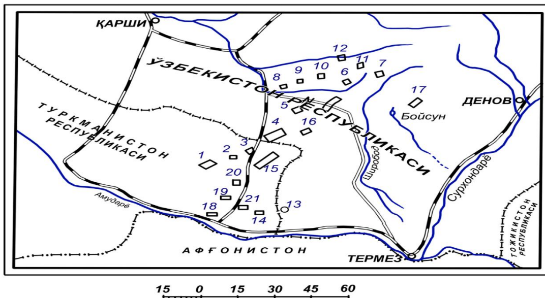
8-rasm. Janubiy-gʻarbiy Hisor togʻ tizmalari boʻyicha kaliyli tuz konlarining joylashishi.
