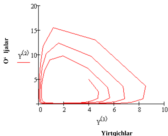
9.8-rasm. 9.7-rasmning fazali tasviri.
