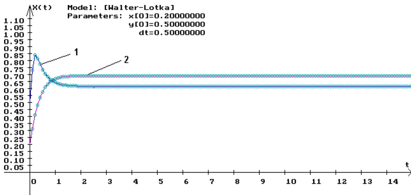
9.9-rasm. Volter-Lotka diskret modelining x_0=0,2 , y_0=0,5 , \Delta t=0,5 dagi hatti-harakati ( 1 - y(t) ; 2 - x(t) ) egri chiziqlar. Bu erda va kelgusida r_x = r_y = 1 , y^* = 1,1 , \mu_x = 0,5 , \square_y = 0,7 deb olinadi).
