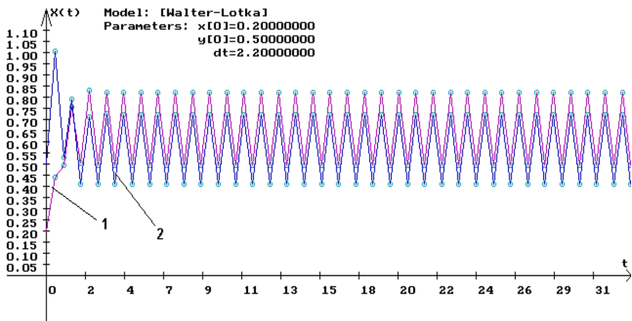
9.11-rasm. Volter-Lotka diskret modelining x_0=0,2 , y_0=0,5 , \Delta t=2,2 dagi hatti-harakati (1 – x(t) ; 2 – y(t) egri chiziqlar).
