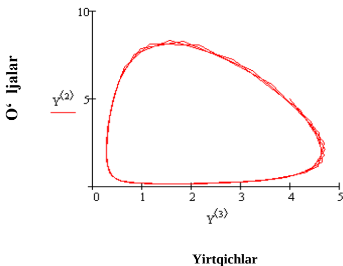
9.2-rasm. Tur ichida raqobat bo'lmagan holda Volter-Lotka modelining evolyusiyasi, yirtqichlarning boshlang'ich soni x_1^0=500 va o'ljalarning soni esa x_2^0=400 , a=4 , b=2,5 , c=2 , d=1 .
