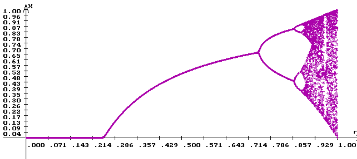
7.14-rasm. r ning har xil qiymatlari (abssissalar o'qi) ga nisbatan katta n larda Ferxyulst-Perl diskret modeli echimining (ordinatalar o'qi) hatti-harakati.
