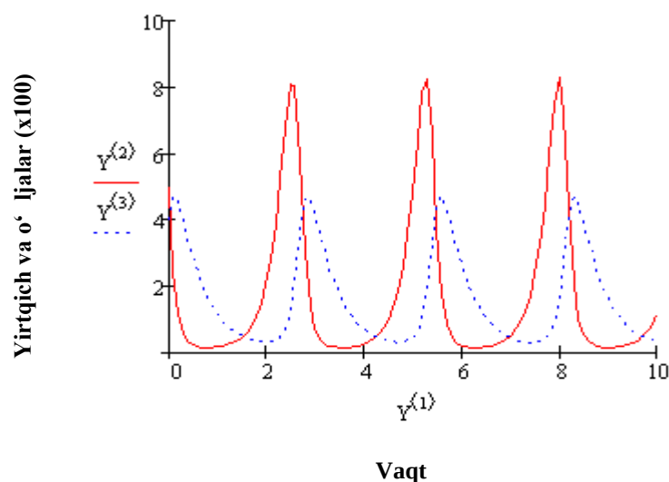
9.2-rasm. Tur ichida raqobat bo'lmagan holda Volter-Lotka modelining evolyusiyasi, yirtqichlarning boshlang'ich soni x_1^0=500 va o'ljalarning soni esa x_2^0=400 , a=4 , b=2,5 , c=2 , d=1 .
