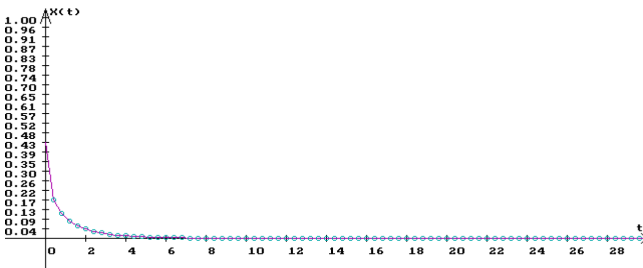
7.10-rasm. Frexyulst-Perl diskret tenglama echimining evolyusiyasi x_0=0,5 , r=0,2 (bu erda va kelgusida: t o'qi bo'yicha qadamlar (2:5 masshtabda), X(t) o'qi bo'yicha esa n -qadamdagi echim ajratilgan).
