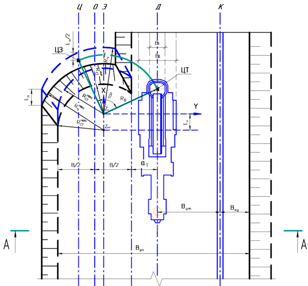
Разрез А-А
