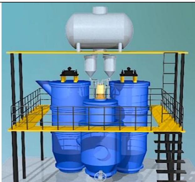
ПЧВ – 300 plazmakimyoviy tiklash qurilmasi.
