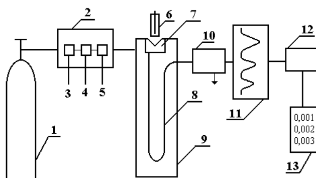
. 1.5- Rasm. Gaz xromatografining blok diagrammasi
