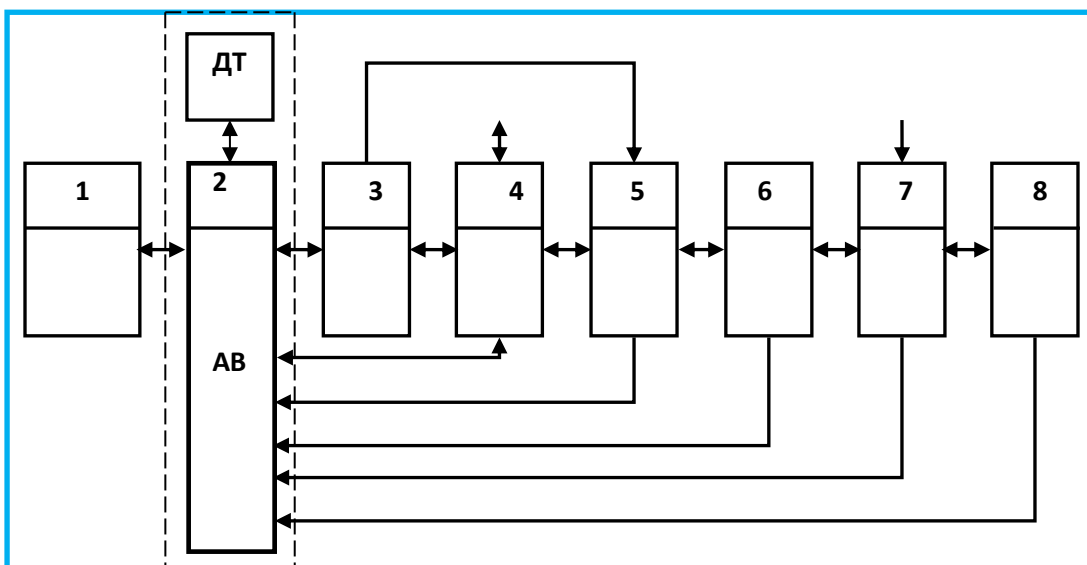
13.3 – rasm. Mikroprocessorli boshqariladigan elektr yuritmaning tarkibiy tuzilishi
