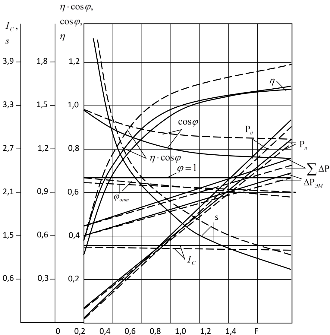
17.4 – rasm. Chastotani o'zgartirib tezligi rostlanadigan elektr yuritmalardagi 4A rusumdagi asinxron motor ko'rsatkichlarining magnet oqimining nominal va optimal qiymatlaridagi chastotaga bog'liq o'zgarish tavsiflari
