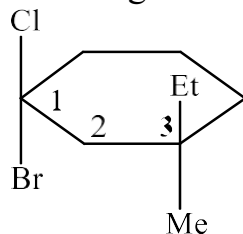
1r-brom-3-metil-1-xlor-3t-etilsiklogeksan
