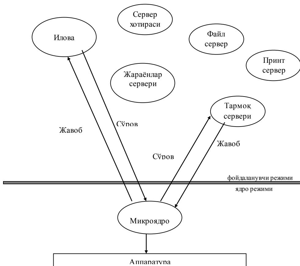
1.4.-расм. ОТ клиент сервер структураси.
