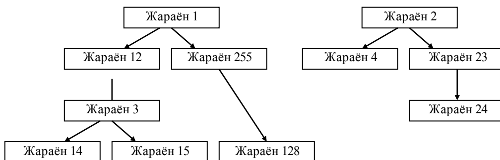
Расм.2.3. содалаштирилган жараёнларнинг ўрмони. Стрелка ота – фарзанд муносабатини кўрсатади.
