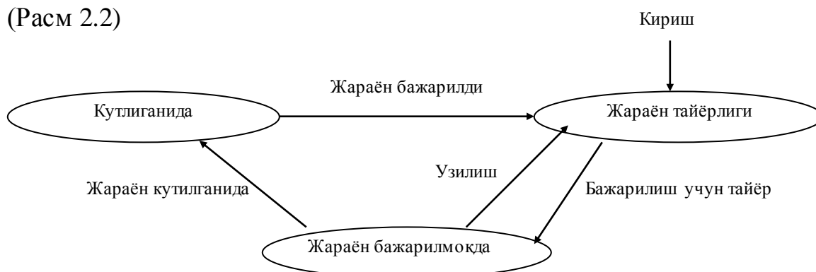
Расм 2.2. Жараён ҳолатининг янада тўлиқ диаграммаси
