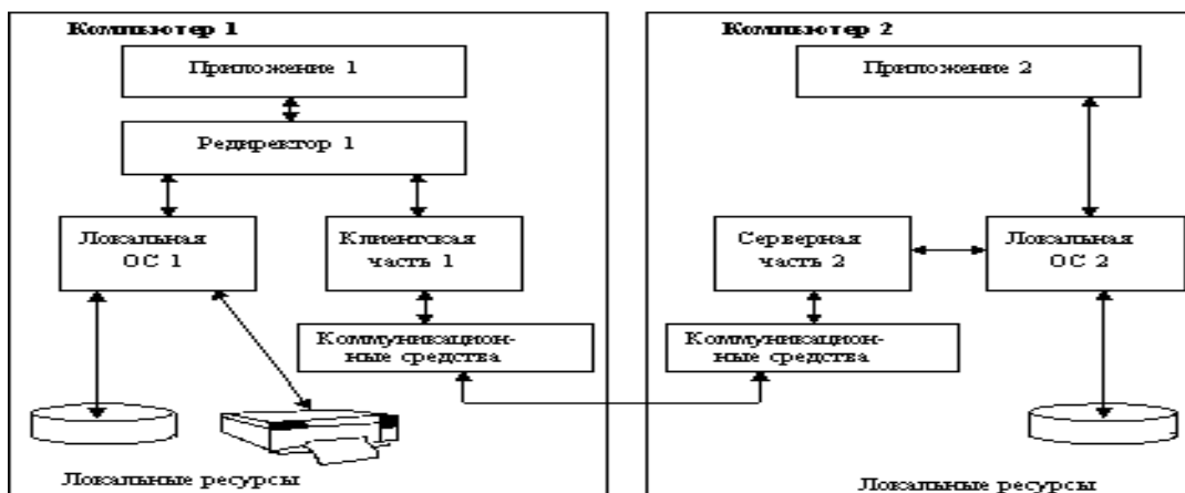
3.2 – расм. компьютерларнинг ўзаро алоқасидаги операцион тизим компонентларининг ўзаро алоқаси.
