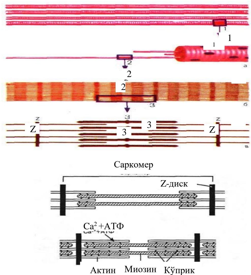
14-rasm. Mushaklarni qisqartirish sxemasi, unda miozin oqsili asosidagi, to'g'ri chiziqli harakatlanuvchi oqsilli motor ishtirok etadi: 1 – mushak tolalari; 2 – mushak tolasining maxsus organoidini fragmenti – miofibrillar; 3 – miozin molekulasi
