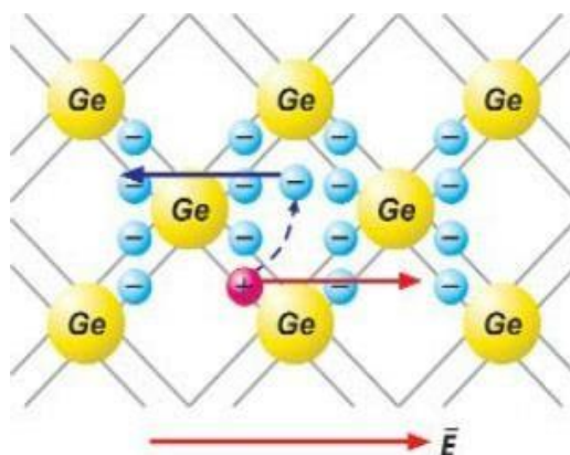
12 – rasm. Germaniy kristalidagi juft elektron bog'lari
