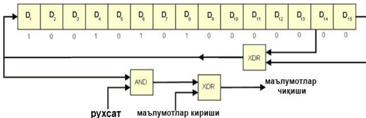
3.6-rasm. Ma'lumotlarni randomizatori
