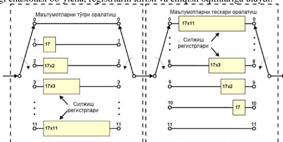
3.8-rasm. Ma’lumotlarni tashqi oralatish
