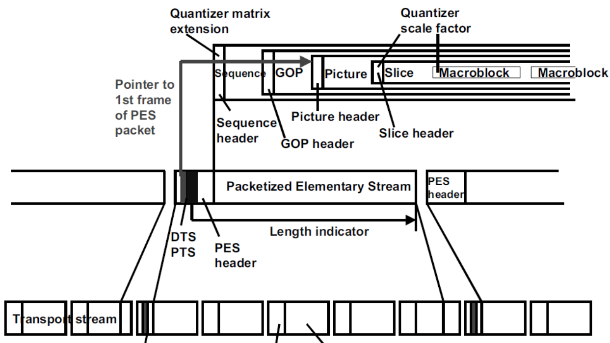
3.14.rasm. MPEG-2 ma'lumotlar oqimi sturkturasi
