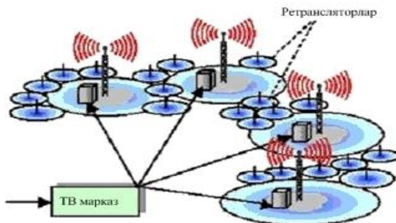
3.12-rasm. DVB-N bir chastotali tarmoq varianti
