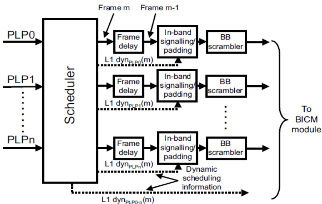
4.5.rasm. DVB-T2 tizimi ma'lumotlar oqimiga moslashish bloki
