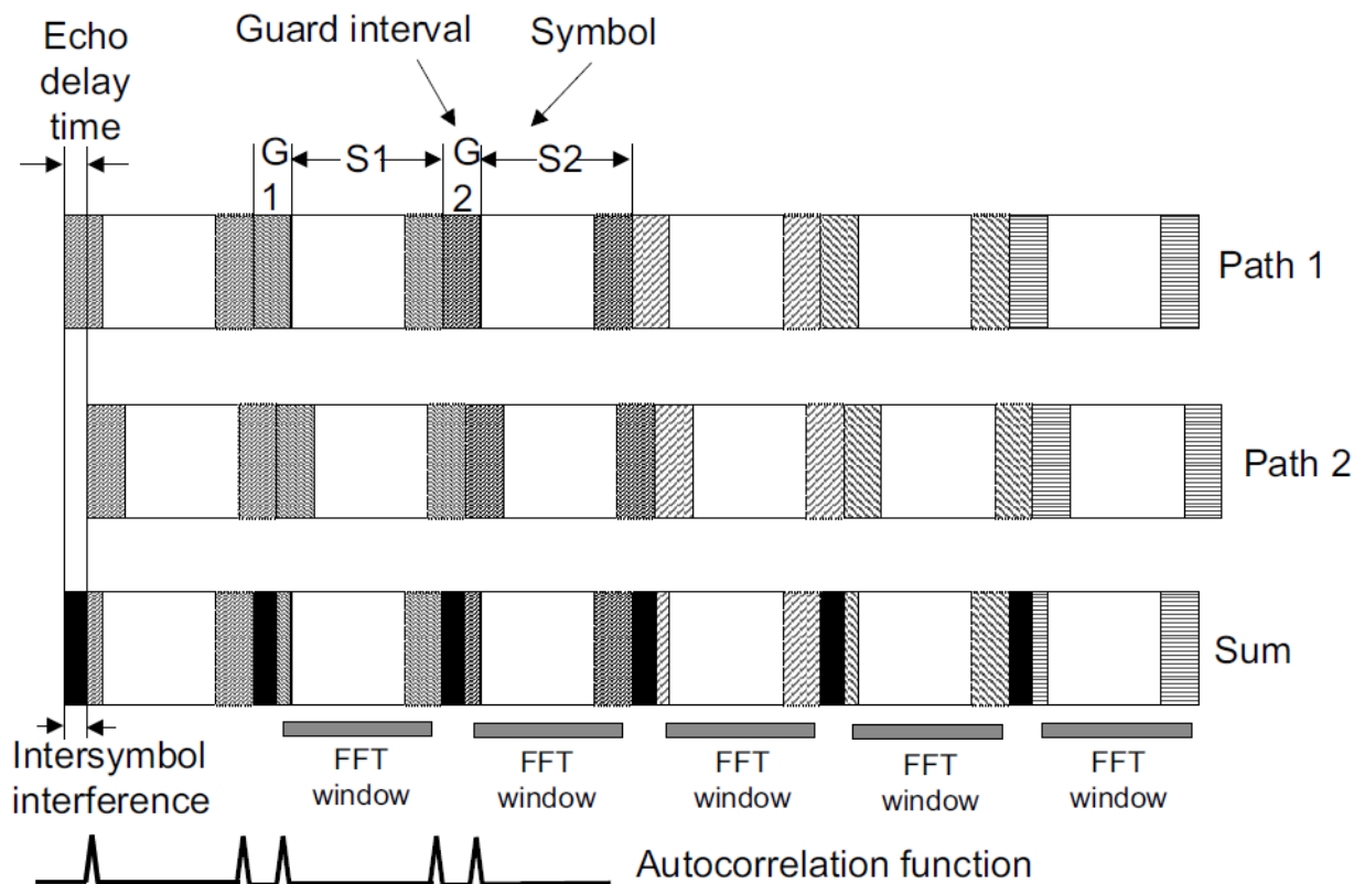
2.19. rasm. OFDM da ko'pnurli qabul qilish
