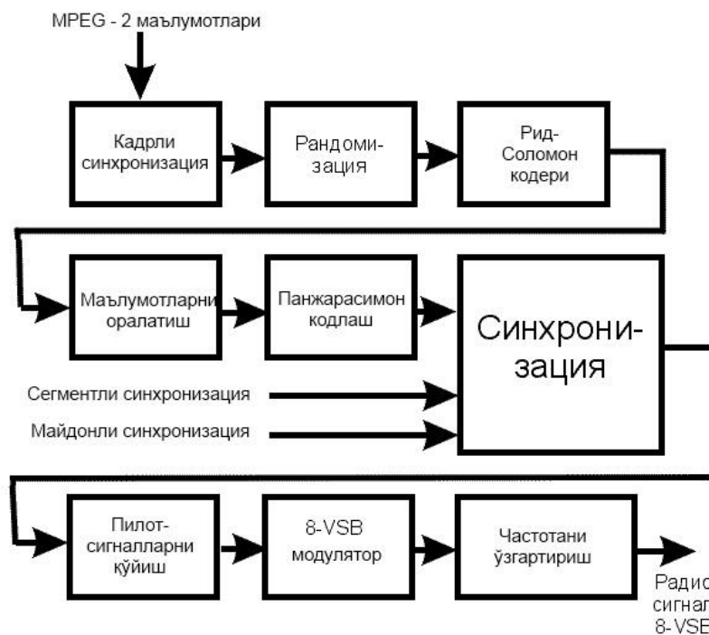
4.15-rasm. ATSC tizimining uzatuvchi qismi tuzilishi.
