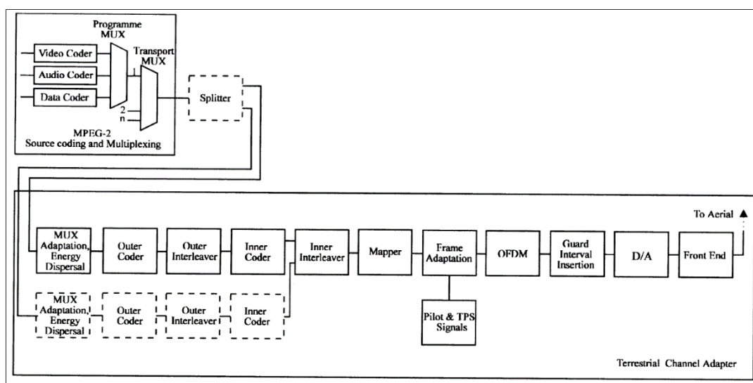
3.4. rasm. DVB-T tizimining uzatuvchi qismining tashkiliy chizmasi
