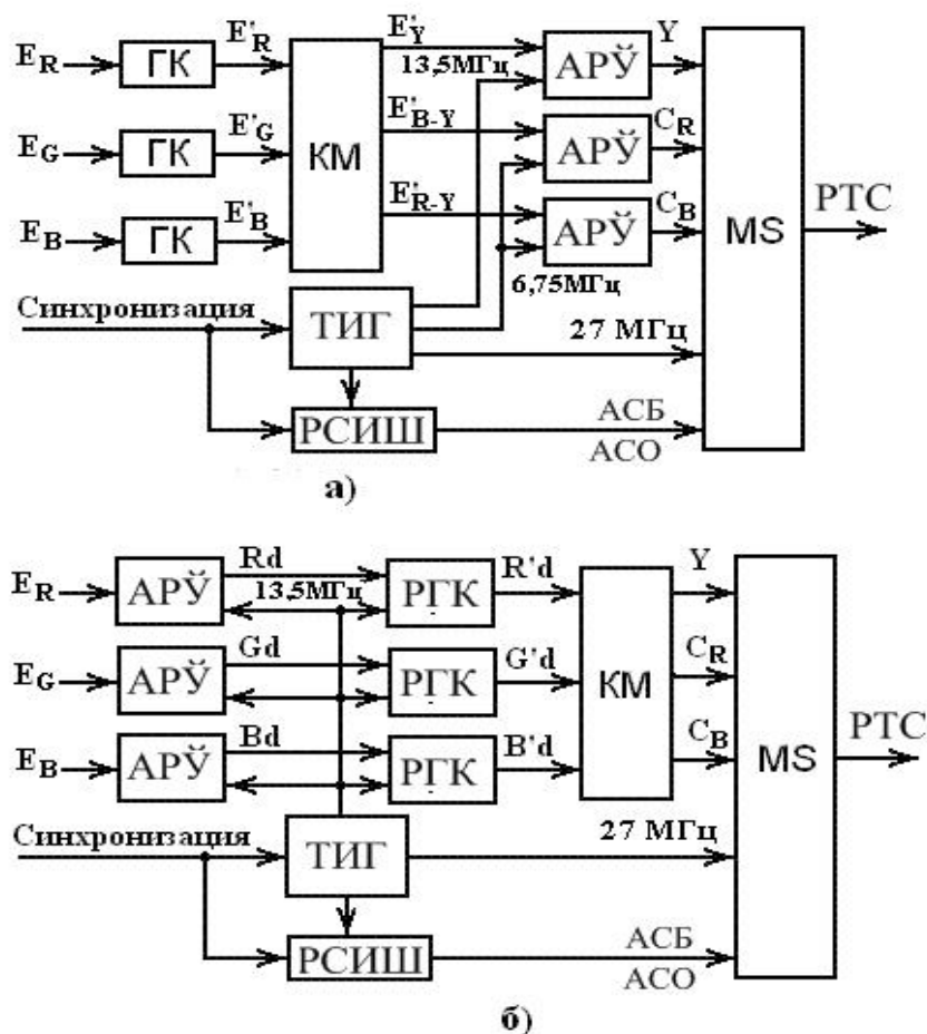
1.11-rasm. Raqamli televizion signalni hosil qiluvchi qurilmaning sxemasi.
