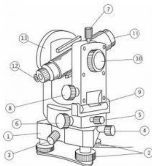
1 rasm. Yuqori aniq optik-elektron taxeovetrning umumiy konstruksiyasi va asosiy qismlari:
