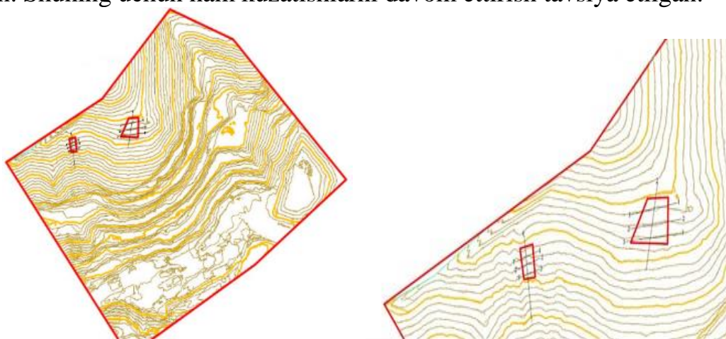
10-rasm. 2- sikl kuzatishlar natijasida tog' jinslarining to'kilib tushish uchatkalari ko'rinishi
