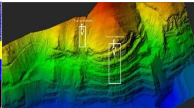
9-rasm. Razrezi uchastkasi (siljishi va deformatsiyalar ko'rsatilgan holda)
