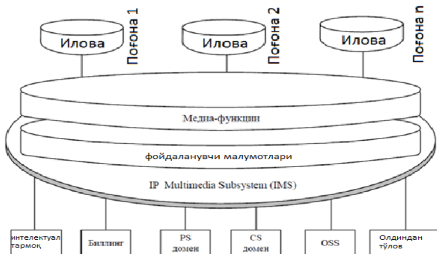
3.4 rasm. IMS da foydalanilayotgan gorizontalar xizmatlar arxitekturasi
