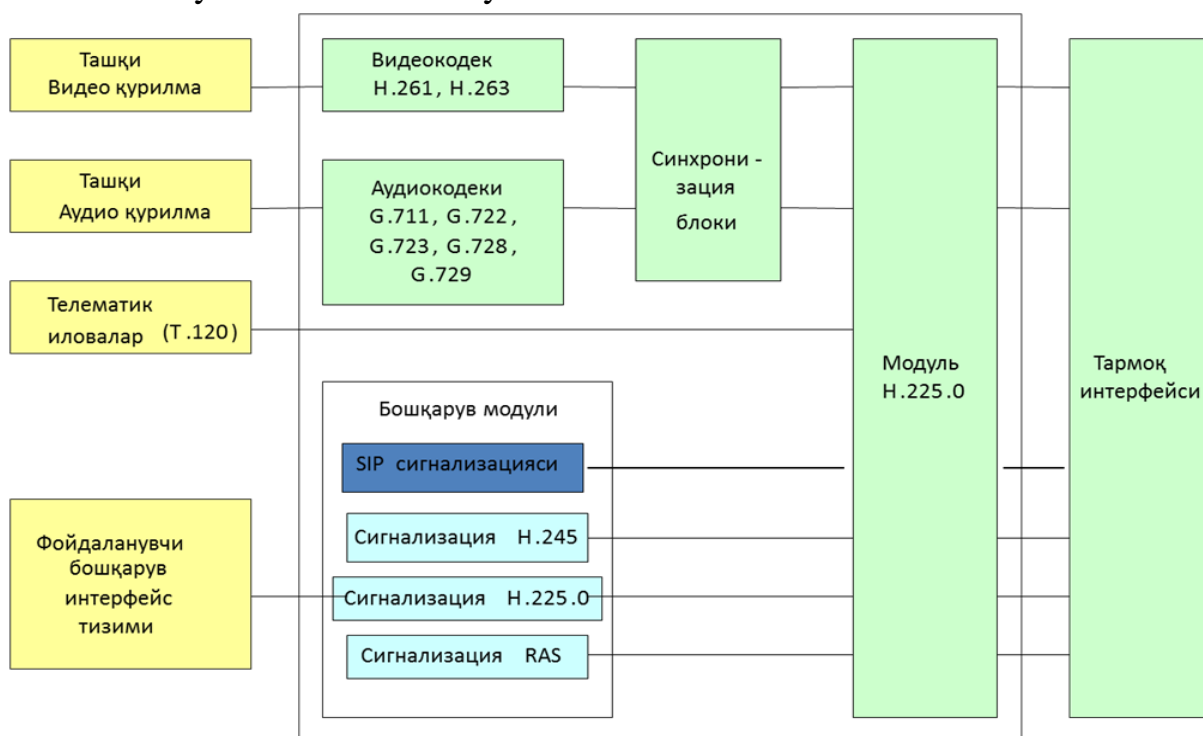
1.5-rasm. SIP, N.323 terminali.
