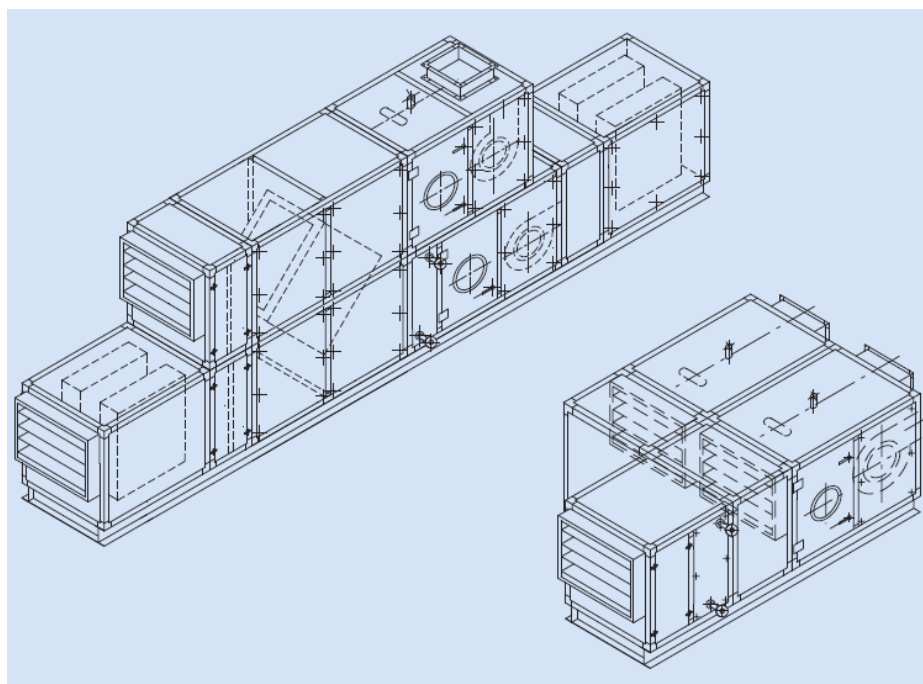
3.9-rasm. KSKP konditsionerining kompanovkasi
