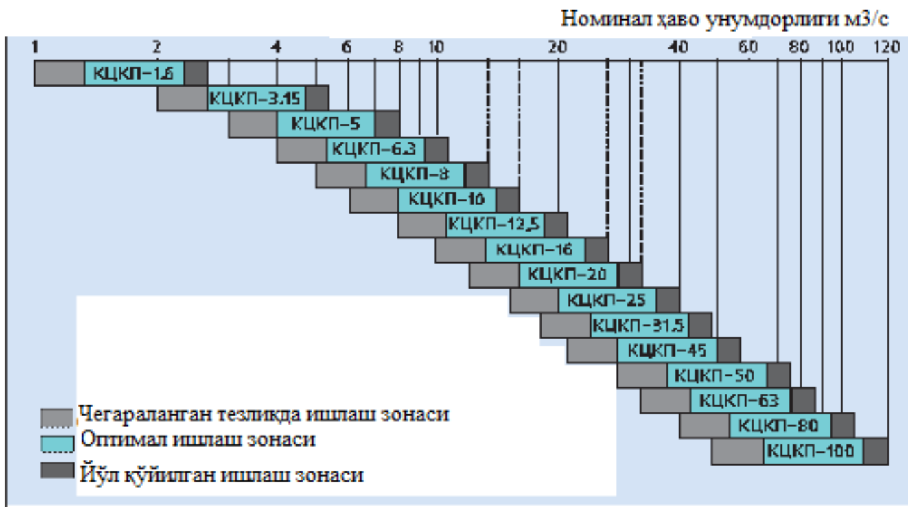
3.7-rasm. Kompakt panelli konditsionerlar “Airmate”
