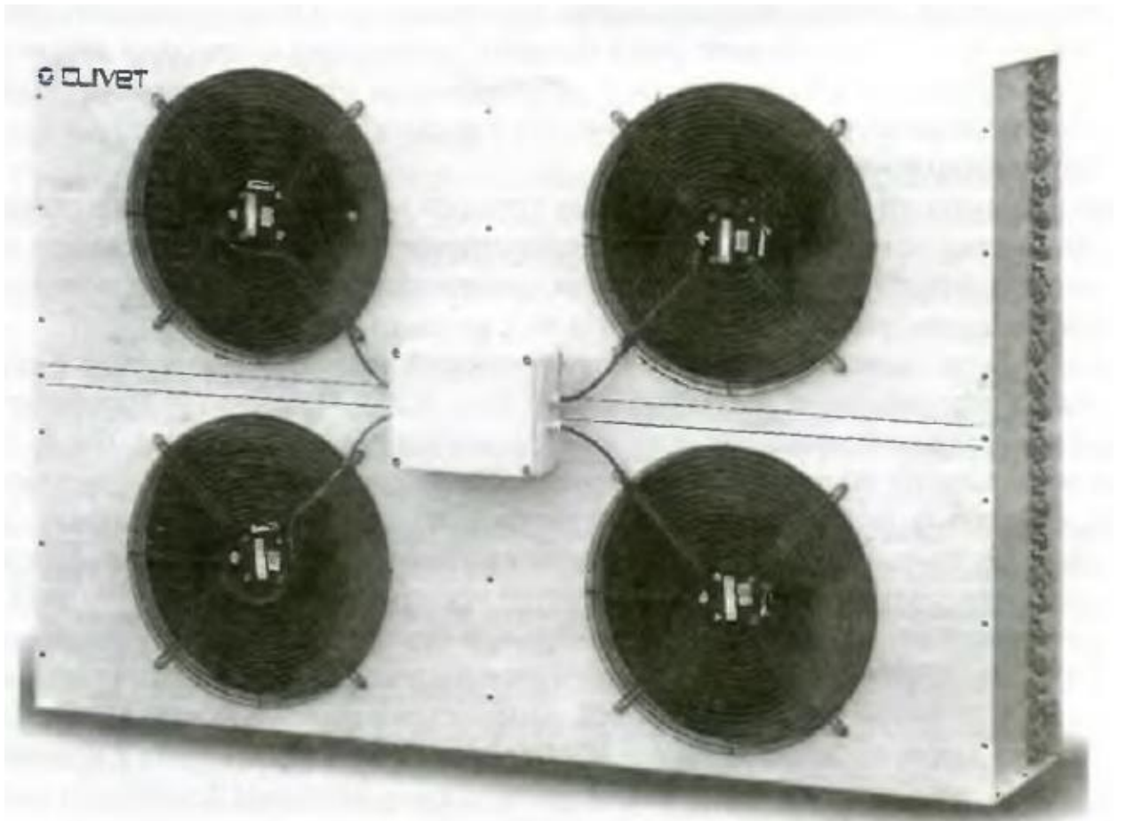
5.1 rasm: Chiller qurilmasi
