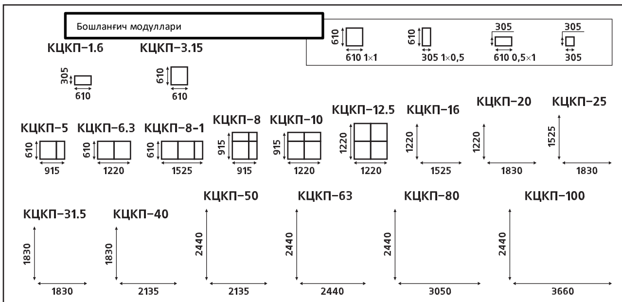
3.4-rasm. Tashqarida va gigienik ishlab chiqariladigan konditsionerlar havo unumdorligining chegaraviy doirasi.
