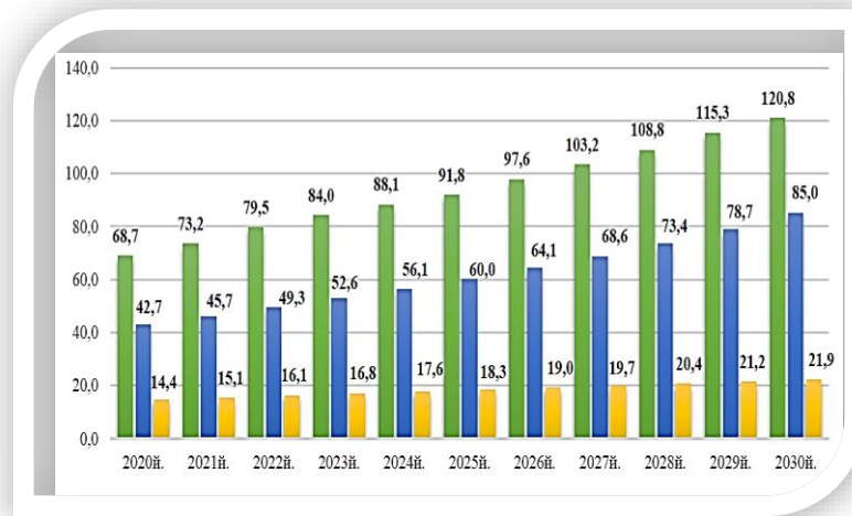
4.1-rasm. 2030 yilgacha elektr energiyasi ishlab chiqarish va iste'mol qilishning prognoz dinamikasi, mlrd.kVt.ch.
