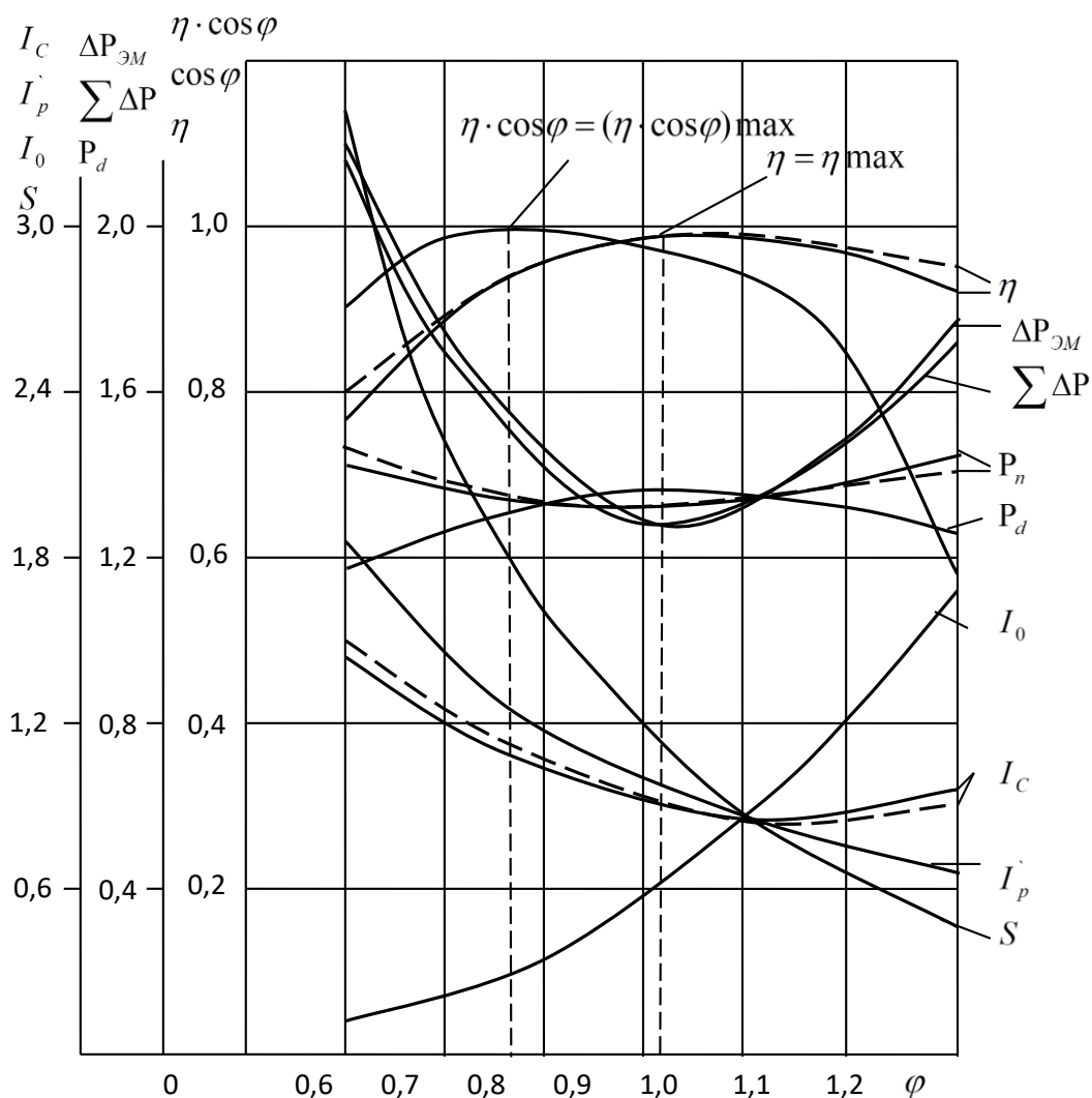
16.4– rasm. Tezligi chastotani o'zgartirib rostlanadigan elektr yuritmalardagi 4A rusumidagi asinxron motorning chastota qiymati f = 1
