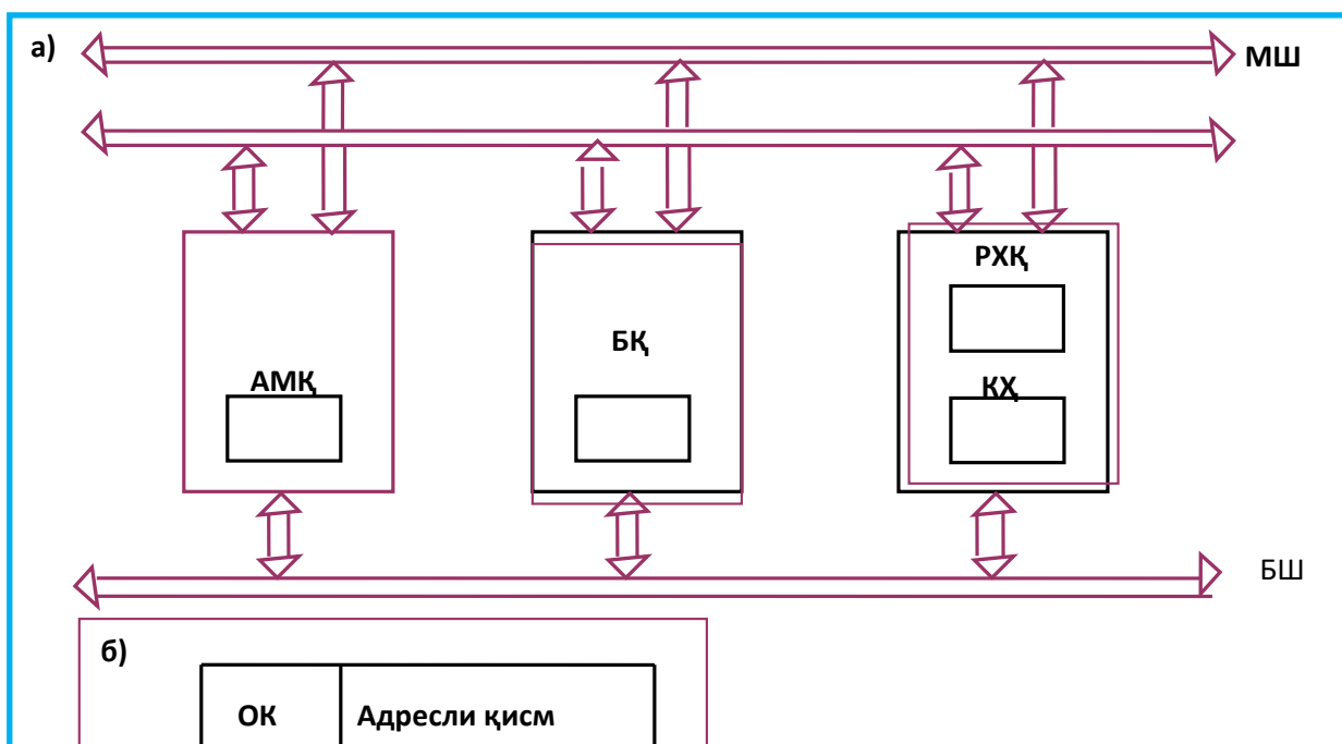
14.3 – rasm. Mikroprotessorning sxemasi (a) va komandalar tarkibi (b)
