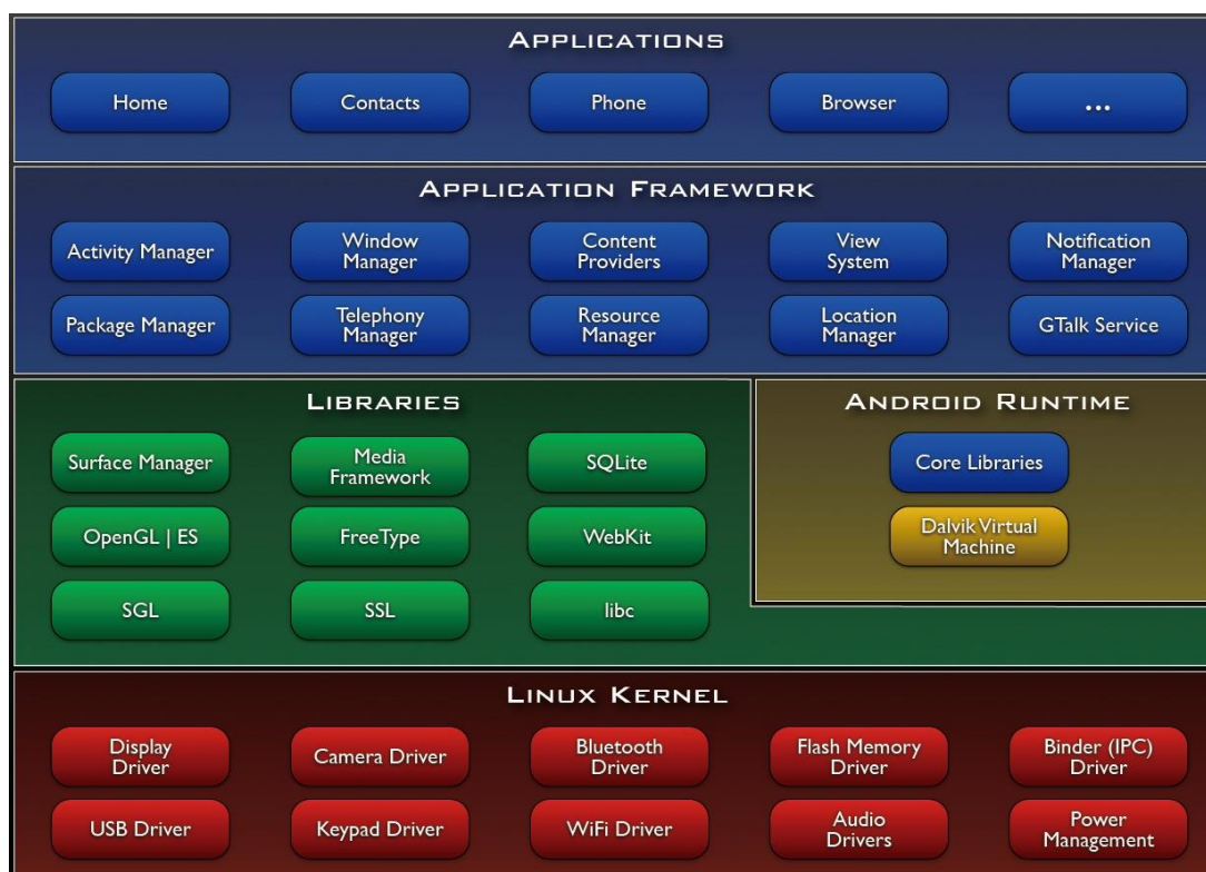
1.2-rasm. Android OT arxitekturasi
