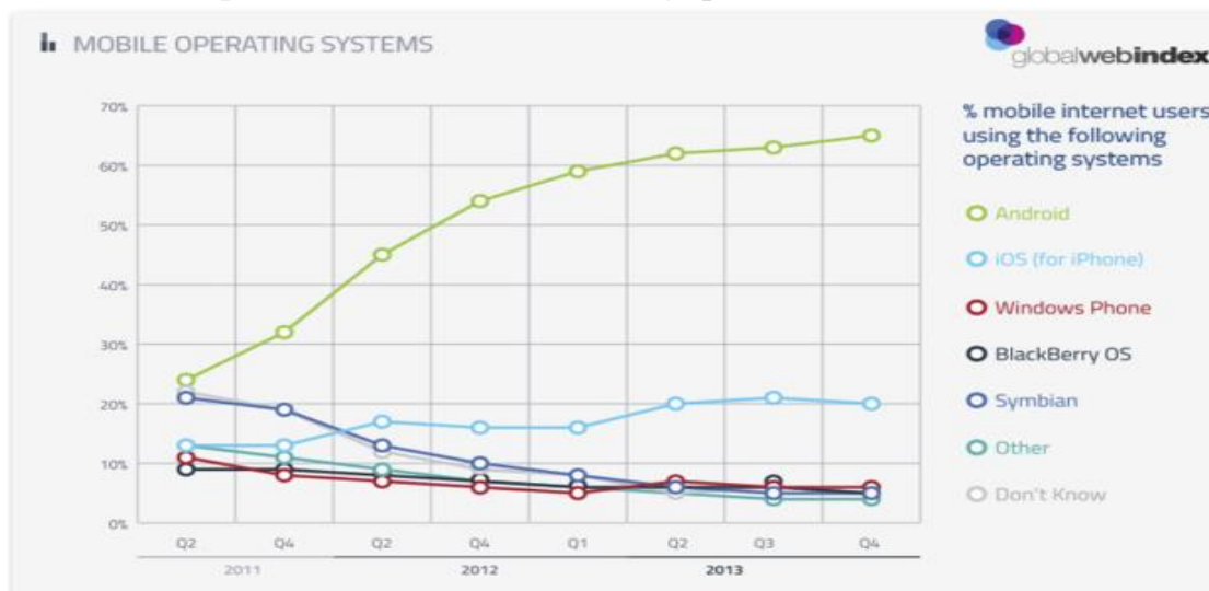
1.1-rasm. Mobil qurilmalar uchun OT larning qo‘llanilish ko‘rsatkichlari
