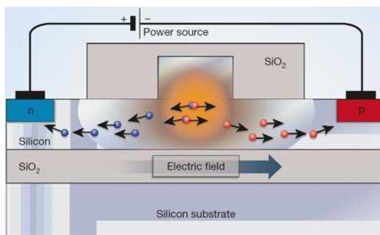
Rasm. 7. Uzluksiz to'liqinli kremniy lazerining PIN-kod tuzilishi
