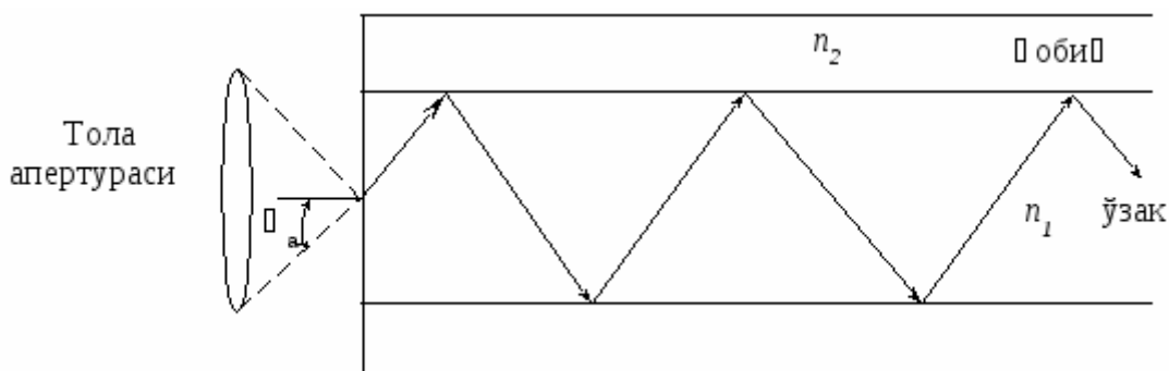
-rasm. Optik tolada yorug'lik nurining tarqalishi.
