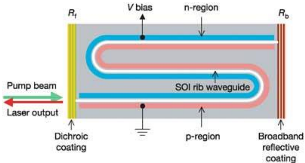
Rasm. 8. Uzluksiz kremniy lazerning sxemasi
