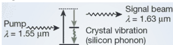
Rasm. 5. Raman effekti tufayli yorug'lik kuchaytirgichining ishlash printsipti
