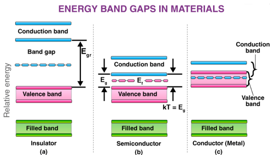
2-rasm. Zonalar nazariyasi, (a) dielektrik, (b) yarimo`tkazgichlar va (c)metall.
