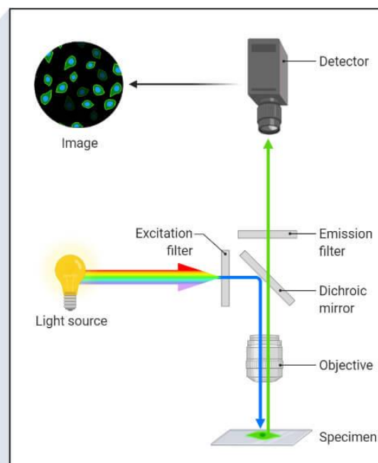
11-rasm. Floresan mikroskopiya
