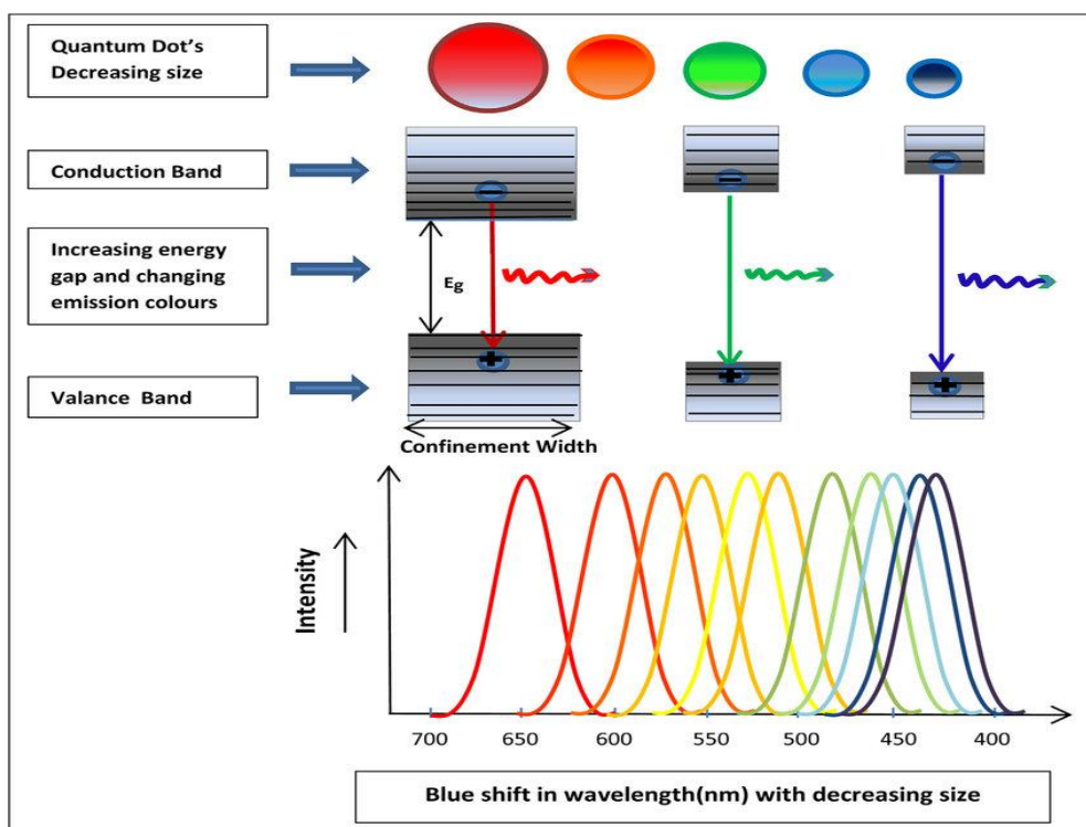
4-rasm. Nanostrukturalarning kvant o'lcham effektlari.
