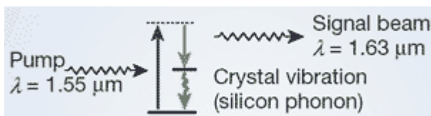
Rasm. 5. Raman effekti tufayli yorug'lik kuchaytirgichining ishlash printsipti
