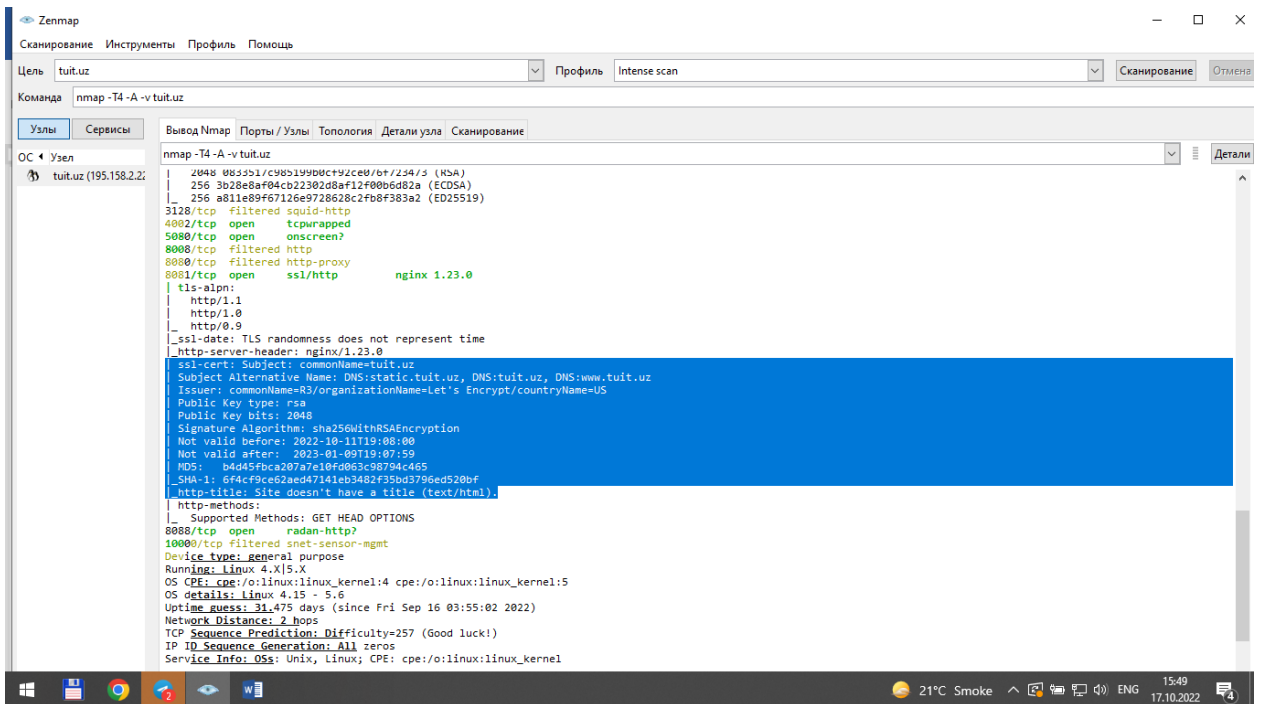
5.9-rasm. SSL sertifikatini haqida ma'lumot
