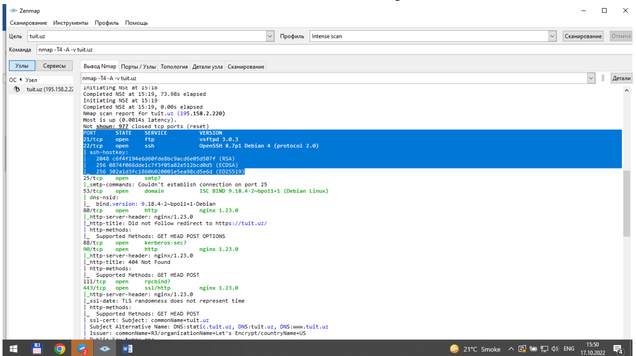
5.10-rasm. ftp va ssh haqida ma'lumot
