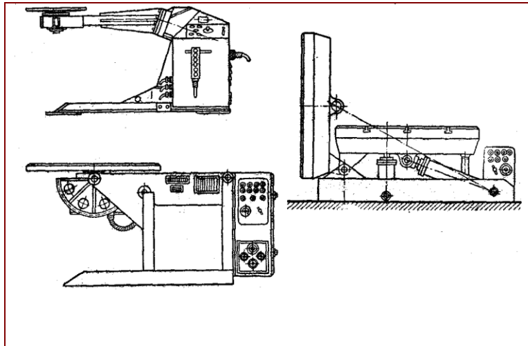
4.9-rasm. Manipulyatorlar.
