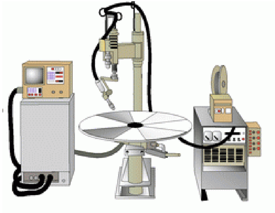
4.11-rasm. To'g'ri chiziqli va halqasimon choklarni payvandlash uchun kolonna 42
